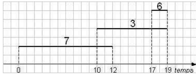
FIG. 8.7: Structure d'intervalles du problème sur M_3 - Étape 1
