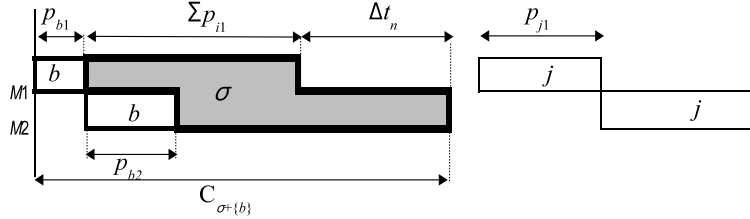
FIG. 7.2: Séquences optimales pour le cas mono-pyramidal ( P_b appartient à I_1 )
