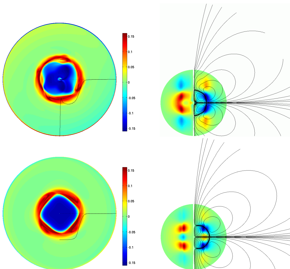
FIG. 6.12 – Vorticit  (  gauche), et champ magn tique (  droite) pour la dynamo quadrupolaire satur e Q6_h ( E = 10^{-6} , Ro = -0.08 , Pm = 0.1 ) qui s'inverse. La ligne du haut pr sente l' tat pour le maximum du champ magn tique, et la ligne du bas pour le minimum (voir fig. 6.10).
