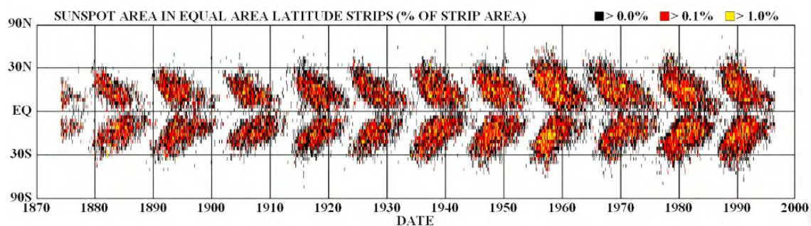
FIG. 1.8 – Position des taches solaires de 1870 à 1995. La ligne centrale horizontale représente l'équateur du Soleil. On remarque que les taches solaires apparaissent au nord et au sud, puis migrent vers l'équateur. C'est le diagramme "papillon" qui montre bien le cycle à 11 ans. (NASA)
