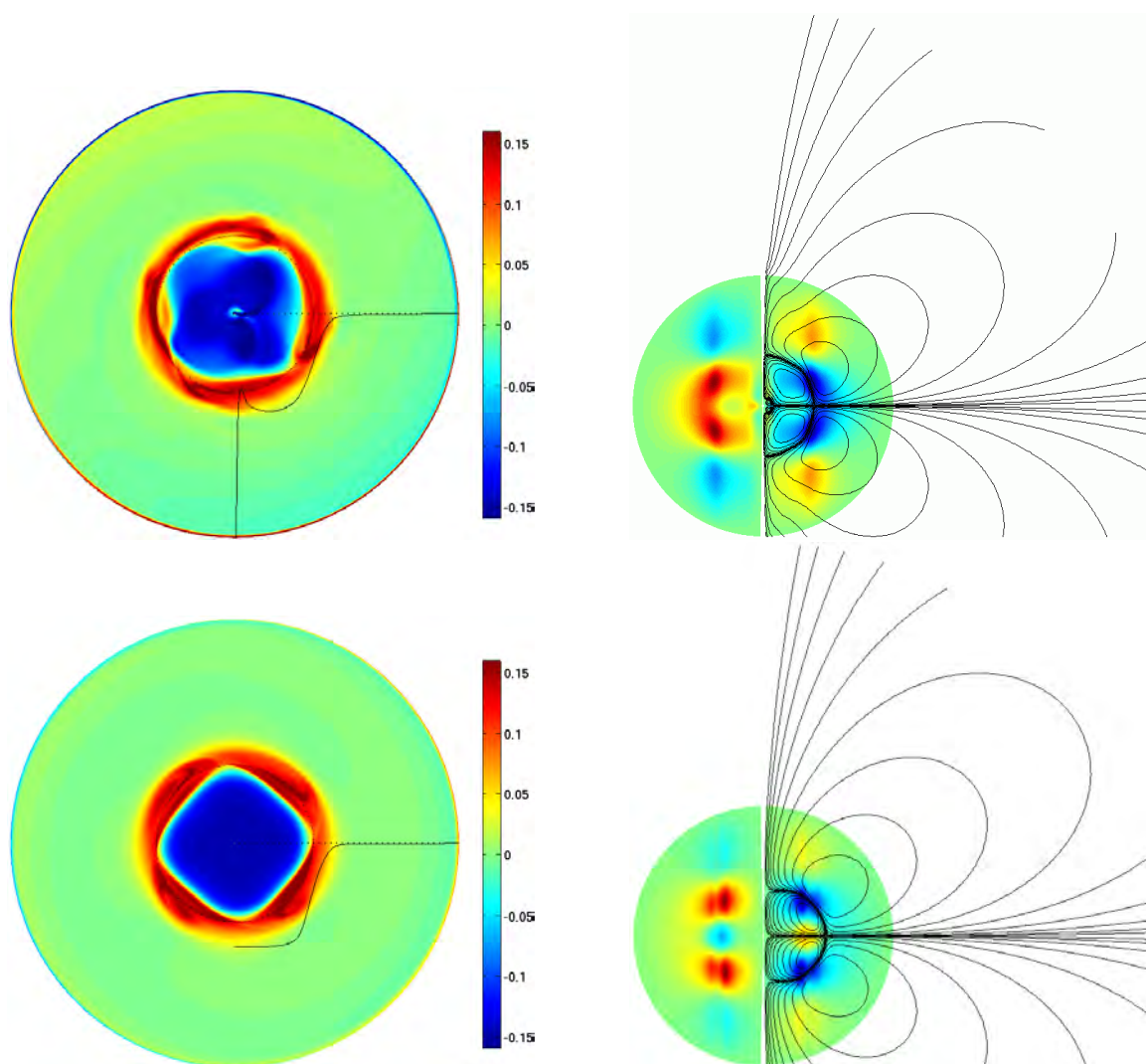
FIG. 6.12 – Vorticité (à gauche), et champ magnétique (à droite) pour la dynamo quadrupolaire saturée Q6_h ( E = 10^{-6} , Ro = -0.08 , Pm = 0.1 ) qui s'inverse. La ligne du haut présente l'état pour le maximum du champ magnétique, et la ligne du bas pour le minimum (voir fig. 6.10).
