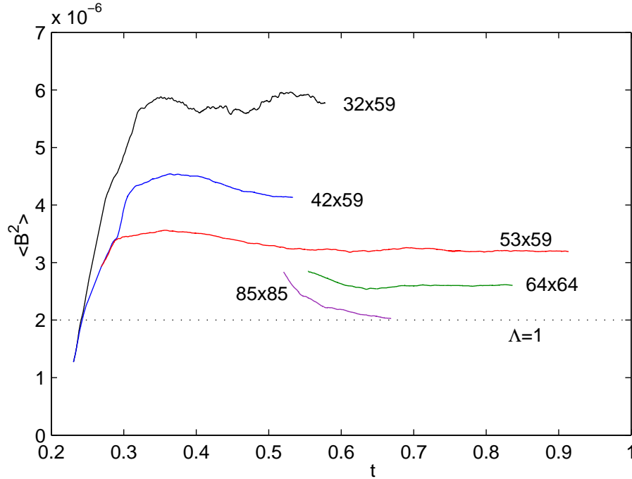
FIG. 6.7 – Évolution de l'énergie magnétique en fonction du temps pour les modèles Q8_{xx} . Les courbes sont marquées par m_{\max}^B \times l_{\max} . \Lambda = 1 correspond donc à \langle B^2 \rangle = 2 \cdot 10^{-6} .
