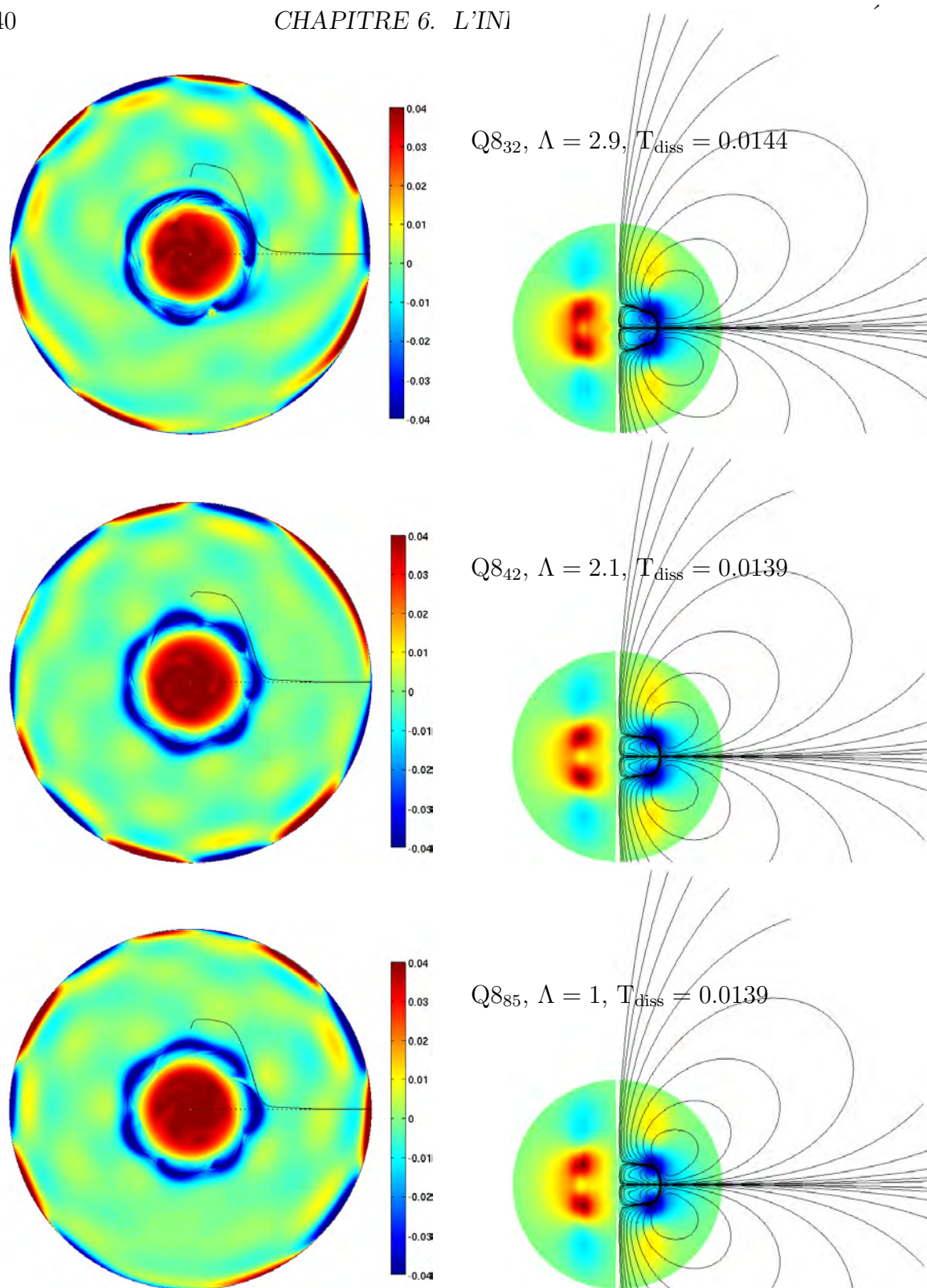
FIG. 6.8 – Effet de la troncature sur les dynamos saturées. Champ de vorticité totale et vitesse angulaire zonale (à gauche), et champ magnétique (à droite) pour des dynamos saturées Q8_{xx} (avec E = 10^{-8} , Ro = 0.02 , Pm = 0.005 ).
