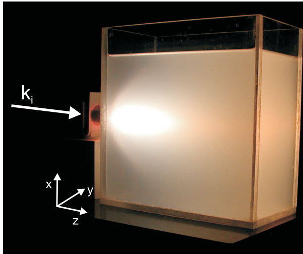
Figure 2.5: Light diffusion in a turbid liquid (courtesy of Francesco lo Bue, http://olympus.umh.ac.be/ ).
