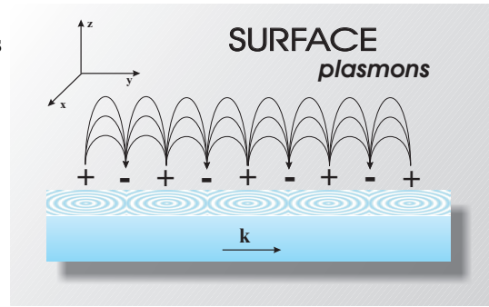
Fig. 4 : Une vision d'artiste des plasmons de surface à l'interface vide/métal.
