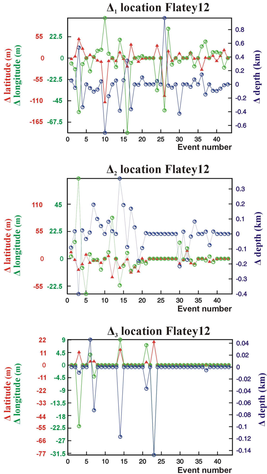
Figure II-43: Changements de position pour chaque séisme de l'essai Flatey12 entre deux processus successifs de relocalisation.
