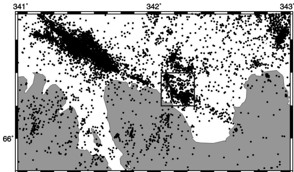
Figure II-41: Zone d'étude pour la relocalisation d'essaims de séismes.
