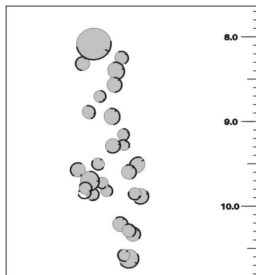
Figure II-51: Analyse des mécanismes au foyer de l'essaim Flatey12. Représentation suivant un angle de vue perpendiculaire au plan de faille de chacun des plans nodaux de l'essaim. Les mécanismes coloriés en gris sont ceux retenus pour définir le mouvement sur le plan de faille général. Même modes de représentation qu'à la Figure II-47.
