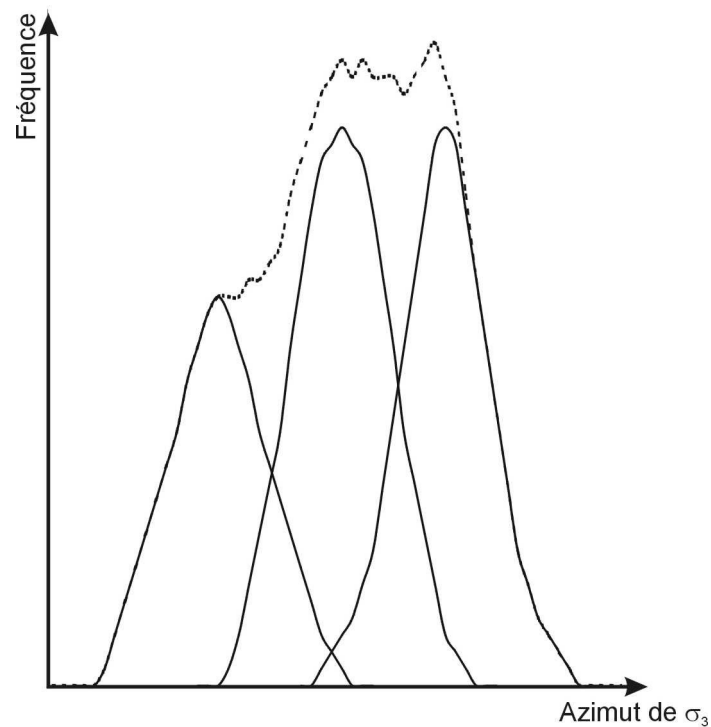
Figure II-16: Problème du chevauchement des azimuts. Cas de trois phases tectoniques distinctes (traits continus) dont les directions d'extension (par exemple) se chevauchent partiellement. Le signal apparent (trait discontinu) est alors fortement influencé par le recouvrement azimutal.
