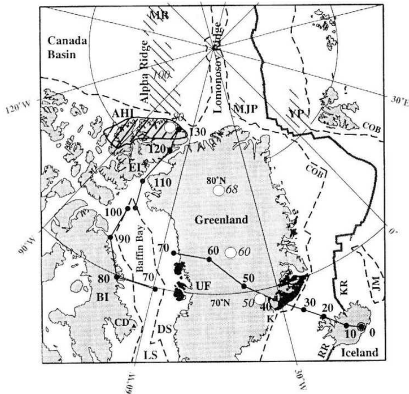
Figure I-4: Trajectoire de la dérive du point chaud islandais déterminé par Lawver et Müller (1994).
