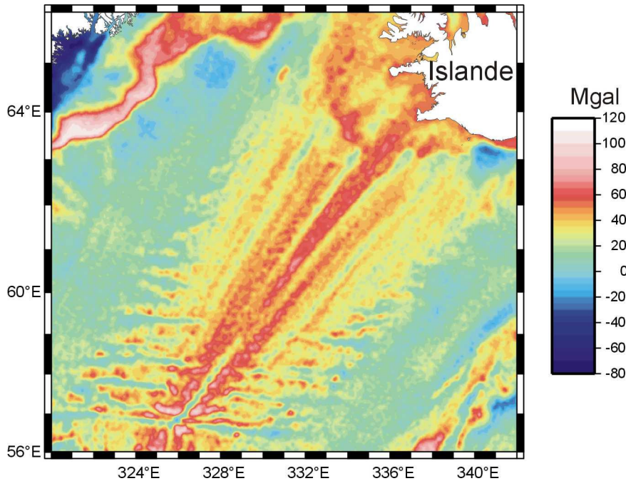
Figure I-9: Carte d'anomalies gravimétriques le long de la dorsale de Reykjanes. D'après les données de Sandwell et Smith (1997).
