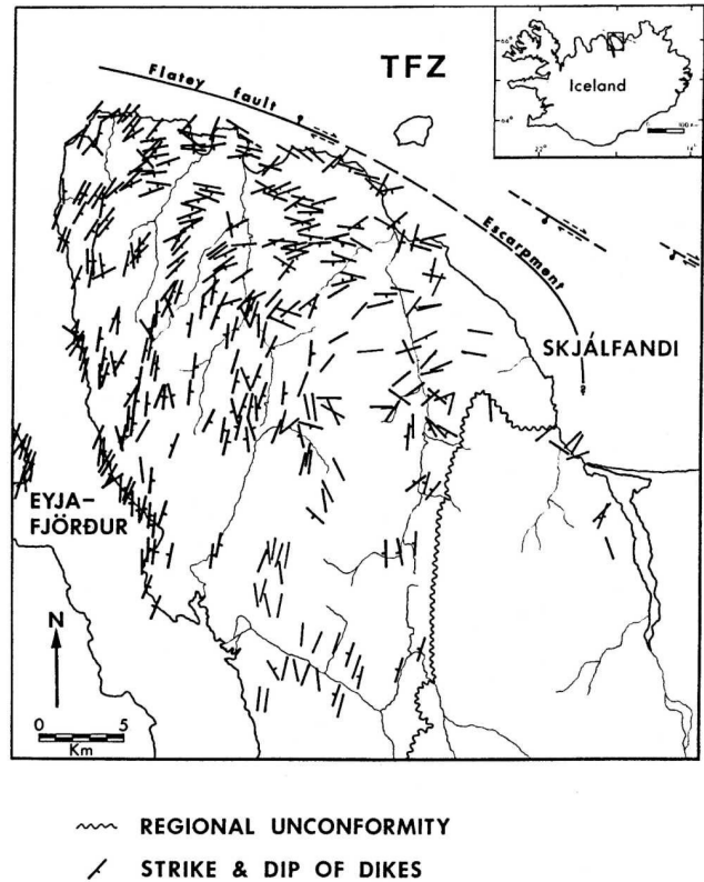
Figure II-3: Orientations des dykes dans la péninsule de Flateyjarskagi (Young et al., 1985).
