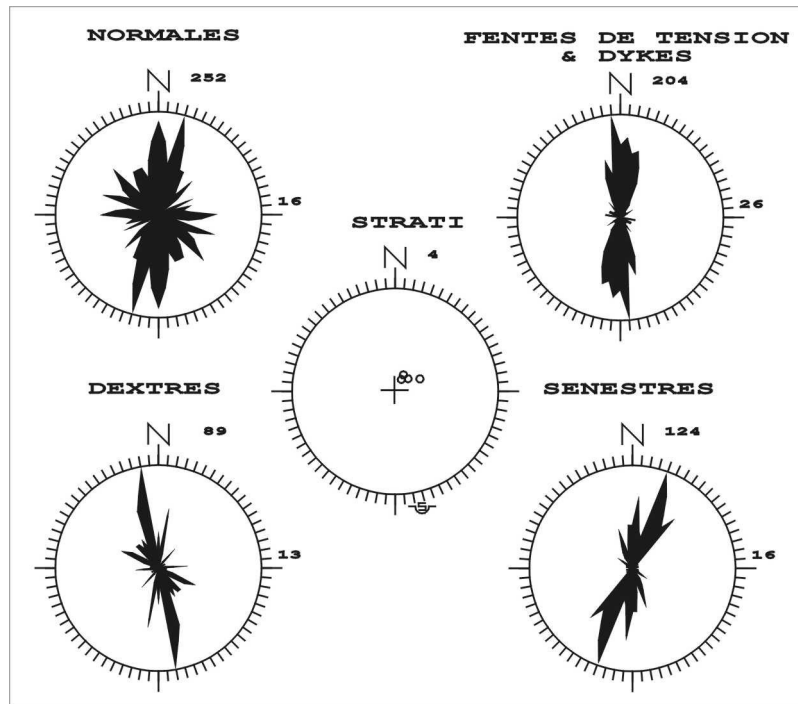
Figure II-26: Rosaces de distribution azimutale des structures cassantes distantes de la zone de connexion.
