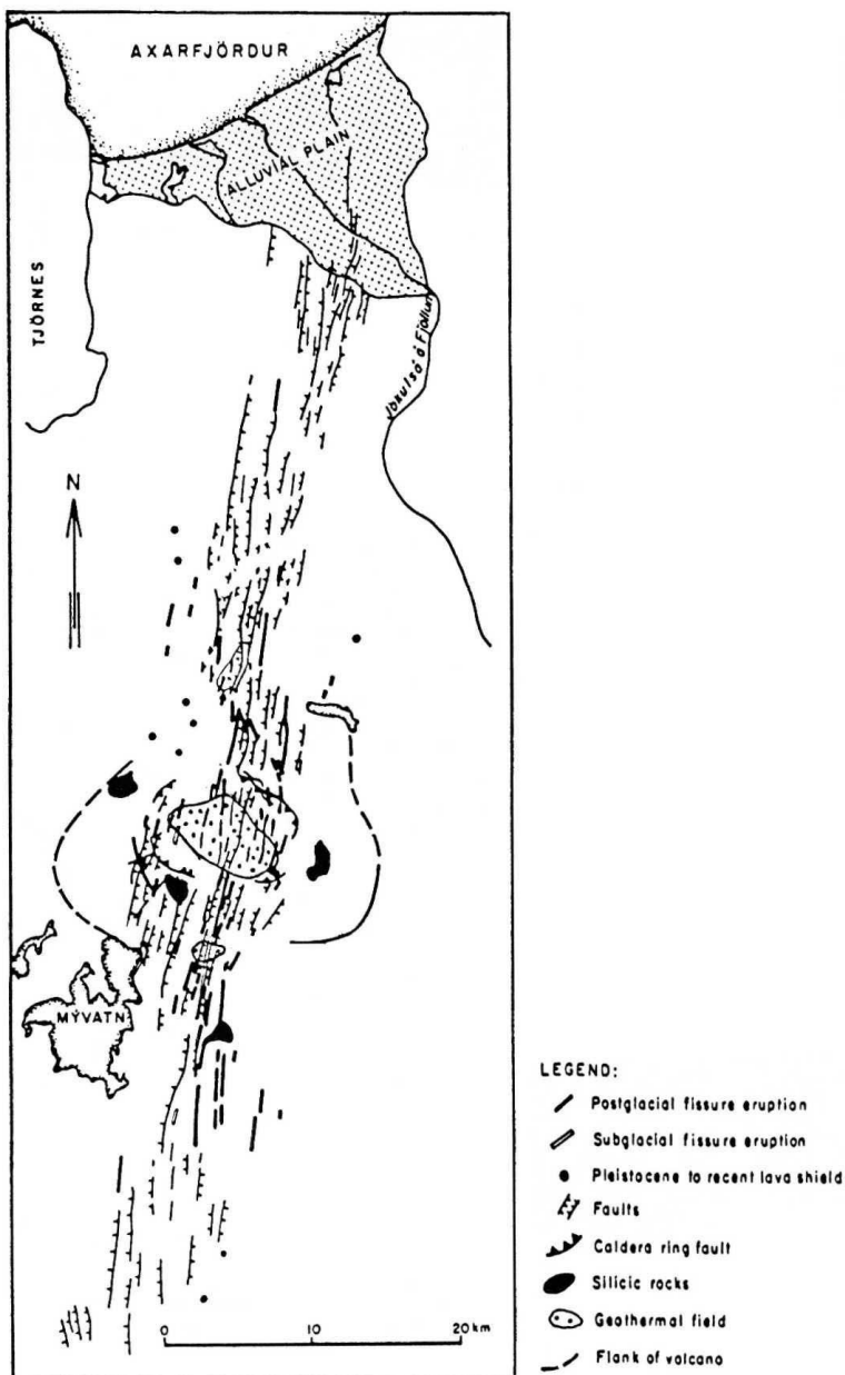
Figure I-14: Disposition schématique des différents éléments d'un faisceau de fractures (Forslund et Gudmundsson, 1991).
