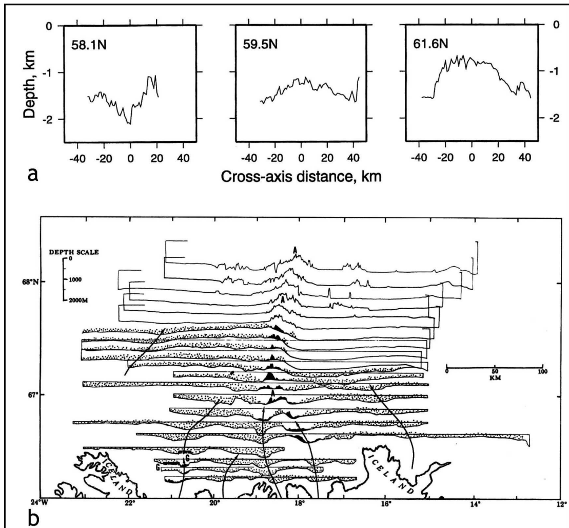
Figure I-8: Profils bathymétriques à travers la dorsale médio-Atlantique à proximité de l'Islande. a: Ride de Reykjanes (Searle et al., 1998). b: Ride de Kolbeinsey (Vogt et al., 1980). En (b), les affleurements basaltiques sont indiqués en noir et les régions recouvertes de sédiments glaciaires sont indiquées par des pointillés.
