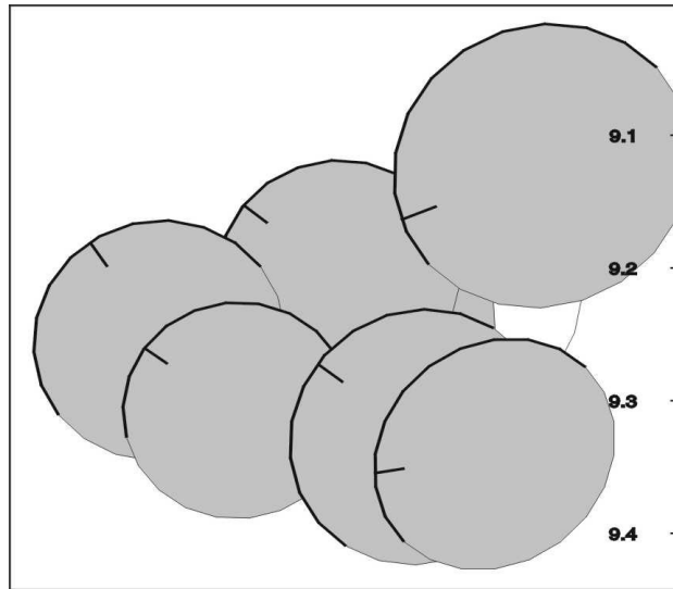
Figure II-53: Analyse des mécanismes au foyer de l'essai Flatey18. Représentation suivant un angle de vue perpendiculaire au plan de faille de chacun des plans nodaux de l'essai. Les mécanismes coloriés en gris sont ceux retenus pour définir le mouvement sur le plan de faille général. Même modes de représentation qu'à la Figure II-47.
