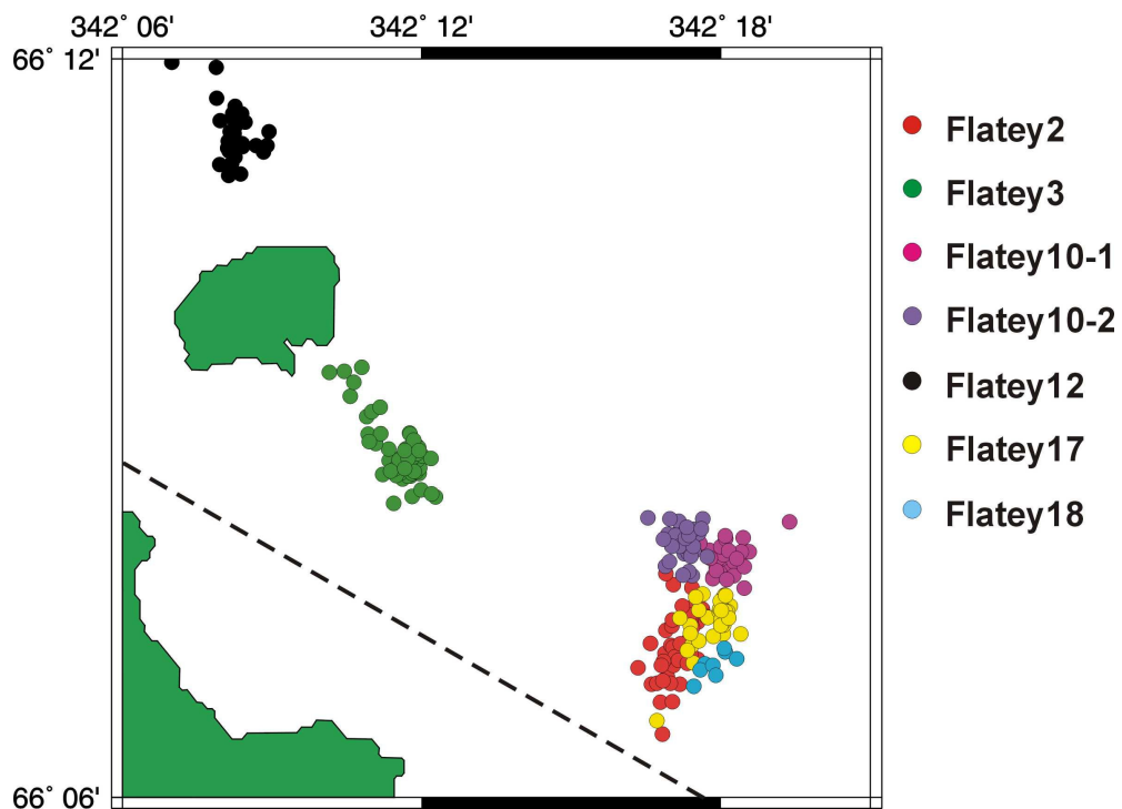
Figure II-42: Localisation des séismes de chaque essaim avant relocalisation.
