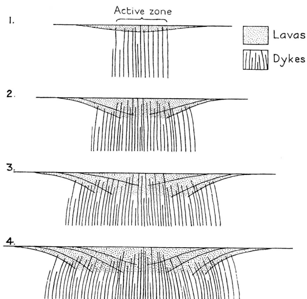
Figure I-19: Modèle d'accrétion de Bodvarsson et Walker (1964).
