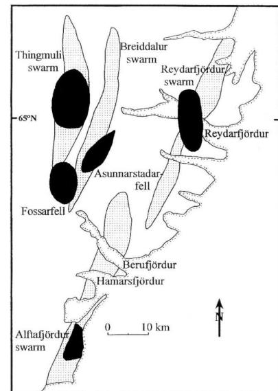
Figure I-15: Faisceau de dykes et complexes filoniens annulaires dégagés par l'érosion dans l'Est de l'Islande (Gudmundsson, 1998). Les faisceaux de dykes sont en gris clair et les complexes filoniens en noir.
