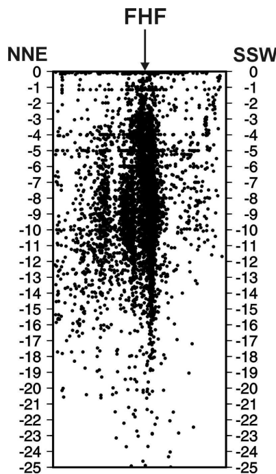
Figure II-20: Sismicité de la FHF le long d'une coupe NNE-SSW. L'ensemble des données sismiques de la zone indiquée sur la Figure II-18 est projeté sur une coupe de direction N025°E, perpendiculaire à la direction moyenne de la FHF. La position de la FHF est indiquée sur la coupe. Les profondeurs sont données en kilomètres. Les séismes considérés vont du 28/08/1993 au 01/09/2002.
