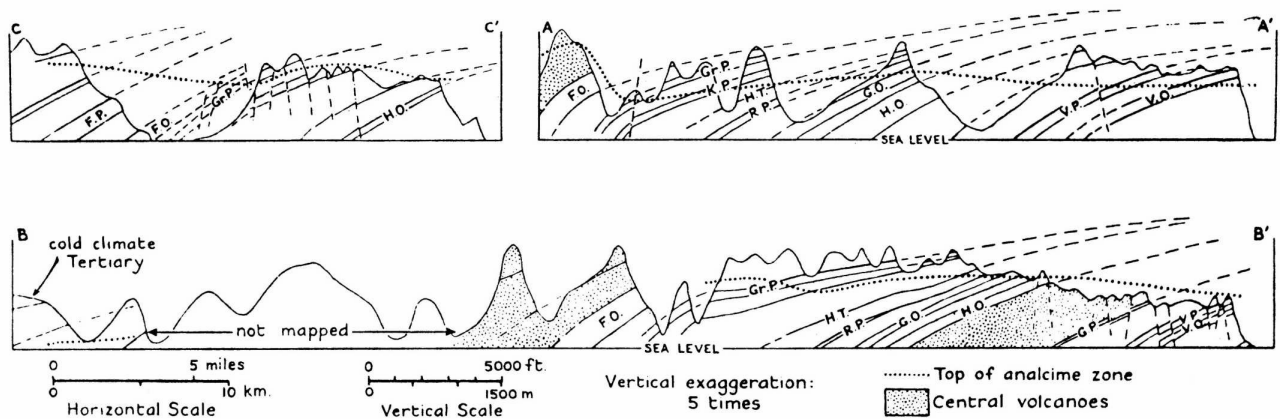
Figure I-18: Coupe schématique E-W à travers les séries tertiaires dans l'Est de l'Islande (Walker, 1960).
