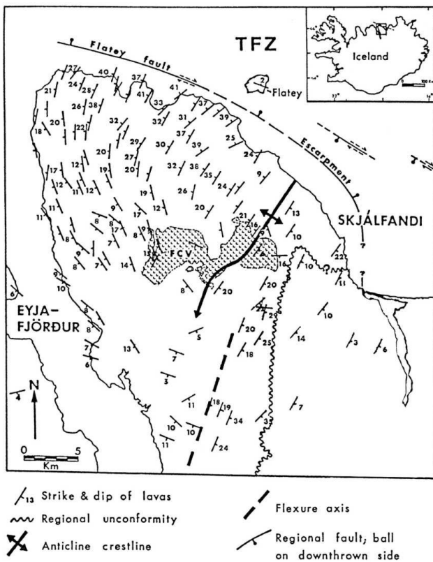
Figure II-2: Pendage des laves dans la péninsule de Flateyjarskagi (Young et al., 1985). FCV: Flateyjardalur Central Volcano.
