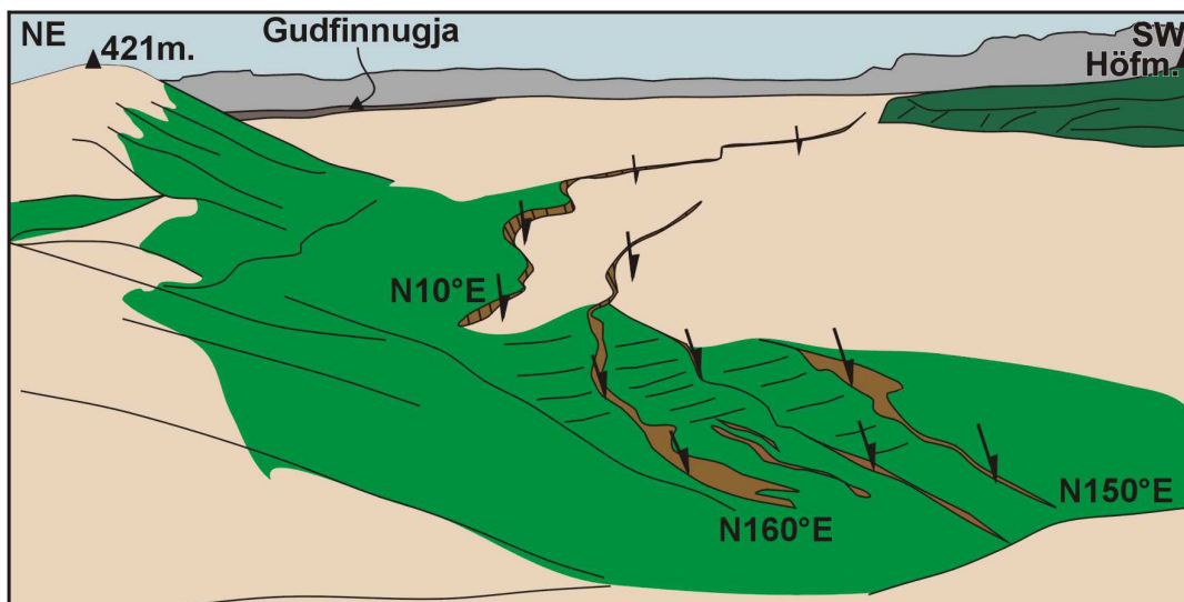
Figure II-38: Failles normales disposées en échelon et relayant le mouvement décrochant de la Faille Septentrionale.
