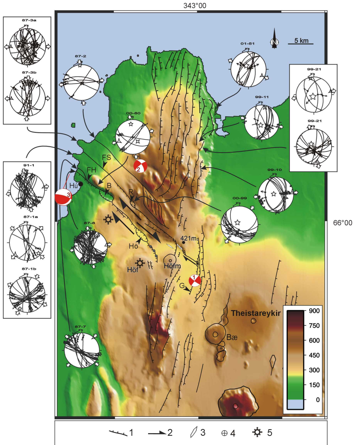
Figure II-39: Synthèse de l'analyse structurale de la péninsule de Tjörnes.
