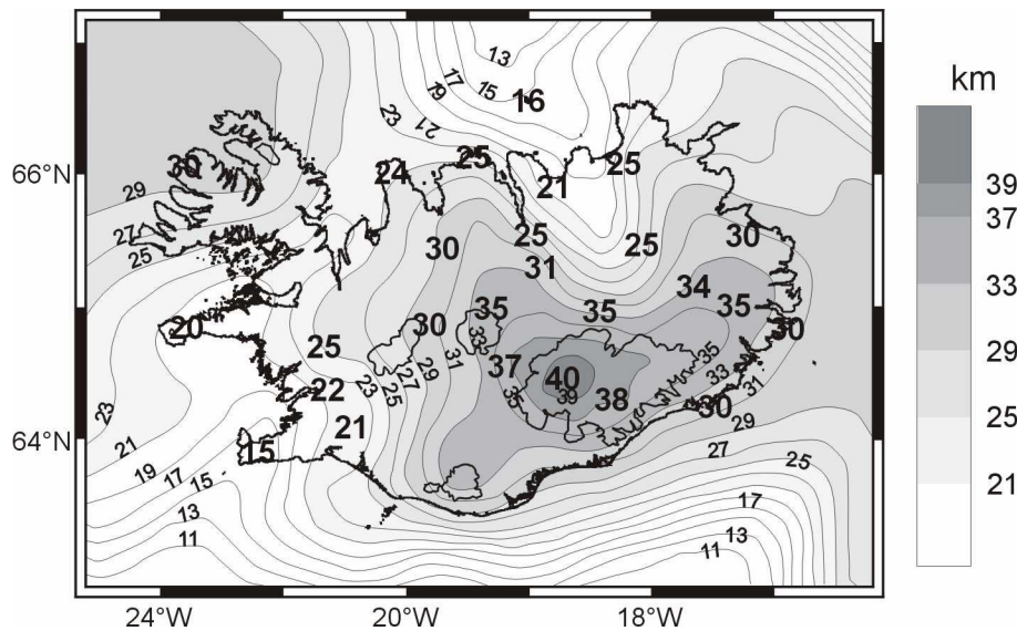
Figure I-5: Epaisseur crustale en Islande (modifié d'après Kaban et al., 2002). Mesures crustales ponctuelles par méthode sismique de Bjarnason et al. (1993), Menke et al., (1996, 1998), Staples et al. (1997), Darbyshire et al. (1998, 2000a, 2000b), Du et Foulger (2001) et Du et al. (2002).
