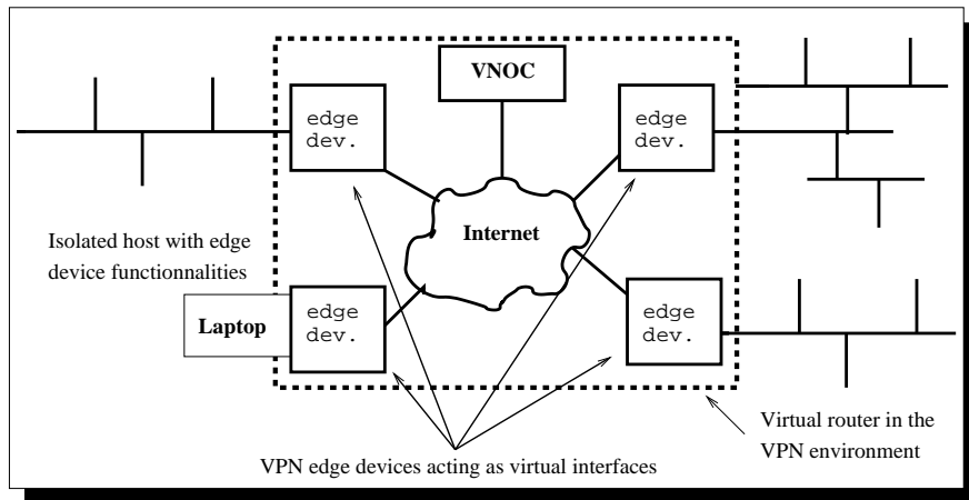
Figure 12.1. Le concept du routeur virtuel.
