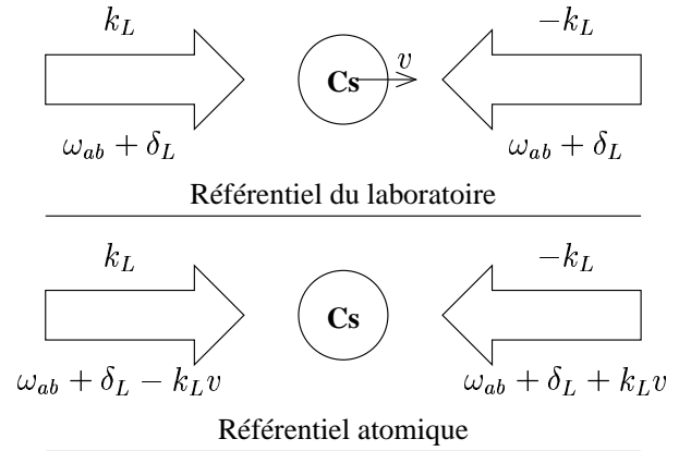
FIG. 2: Effet Doppler
