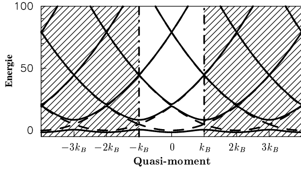
FIG. 41: Repli des bandes d'énergie dans la zone de Brillouin
