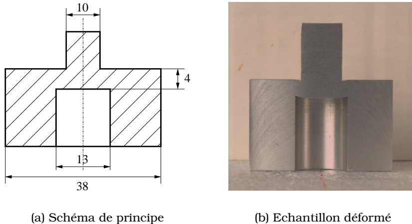
FIG. 2.9 – Essai de cisaillement dynamique
