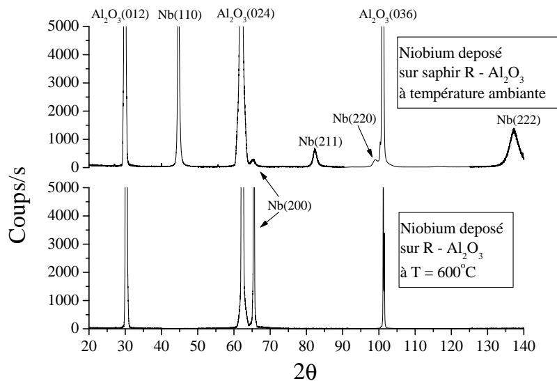
FIG. 4.1: Comparaison des graphes de diffraction \theta - 2\theta de deux films de Nb dont la croissance sur substrat saphir (d'orientation [1\bar{1}02] ) a été obtenue avec les mêmes paramètres de dépôt optimaux, excepté la température de dépôt : le film du haut a été déposé à température ambiante, celui du bas à 600^\circ\text{C} . Extrait de [Delaët et al. , 2001b].
