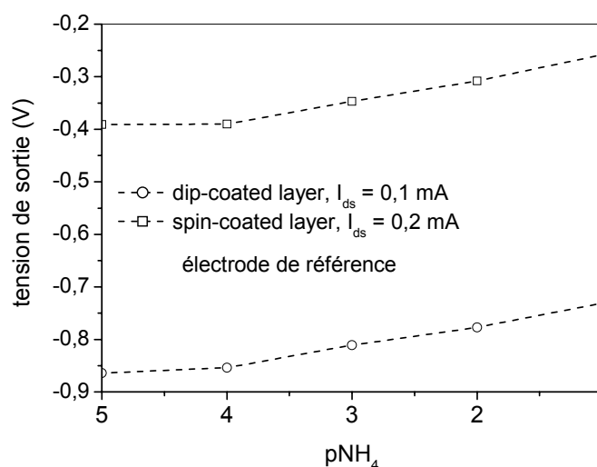
Figure 4.31: Sensibilité des p\text{NH}_4 – ChemFETs avec différentes techniques de dépôt des membranes.
