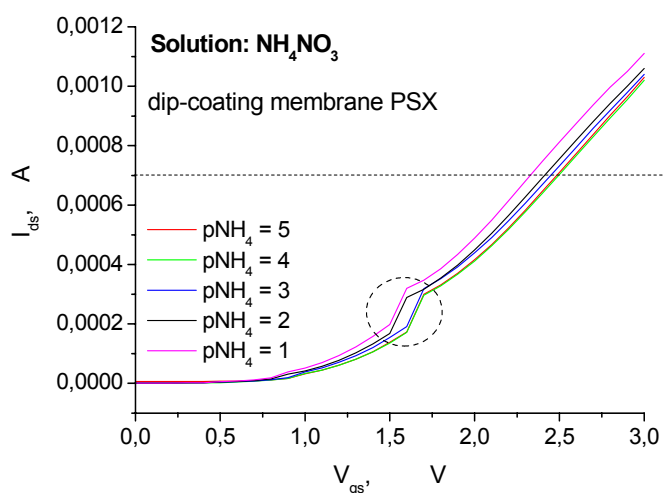
Figure 4.26 Courbes de transfert du capteur \text{pNH}_4 - ChemFET
