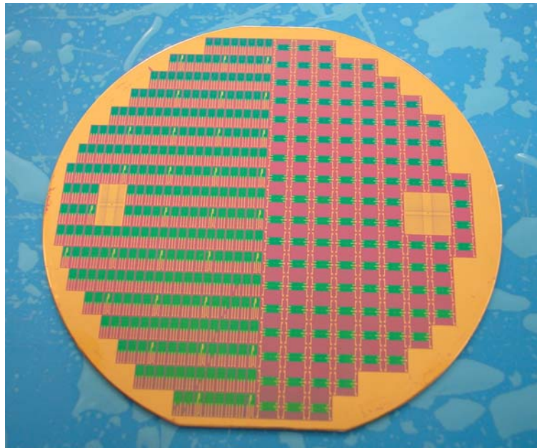
Figure 2.33: Photographie d'une plaquette des FSC-ChemFETs
