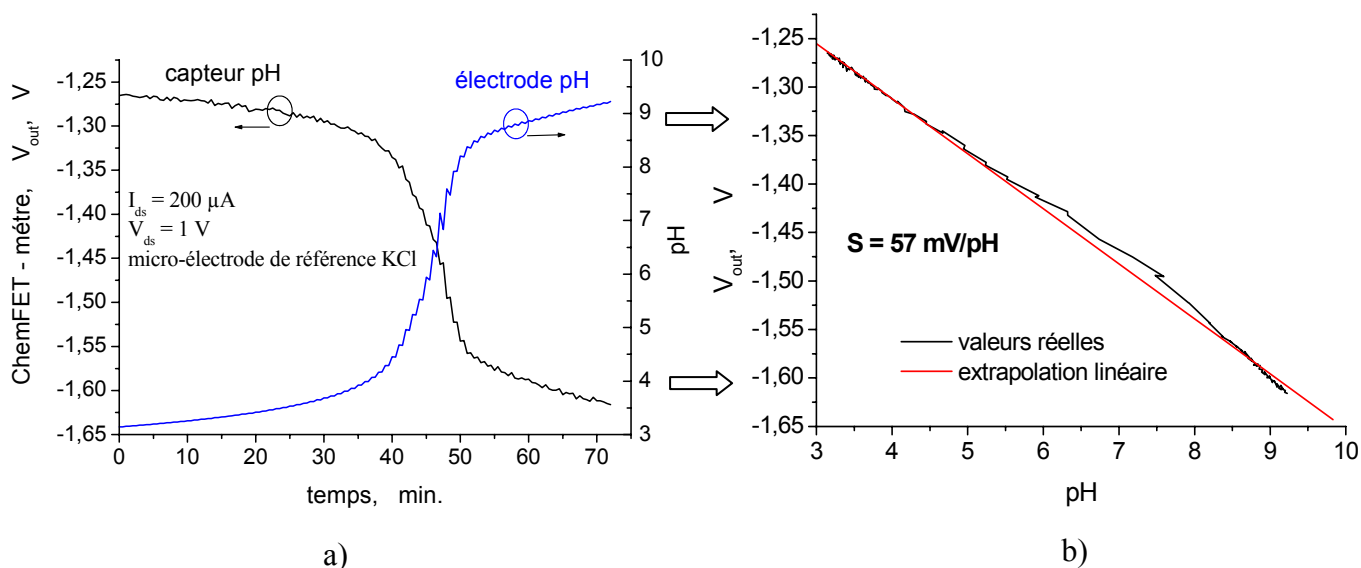
Figure 4.25: Réponse du capteur pH-ChemFET et électrode pH aux variations de la concentration hydrogène en continu (a) et la courbe de sensibilité (b)
