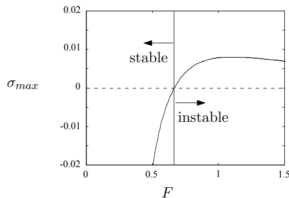
FIG. 7.9 – Billes de verre. Taux de croissance du mode le plus instable \sigma_{max} (adimensionné) en fonction du nombre de Froude ( \theta = 29^\circ ).
