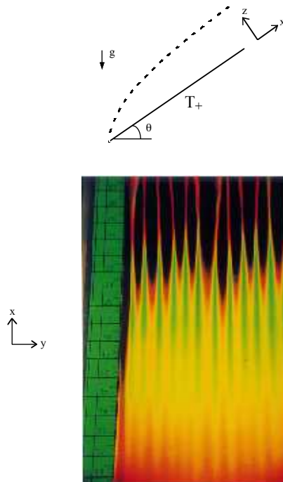
FIG. 1.7 – Rouleaux de convection longitudinaux dans un écoulement de couche limite le long d'une plaque chauffée inclinée (Jeschke &amp; Beer 2001).
