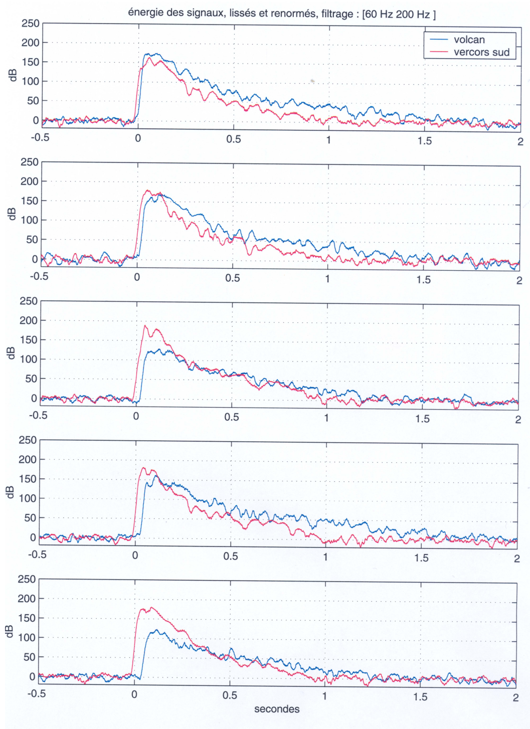
FIG. 3.4 – Comparaison de la coda acquise sur deux sites, dans le sud Vercors urgonien (en rouge) et au pied du Puy des Goules (Auvergne, en bleu). De haut en bas, la distance source-capturs est de 10 m, 15 m, 20 m, 25 m et 30 m.
