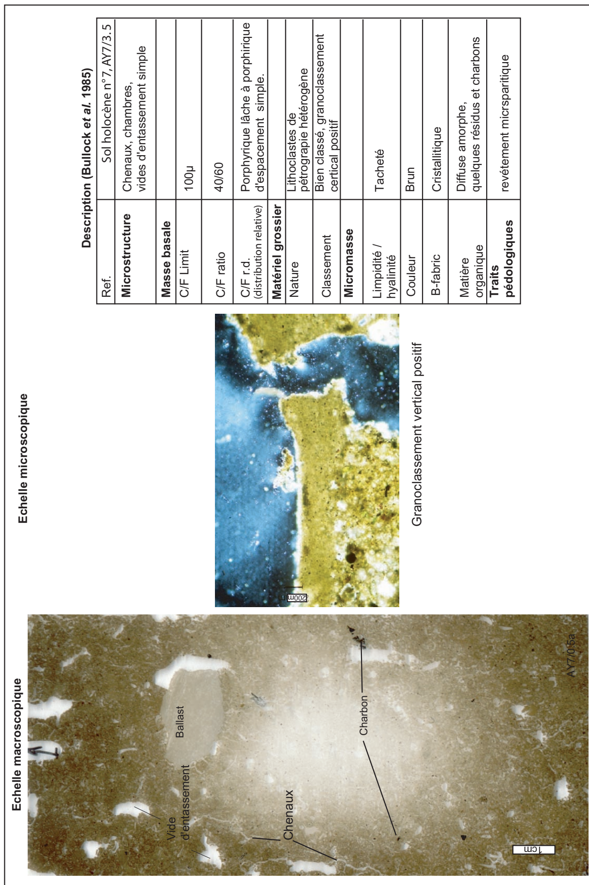
Figure 59 : Observation micromorphologique du paléosol n°7 (AY7/0.5)
