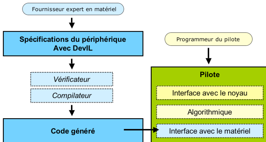
Figure 1-10 Conception d'un pilote avec la méthode DEVIL
