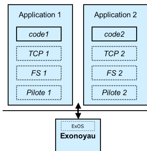
Figure 1-9 Approche Exonoyau selon XOK
