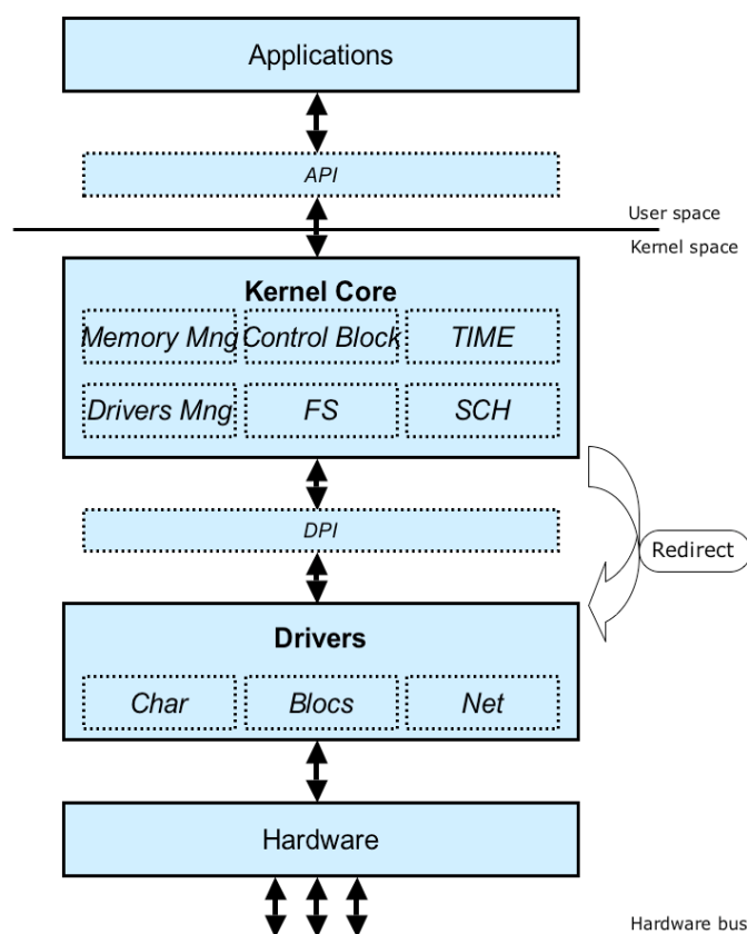
Figure 3-1 Architecture d'un système d'exploitation moderne
