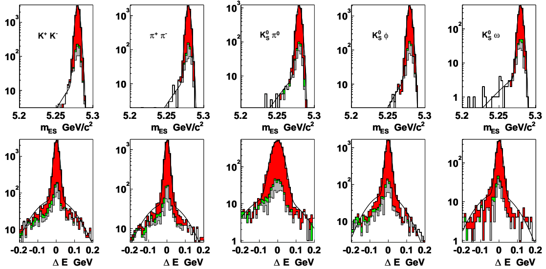
FIG. 7.6 – Les distributions de m_{ES} (en haut) et \Delta E (en bas) pour les évènements de Monte Carlo de signal. Les candidats bien reconstruits sont en rouge, les candidats où des traces et/ou des \gamma servant à le reconstruire viennent du reste de l'évènement. En gris, les candidats pour lesquels les bonnes traces et \gamma ont été prises mais elles ont été mal combinées.
