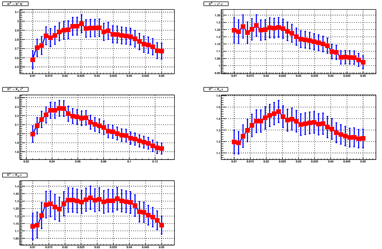
FIG. A.6 – Optimisation de \Delta E pour les cinq modes CP . \zeta , sur l'axe y , est définie dans la section 4.7.1. L'échelle est différente pour le mode K_S^0 \pi^0 .
