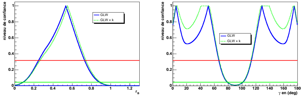
FIG. C.2 – Niveaux de confiance de r_B et \gamma de l'ajustement des \mathcal{R}_\pm et \mathcal{A}_\pm par CkmFitter [19] en variant k entre 0,8 et 1. Les droites rouge et verte correspondent à un et deux écarts type.
