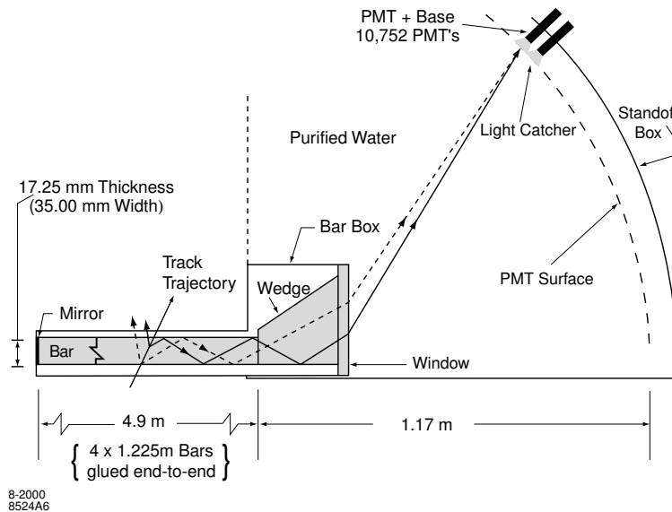
FIG. 3.11 – Schéma illustrant le principe de fonctionnement du DIRC. Une particule produit des photons Cherenkov dans les barres de quartz. Certains de ces photons se propagent par réflexion totale jusqu'au bout des barres avec une possible réflexion dans le miroir et puis ensuite dans une cuve d'eau ( n_{\text{eau}} = 1,33 ) appelé SOB ( Stand Off Box ) et finissent dans des photo-multiplieurs. L'information sur l'angle Cherenkov est conservée au cours du voyage des photons et l'utilisation de l'information venant de plusieurs photons permet de donner sans ambiguïté une estimation de l'angle Cherenkov.
