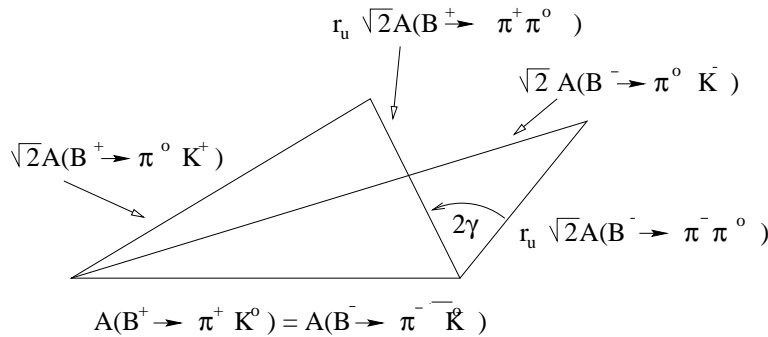
FIG. 2.6 – Relations triangulaires des désintégrations B^+ \rightarrow \pi^+\pi^0, \pi^+K^0, \pi^0K^+ en utilisant la symétrie de saveur SU(3) et en négligeant les contributions des diagrammes pingouin électrofaible (méthode GRL).
