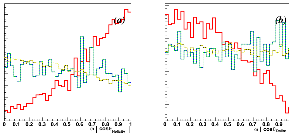
FIG. 4.10 – Les distributions angulaires pour (a) l'hélicité normale de \omega et (b) l'angle Dalitz \omega . La ligne continue correspond au signal, la ligne hachurée claire correspond au Monte Carlo q\bar{q} et celle foncée et hachurée correspond au Monte Carlo B\bar{B} . Ce graphe est produit après présélection.
