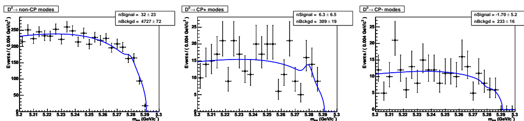
FIG. 5.7 – Distribution après ajustement par Argus + \mathcal{G} gaussienne dans les ailes de \Delta E pour les (a) modes non- CP , (b) modes CP+ , (c) modes CP- .
