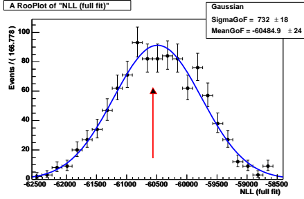
FIG. 5.12 – La distribution de maximum de vraisemblance à partir de 1000 simulations Monte Carlo rapides. La flèche correspond à la valeur du maximum de vraisemblance de l'ajustement CP final sur les données.
