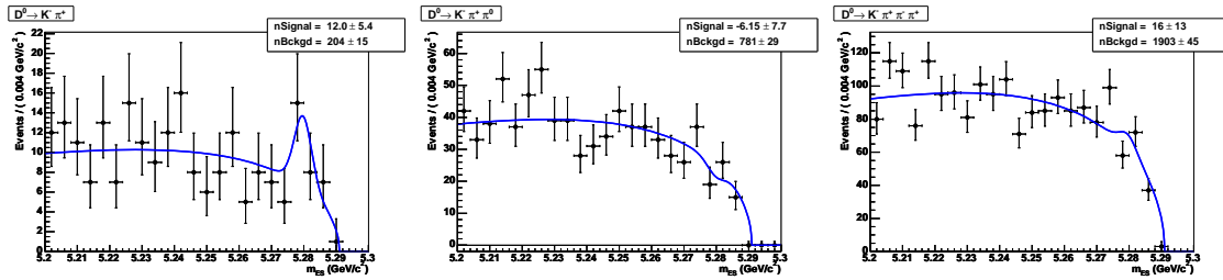
FIG. 5.4 – Distributions en m_{ES} des modes (a) K^- \pi^+ (b) K^- \pi^+ \pi^0 (c) K^- \pi^+ \pi^- \pi^+ pour 210,7 \text{ fb}^{-1} de données prises dans les ailes de m(D^0) .
