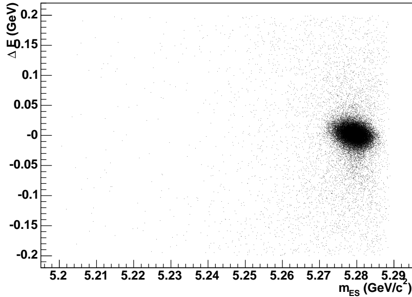
FIG. 4.15 – Le plan m_{ES}-\Delta E pour le Monte Carlo de signal des candidats B reconstruits dans les modes CP+ . Les évènements hors de la tache correspondent à des évènements mal reconstruits.
