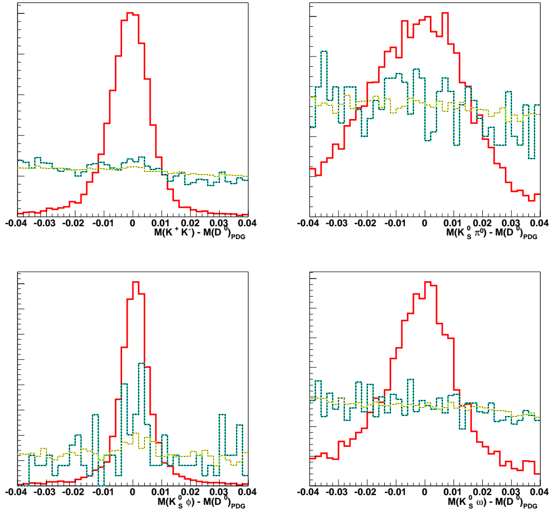
FIG. 4.13 – Les distributions de masse invariante des candidats D^0 pour les modes (a) K^+ K^- (b) K_S^0 \pi^0 (c) K_S^0 \phi (d) K_S^0 \omega . La distribution du \pi^+ \pi^+ n est pas affichée. Elle est très proche de celle du mode K^+ K^- . La ligne continue correspond au signal, la ligne hachurée claire correspond au Monte Carlo q\bar{q} et celle foncée et hachurée correspond au Monte Carlo B\bar{B} . Ce graphe est produit après présélection.
