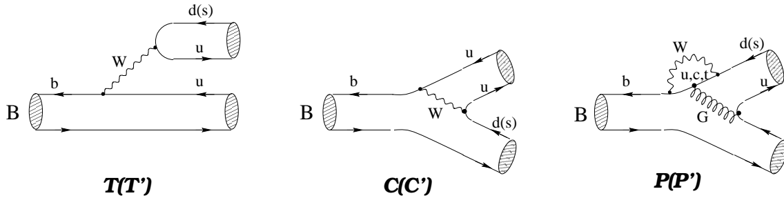
FIG. 2.5 – Diagrammes de Feynman dominant les désintégrations à deux corps sans charme. Le ' correspond aux désintégrations avec un quark s dans l'état final. On néglige les diagrammes d'annihilation et ceux des pingouins électrofaibles.
