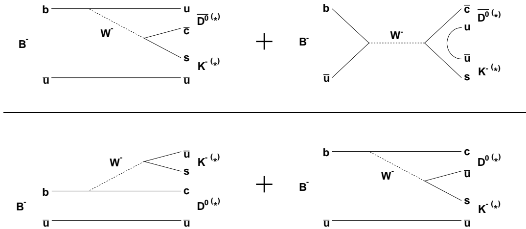
FIG. 2.1 – Diagrammes de Feynman pour les modes B^- \rightarrow D^{0(*)} K^{-(*)} et B^- \rightarrow \bar{D}^{0(*)} K^{-(*)} . Les diagrammes de gauche sont les diagrammes dominant les interférences et sont ceux que l'on considère généralement. Les diagrammes de droite ont la même phase que ceux de gauche et changent légèrement le rapport r_B , défini par la formule 2.5.
