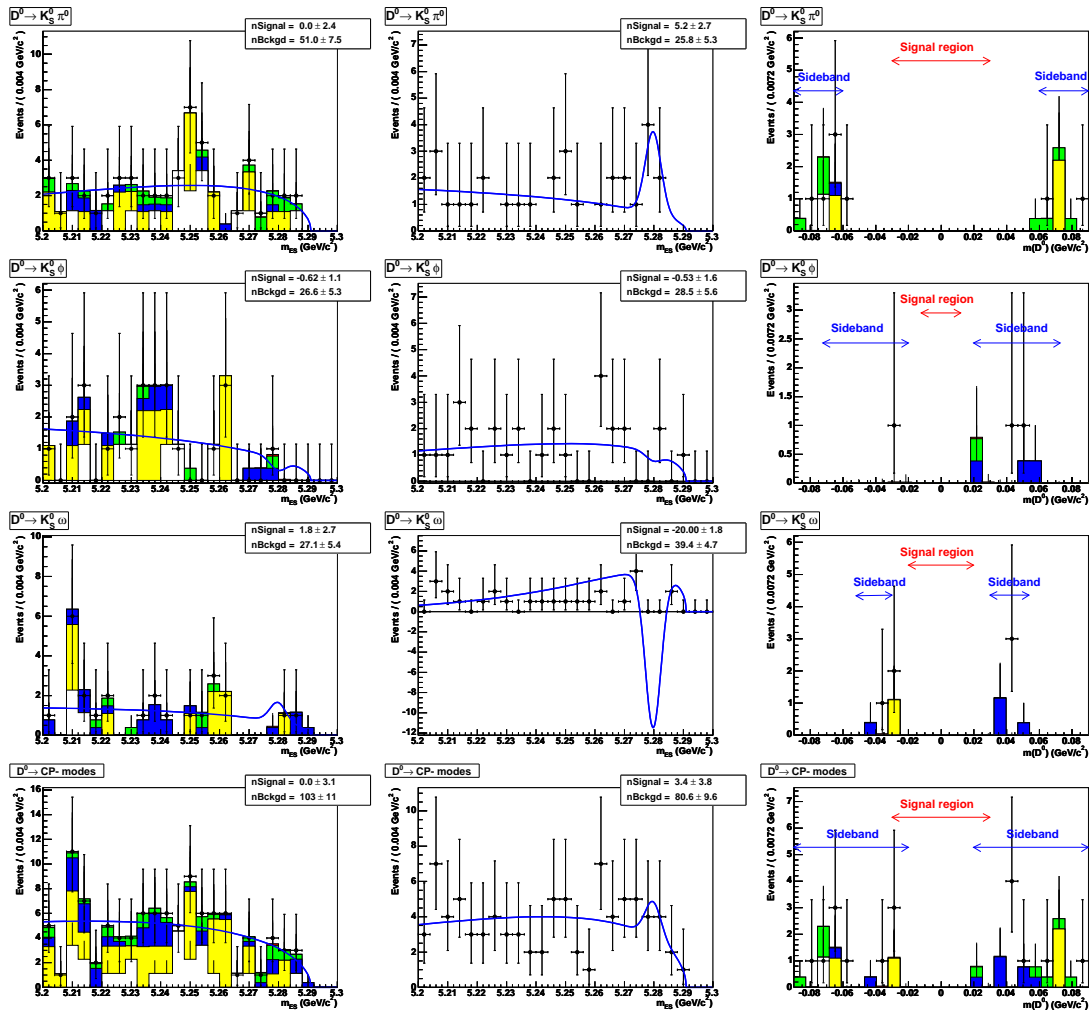
FIG. 5.6 – Les distributions D^0_{CP-} dans les ailes de m(D^0) pour 210,7 \text{ fb}^{-1} . La première ligne correspond au mode K_S^0 \pi^0 , la seconde au mode K_S^0 \phi , la troisième au mode K_S^0 \omega et la dernière au trois modes combinés. La première colonne présente la distribution en m_{ES} de Monte carlo générique et la seconde celle des données réelles, après sélection sur m(D^0) dans la région fléchée dans la troisième colonne. Les ajustements des distributions en m_{ES} (Gaussienne + Argus) donnent une idée de la contribution du bruit de fond non charmé.
