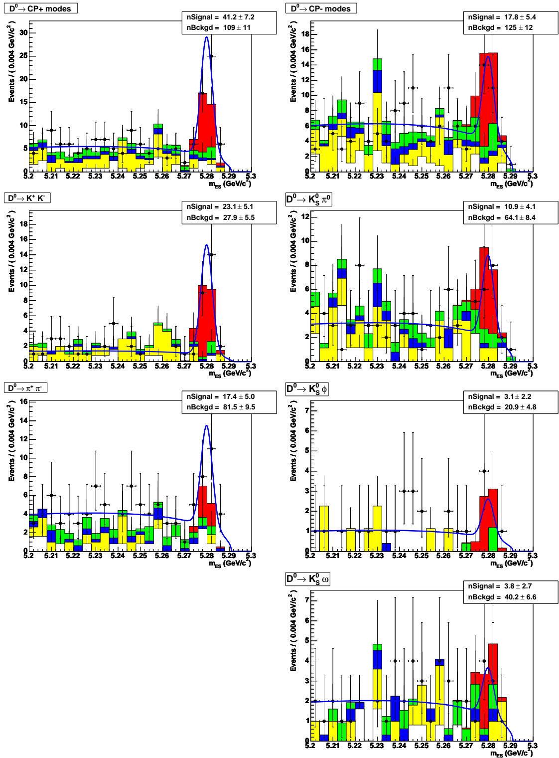
FIG. 4.23 – Comparaison des distributions de données et de simulation en m_{ES} des désintégrations B^- \rightarrow D_{\pm}^0 K^{*\mp} pour 210,7 \text{ fb}^{-1} . Les ajustements sont fait par une \mathcal{A} rgus plus une \mathcal{G} aussienne. Le paramètre de la fonction d'Argus est fixé à -22,2 , la valeur centrale et la largeur de la \mathcal{G} aussienne sont respectivement fixées à \mu = 5279,84 \text{ MeV}/c^2 et \sigma = 2,56 \text{ MeV}/c^2 . Les points correspondent aux données et les histogrammes à la simulation Monte Carlo pour r_B = 0 . La colonne de gauche correspond aux distributions des modes CP+ et celle de droite aux CP- . La première ligne est la superposition des modes CP . Le signal est représenté en rouge, le bruit de fond venant du continuum u\bar{u} d\bar{d} s\bar{s} en blanc, celui du c\bar{c} en jaune et le bruit de fond B^+ B^- B^0 \bar{B}^0 en vert-bleu.
