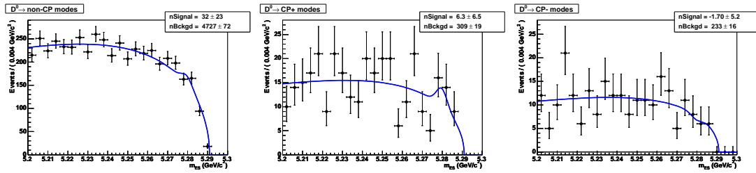
FIG. 5.7 – Distribution après ajustement par Argus + \mathcal{G} aussienne dans les ailes de \Delta E pour les (a) modes non- CP , (b) modes CP+ , (c) modes CP- .
