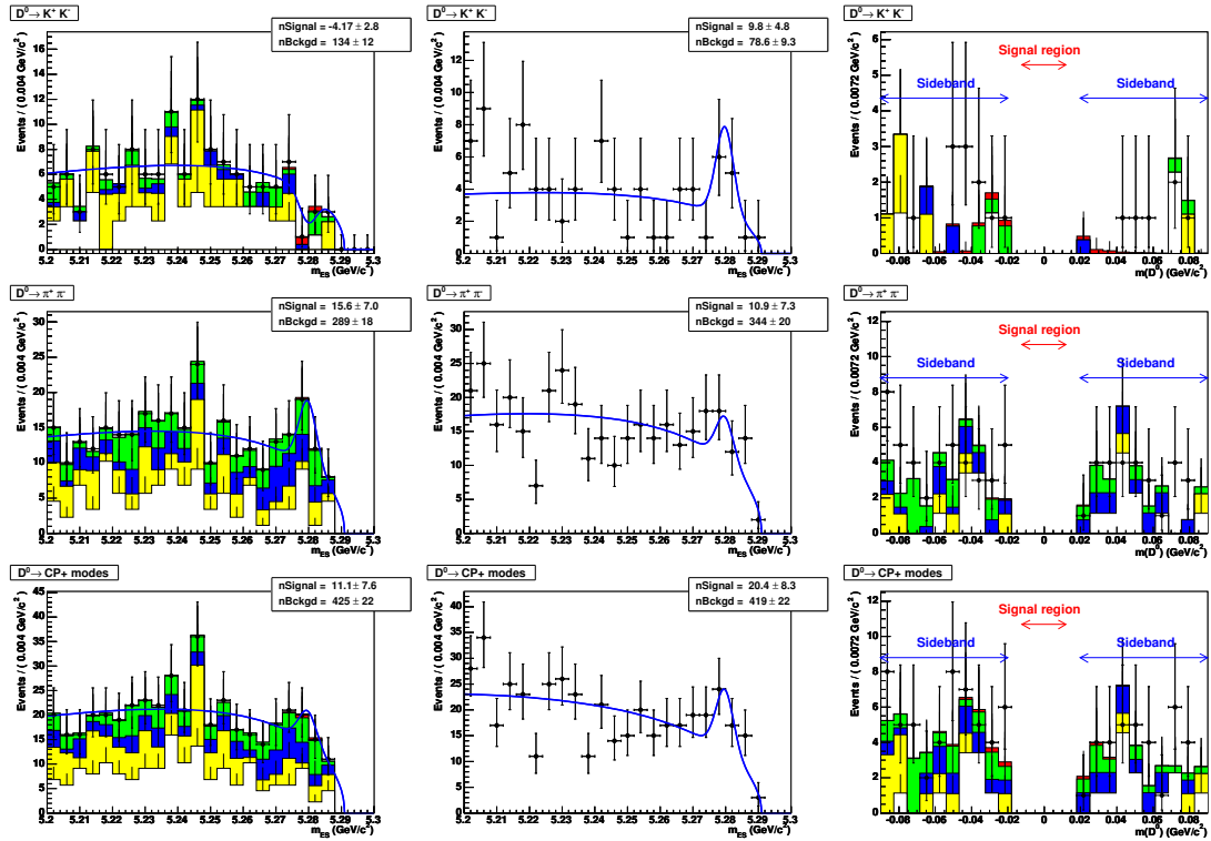
FIG. 5.5 – Les distributions de D_{CP^+}^0 dans les ailes de m(D^0) pour 210,7 \text{ fb}^{-1} . La première ligne correspond au mode K^+ K^- , la seconde au mode \pi^+ \pi^- et la troisième pour les deux combinés. La première colonne présente la distribution en m_{ES} de Monte carlo générique et la seconde celle des données réelles, après sélection sur m(D^0) dans la région fléchée dans la troisième colonne. Les ajustements des distributions en m_{ES} (Gaussienne + Argus) donnent une idée de la contribution du bruit de fond non charmé.
