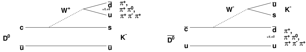
FIG. 2.8 – Diagrammes de Feynman pour les désintégrations des modes non- CP et ADS . Le diagramme de gauche est favorisé de Cabibbo et celui de droite est doublement supprimé.
