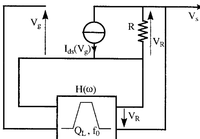
Figure 23 : Schéma de l'oscillateur étudié.
