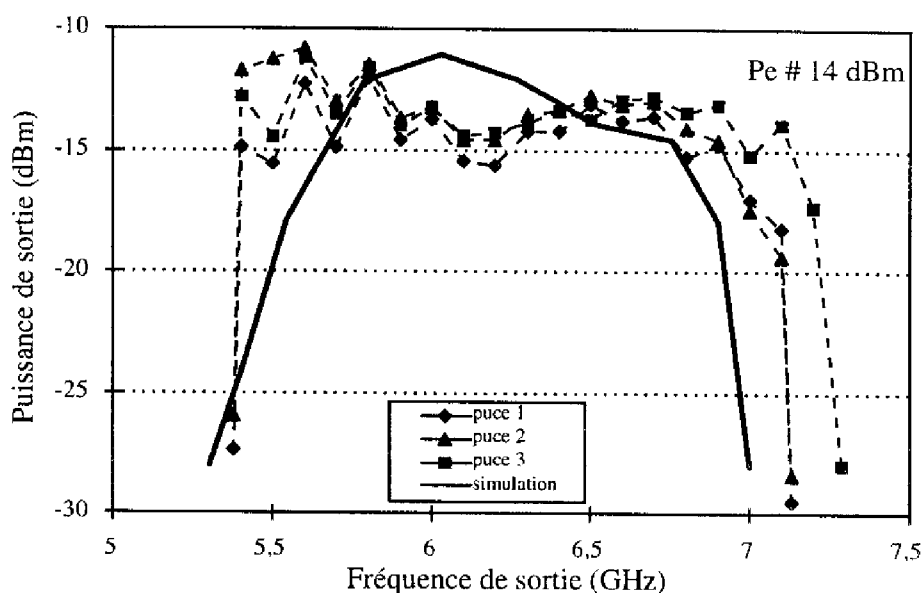
Figure 8 : Bandes de synchronisation [simulation (trait plein), mesures (trait pointillé)]
