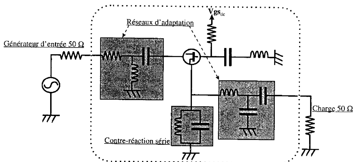
Figure 22 : Nouvelle topologie de diviseur de fréquence.
