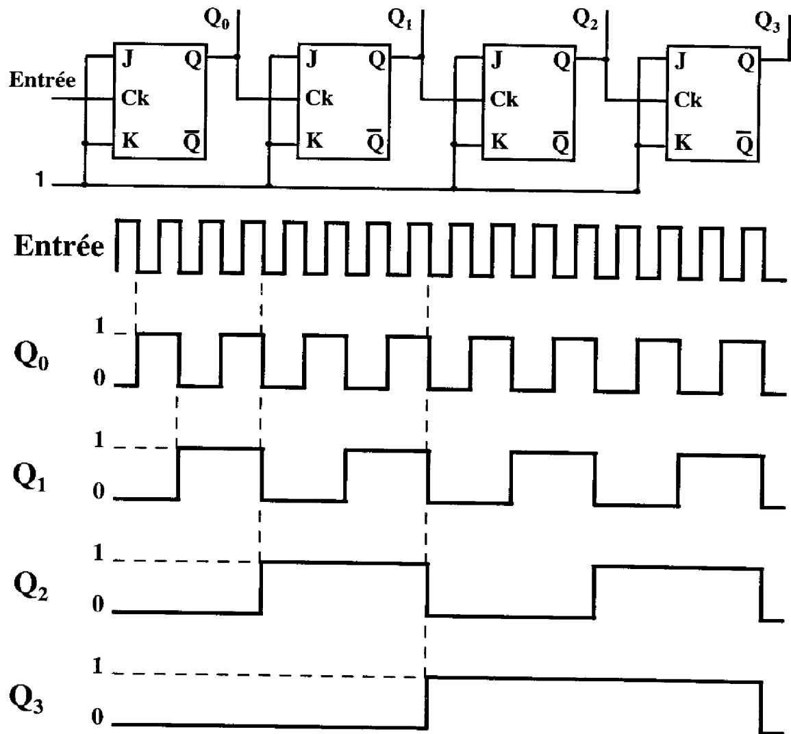
Figure 3 : cascade de bascules JK et chronogramme des sorties successives.
