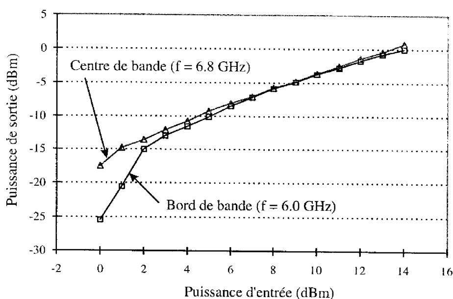
Figure 23 : Puissance de sortie en fonction de la puissance d'entrée.
