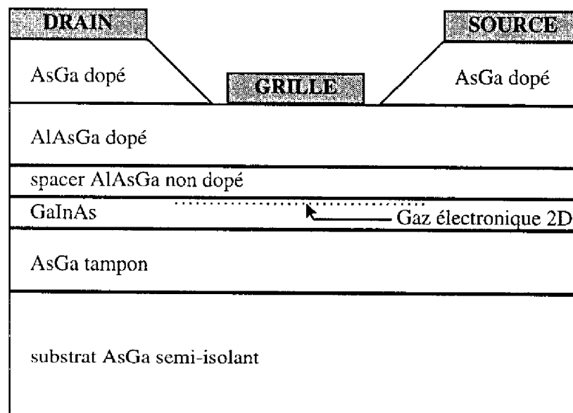
Figure 1 : Schéma d'un empilement classique de couches dans un PHEMT.
