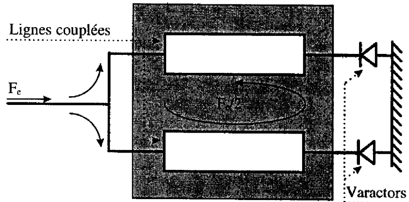
Figure 18 : Schéma du diviseur paramétrique présenté par Harisson.
