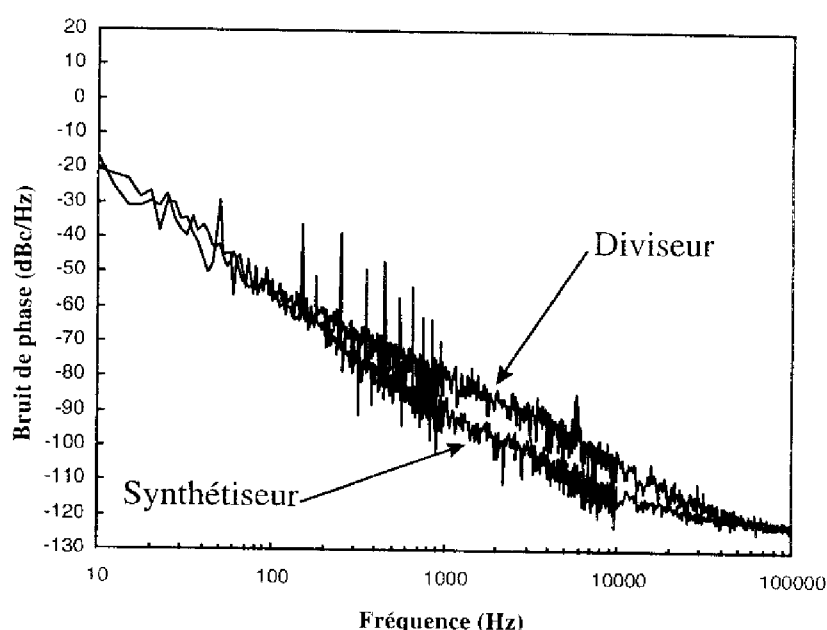
Figure 11 : Mesure du bruit de phase du diviseur de fréquence. ( 12.4 GHz - 6.2 GHz)
