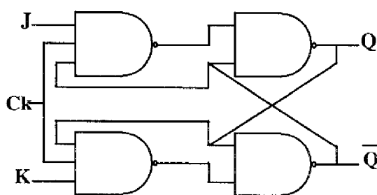
Figure 1 : bascule JK à base de portes Non-ET.
