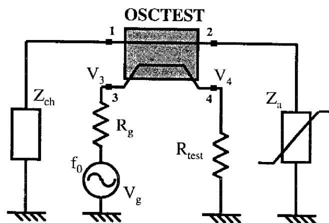
Figure 4 : module 'OSCTEST'
