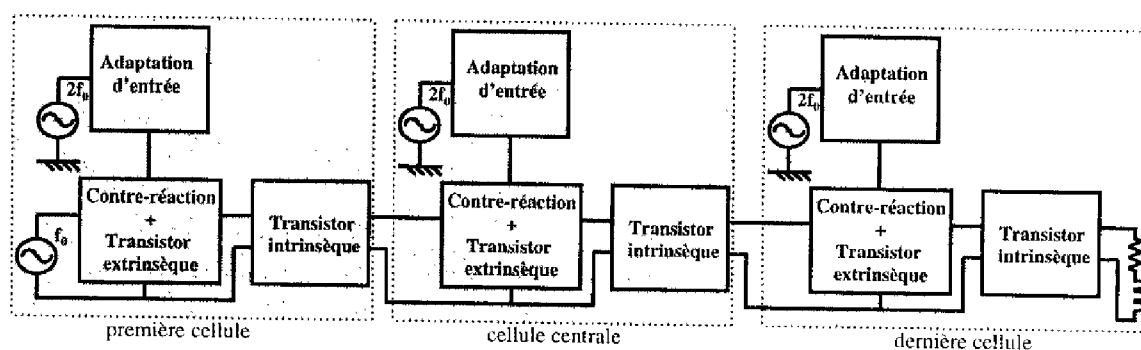
Figure 17 : Schéma synoptique d'une chaîne de diviseurs en boucle ouverte.
