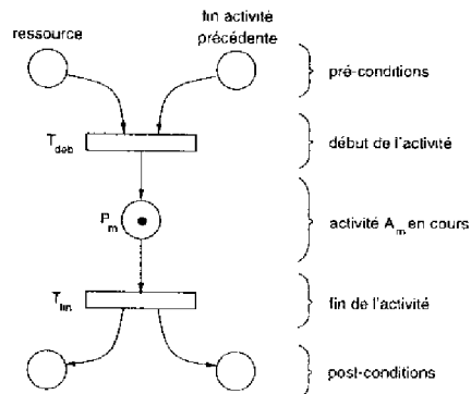
FIG. 1.6 – modélisation par réseaux de Petri d'une activité de commande
