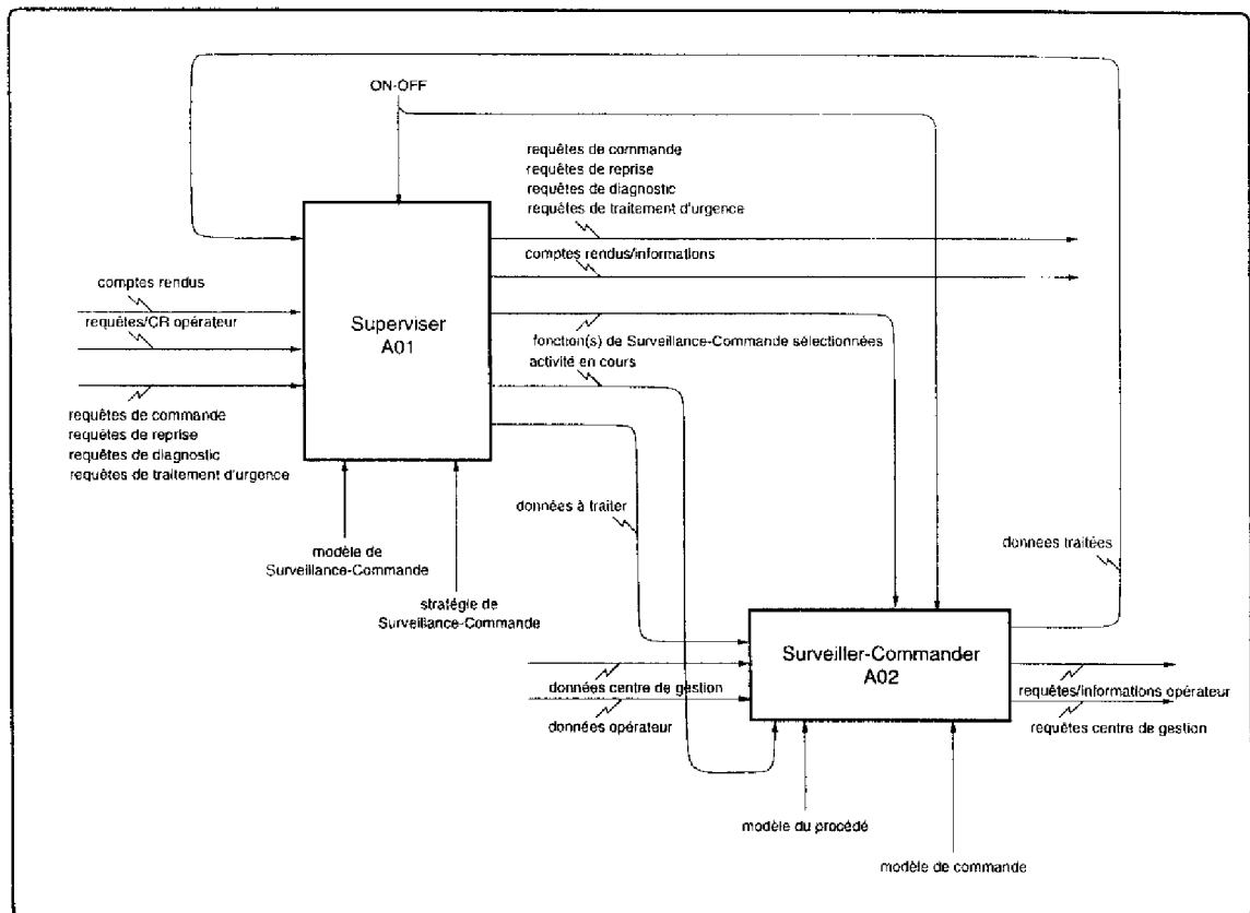
FIG. 2.3 – diagramme A0
