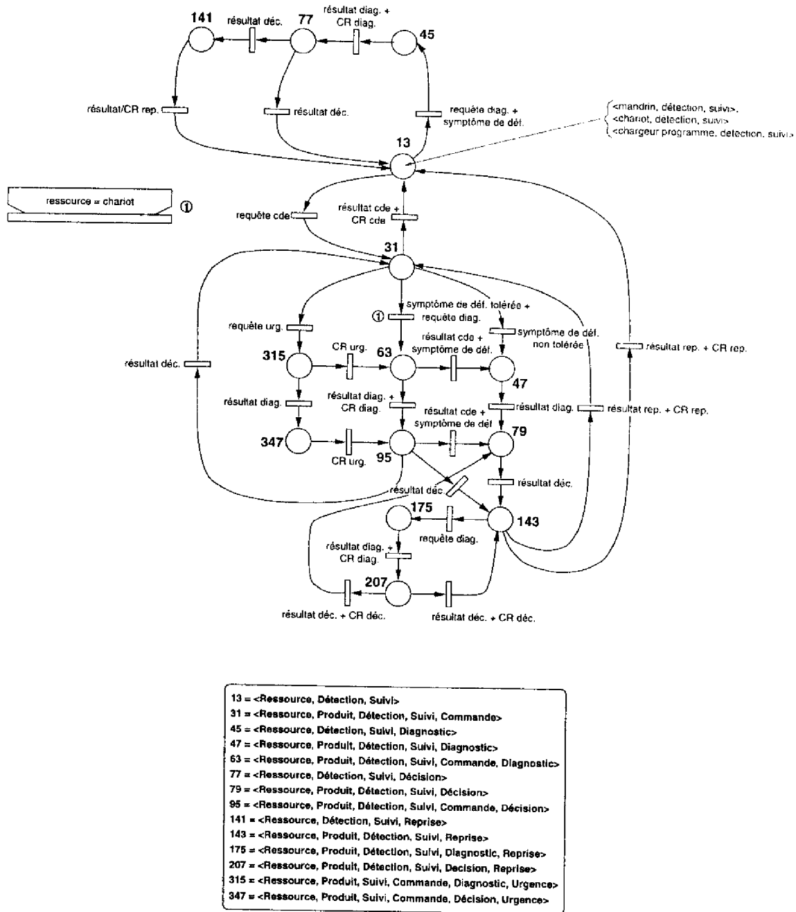
FIG. 1.7 – stratégie de surveillance-commande pour le module Tour
