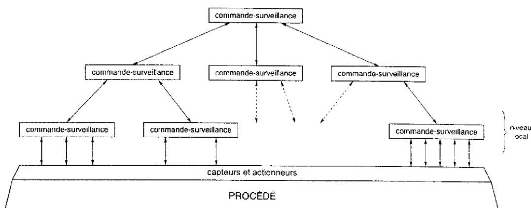
FIG. 2.1 – structure hiérarchique et modulaire de commande surveillance
