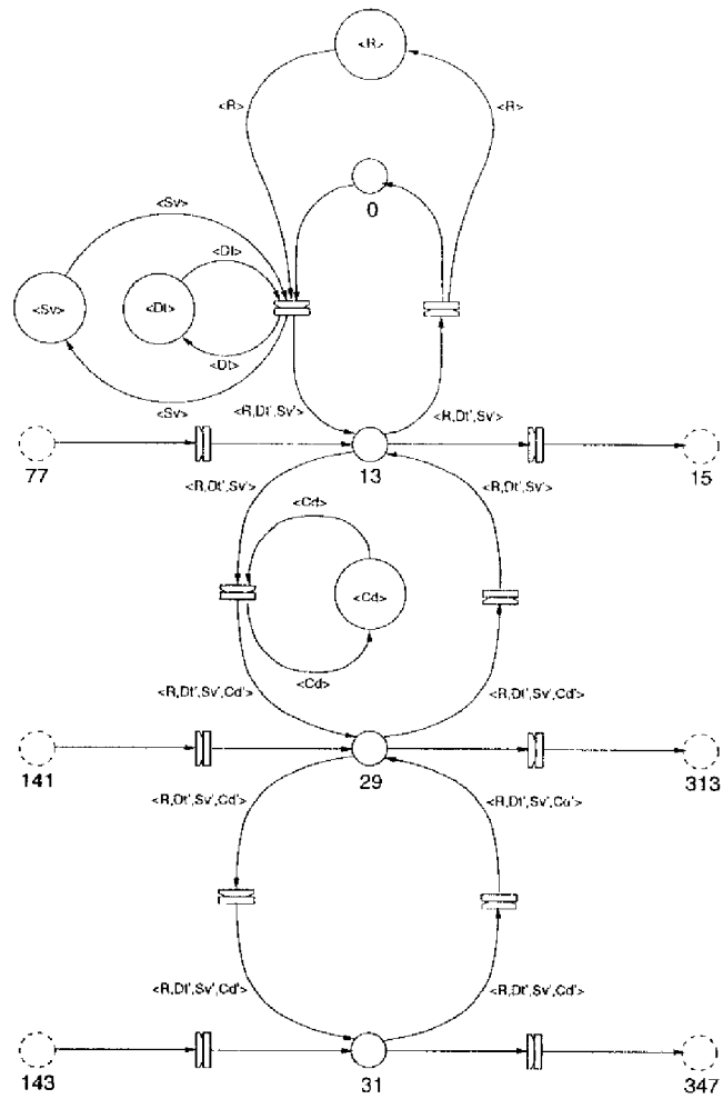
FIG. 3.4 – extrait du modèle de référence pour la surveillance-commande
