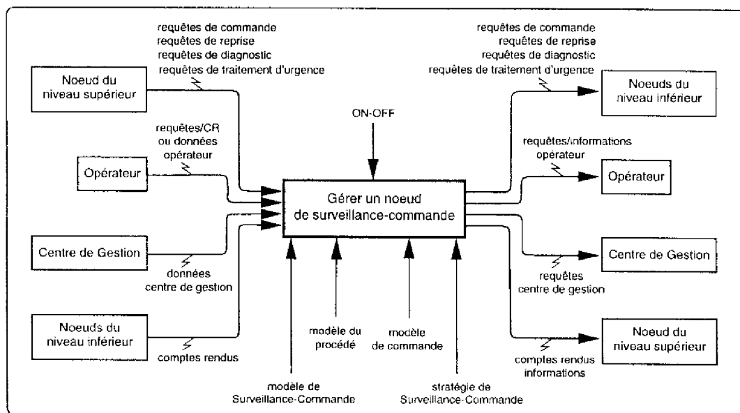
FIG. 2.2 - diagramme A-0
