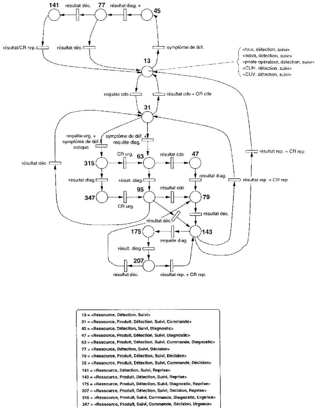
FIG. 1.6 – stratégie de surveillance-commande pour le module Coordination
