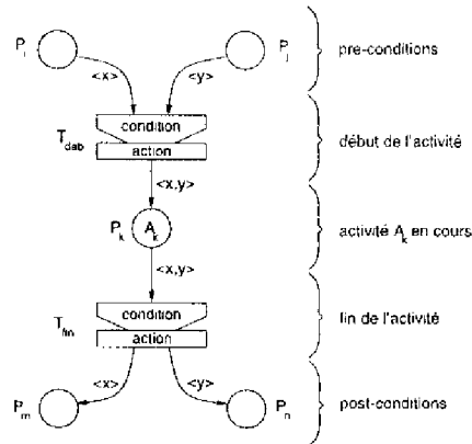
FIG. 3.2 – activité de commande modélisée par RdPO
