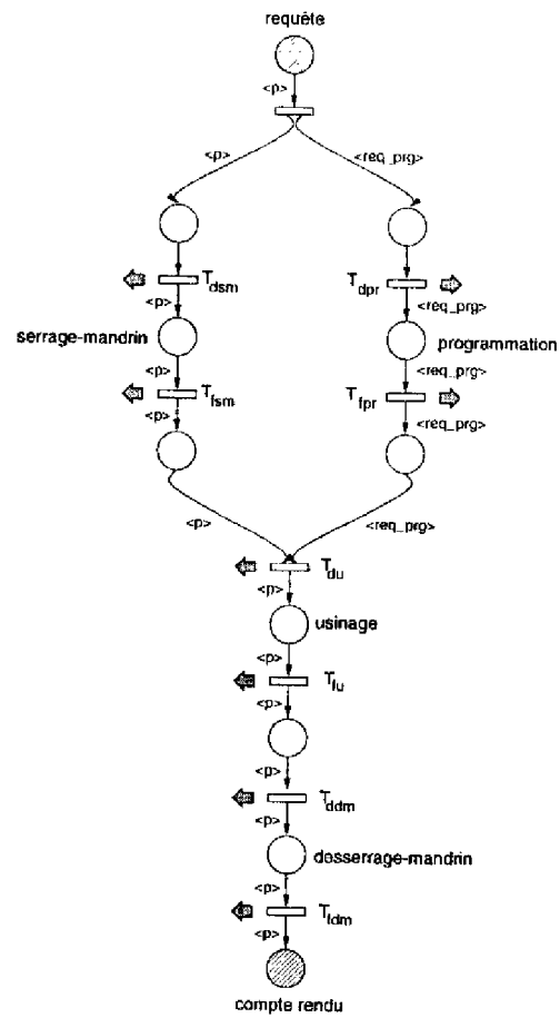
FIG. 2.6 – séquence de commande dans le module Tour
