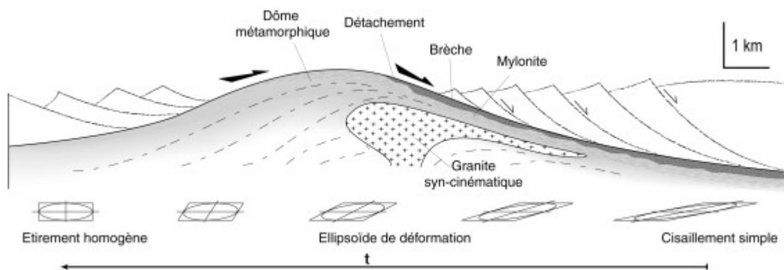
Figure II.2 : Evolution de la déformation d'un dôme vers le détachement. Le cœur dôme (ici intrusé par un granite syn-cinématique du jeu de la zone de cisaillement) est affecté par un étirement homogène ductile, qui évolue vers un cisaillement simple de plus en plus prononcé vers le détachement (mylonite). La mylonite est reprise par une zone de brèches sous le contact entre compartiments inférieur et supérieur. La coupe structurale représente une coupe "temps" de la déformation au cours de l'évolution en détachement de la zone de cisaillement.
