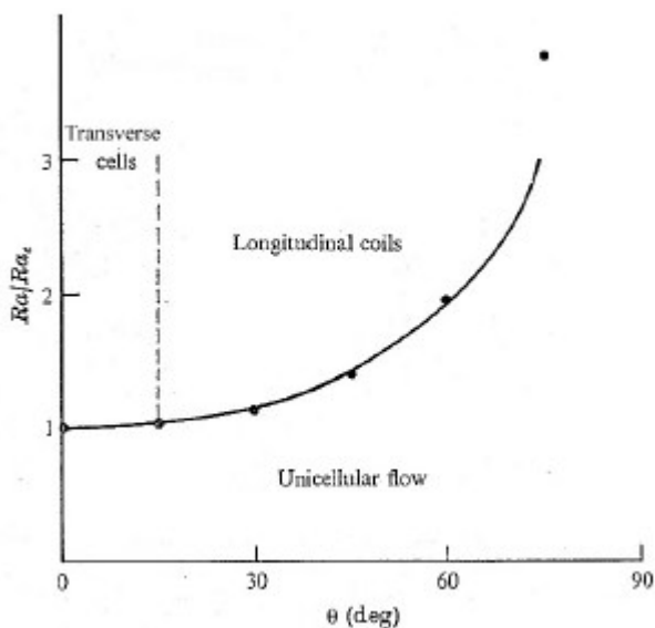
Figure A5.1 : Géométrie des cellules de convection en fonction du rapport Ra/Ra_{\text{critique}} et de l'inclinaison de l'horizon perméable, d'après Bories & Combarous (1973). Trait noir : relation théorique. Points noirs : données expérimentales.
