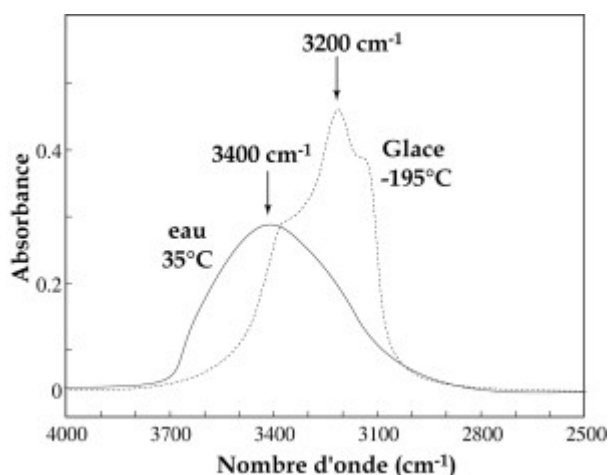
Figure VI.2 : (à droite) Variation de la position du spectre IR de l'eau pure en fonction de la température (figure de Aines & Rossman, 1984, d'après les données de Eisenberg & Kauzmann, 1962). Le pic apparent de la glace à -195\text{ }^{\circ}\text{C} est à 3200\text{ cm}^{-1} . Le pic apparent de l'eau liquide à 35\text{ }^{\circ}\text{C} est à 3400\text{ cm}^{-1} .
