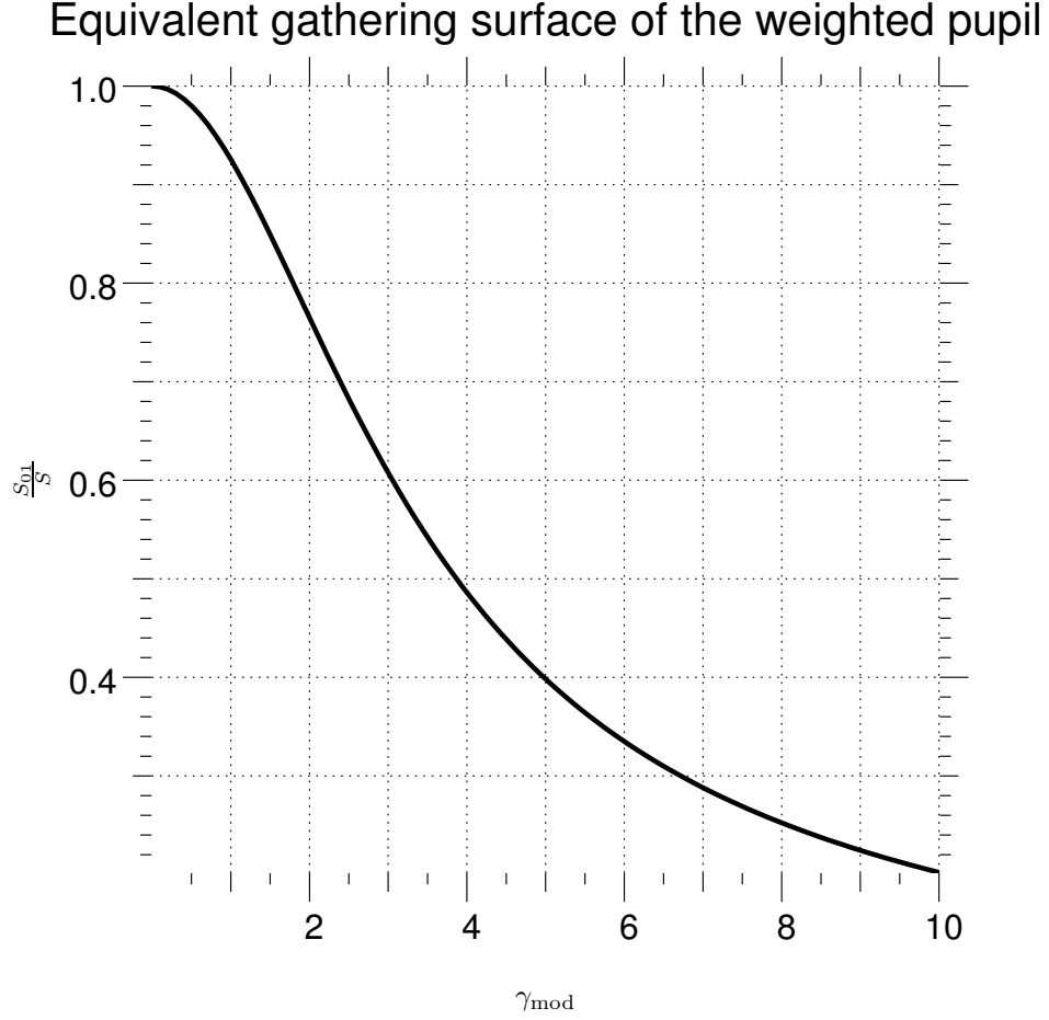
Fig. 5.11 – Surface effective S_{01} de la pupille effective P_{01} rapportée à la surface du d'un Telescope Auxiliaire (AT) du VLTI. \gamma_{\text{obs}} = 1\% comme fonction du rapport d'injection \gamma_{\text{mod}} . L'injection optimale \gamma_{\text{mod}} = 1.213 la surface effective est 91.36% celle de AT. Le cas limite où un trou infiniment fin sert de filtre spatial S_{01} = S .
