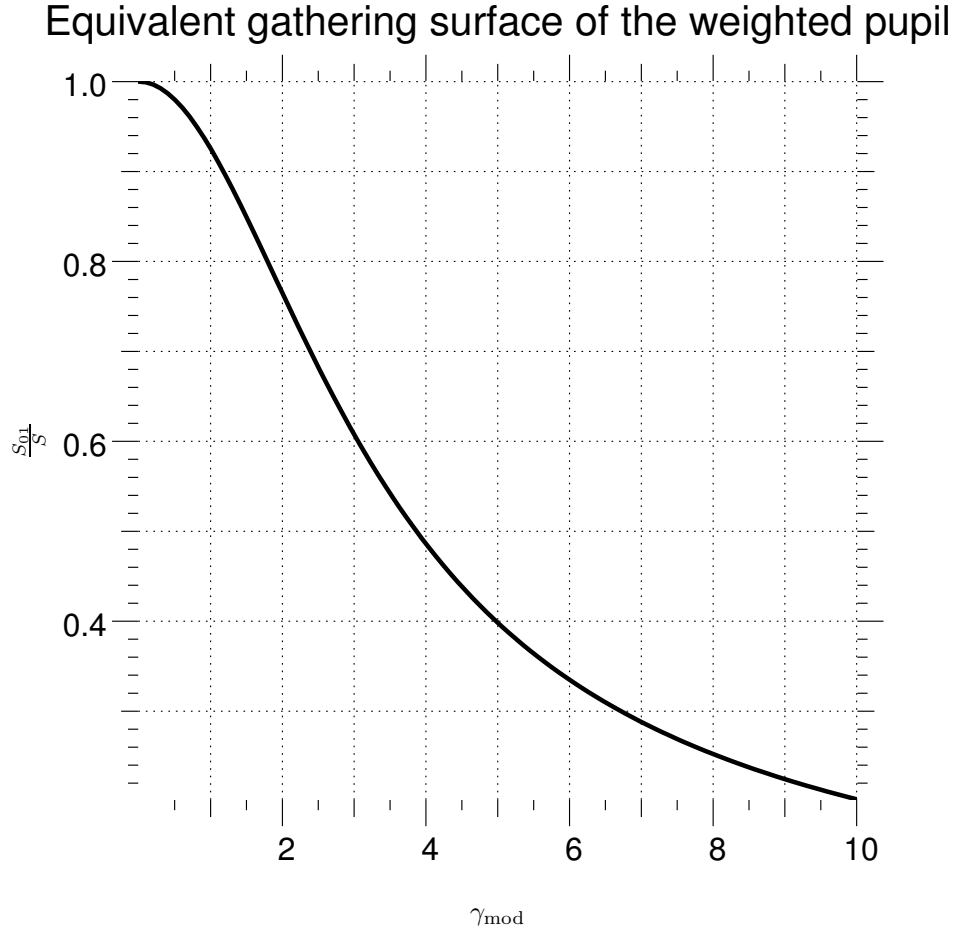
Fig. 5.11 – Surface effective S_{01} de la pupille effective P_{01} rapportée à la surface d'un Telescope Auxiliaire (AT) du VLTI. \gamma_{\text{obs}} = 1\% comme fonction du rapport d'injection \gamma_{\text{mod}} . L'injection optimale \gamma_{\text{mod}} = 1.213 la surface effective est 91.36% celle de AT. Le cas limite où un trou infiniment fin sert de filtre spatial S_{01} = S .
