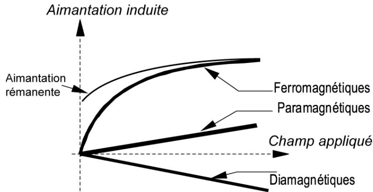
Figure II-6: Comportements magnétiques en fonction du champ appliqué.
