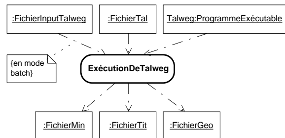
FIG. G.1 – Modélisation de l'exécution du programme TALWEG.
