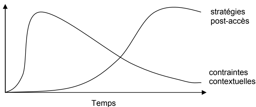
Figure 9. Evolution temporelle de l'effet du contexte sur l'accès à la signification et des stratégies postérieures à l'accès.
