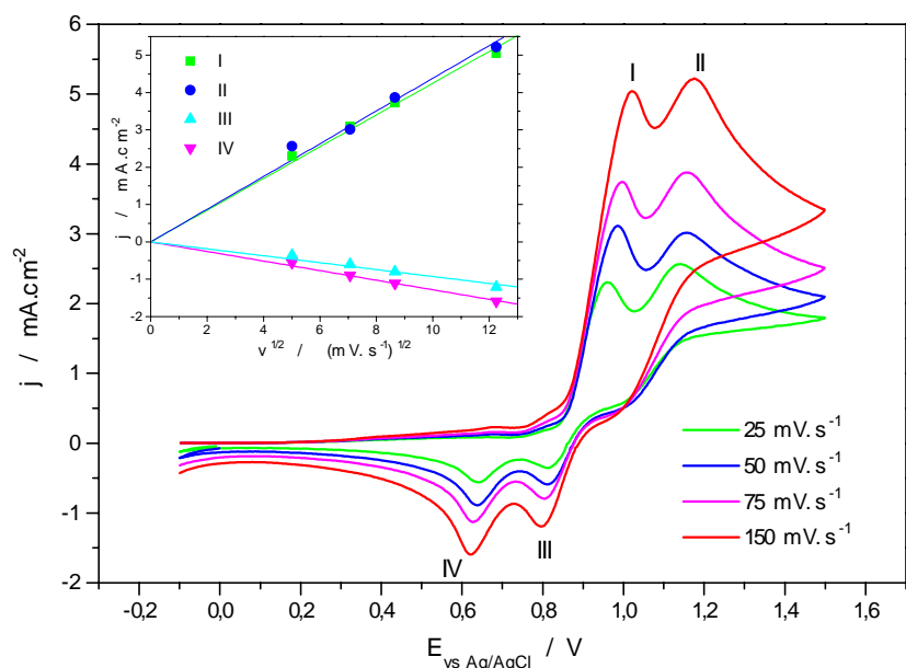
II.14. Courants d'oxydation et de réduction des oligomères de DPA en fonction de la racine de la vitesse de balayage. Les courants d'oxydation (I, II) et de réduction (III, IV) sont linéairement dépendants de la racine de la vitesse de balayage, indiquant un mécanisme limité par diffusion. Les courants d'oxydation sont positifs et les courants de réduction sont négatifs. Les courbes sont enregistrées à 25, 50, 75 et 150 mV.s -1 .
