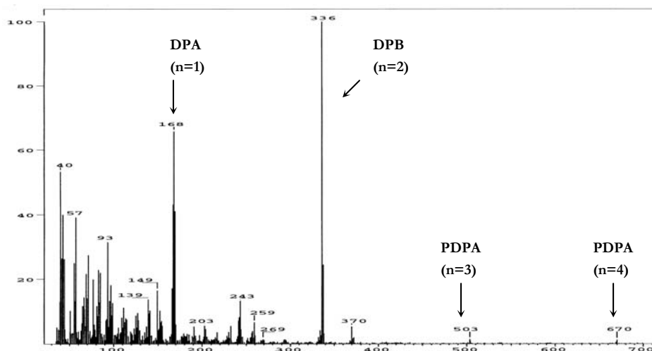
Figure II.3 : Spectre de masse des produits PDPA1 et PDPA2. Les pics sont attribués à DPA, DPB, et à des oligomères (n = 1, 2, 3, 4).
