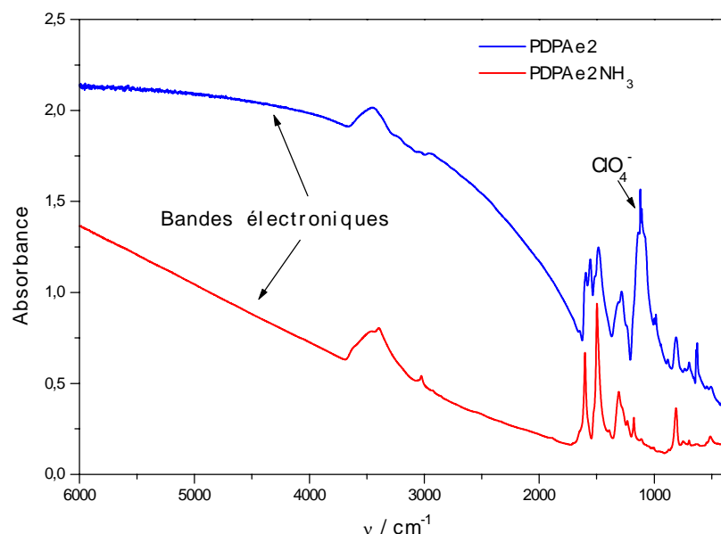
Figure II.6 : Spectre IR de PDPAe2 (bleu) et PDPAe2NH 3 (rouge).
