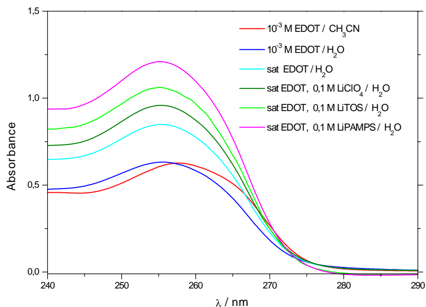
Figure II.42 : Absorbance UV de l'EDOT dans différentes conditions.
