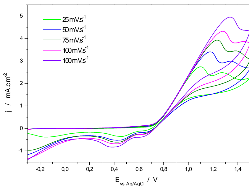
II.15 : Courbes de voltampérométrie cyclique (V) de la polydiphénylamine (PDA) dans l'acétonitrile (AN) à 25 mV.s -1 , 50 mV.s -1 , 75 mV.s -1 , 100 mV.s -1 et 150 mV.s -1 . Les conditions de mesure sont : [PDA] = 10 -3 mol/L, [TBA] = 0,1 mol/L, [LiClO 4 ] = 0,1 mol/L, [AN] = 0,1 mol/L, v sc = 10 mV/s, T = 50°C.
