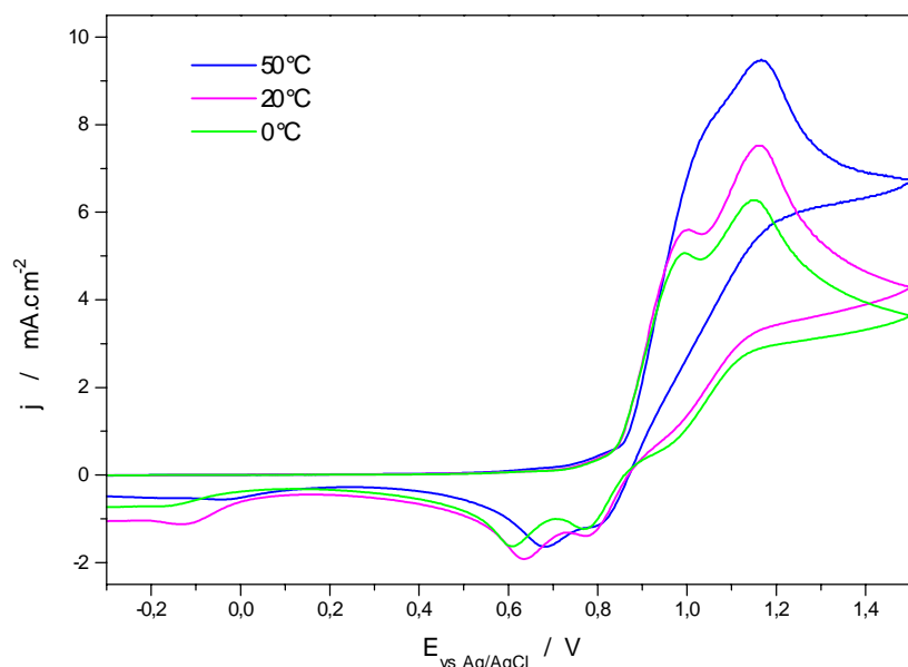
II.14 : Courbes de voltampérométrie cyclique (V) de la polydiphénylamine (PDA) dans l'acétonitrile (AN) à 50°C, 20°C et 0°C. Les conditions de mesure sont : [PDA] = 10 -3 mol/L, [TBA] = 0,1 mol/L, [LiClO 4 ] = 0,1 mol/L, [AN] = 0,1 mol/L, v sc = 10 mV/s, T = 50°C, 20°C, 0°C.
