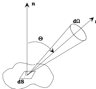
Figure I.7 : Définition de la luminance directionnelle spectrale.
