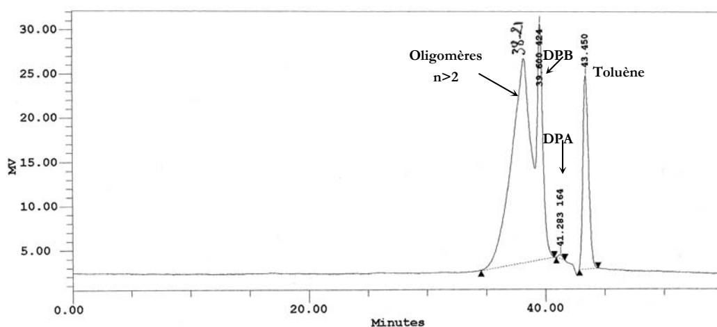
Figure II.2 : Chromatogramme SEC des produits PDPA1 et PDPA2. Les pics sont attribués à DPA, DPB, et à des oligomères (n > 2). Le pic à 43.450 min correspond au toluène.
