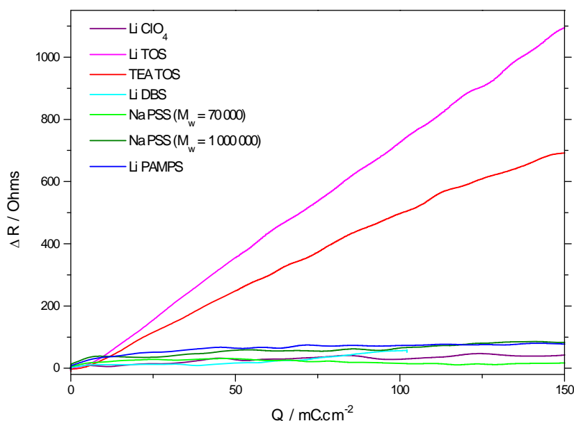
Figure II.46 : Résistance en fonction de la charge au cours de la polymérisation de EDOT dans différents électrolytes aqueux. Polymérisations de EDOT à 0,5 mA.cm^{-2} à partir de solutions aqueuses saturées en EDOT et 0,1 M en électrolyte.
