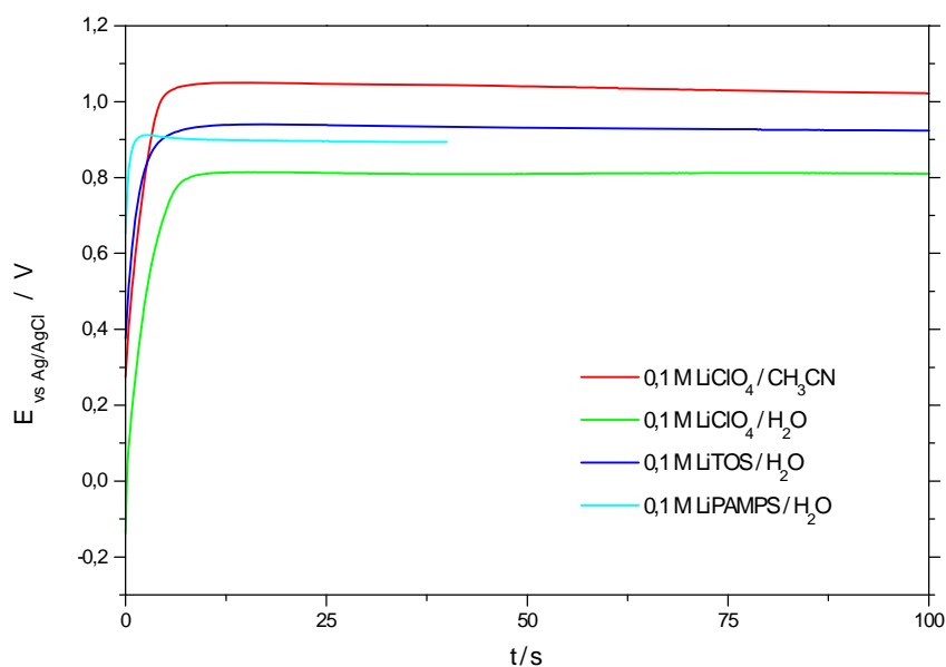
Figure II.43 : Electropolymérisations galvanostatiques de EDOT à 0,5 mA.cm -2 dans différentes solutions électrolytiques. (0,05 M EDOT dans CH 3 CN et solutions saturées en EDOT dans les milieux aqueux).
