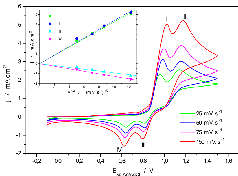
Figure II.14 : Voltammogrammes cycliques d'une solution de DPA 0,01M dans 0,1M TEABF 4 / CH 3 CN à différentes vitesses de balayage (T=-10°C). En insert, densités de courant maximales des pics anodiques et cathodiques en fonction de la racine carrée de la vitesse de balayage.
