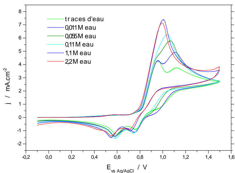
Figure II.16 : Voltammogrammes cycliques de solutions de DPA 0,01M dans 0,1M TEABF 4 / CH 3 CN pour différents teneurs en eau (100 mV.s -1 , T=-10°C).
