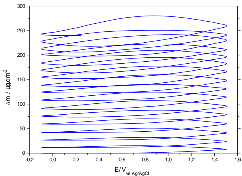
Figure II.26 : Evolution de la masse déposée sur le quartz pendant la voltammétrie cyclique d'une solution de DPA 0,01M dans 0,1M TEATOS / \text{CH}_3\text{CN} ( 100 \text{ mV}\cdot\text{s}^{-1} ).
