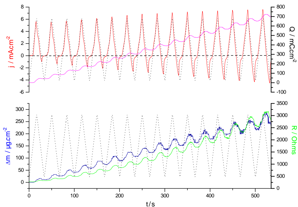
Figure II.25 : Potentiel, courant, charge, masse et résistance pendant la polymérisation par voltammétrie cyclique d'une solution de DPA 0,01M dans 0,1M TEATOS / \text{CH}_3\text{CN} ( 100 \text{ mV}\cdot\text{s}^{-1} ).
