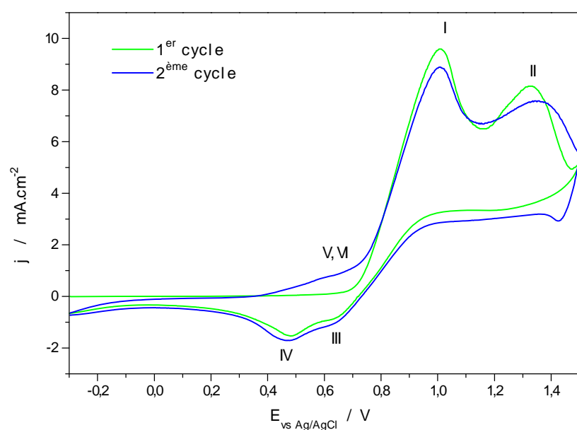
Figure II.13 : Voltammogrammes cycliques d'une solution de DPA 0,01M dans 0,1M TEATOS / \text{CH}_3\text{CN} ( 100 \text{ mV}\cdot\text{s}^{-1} ).
