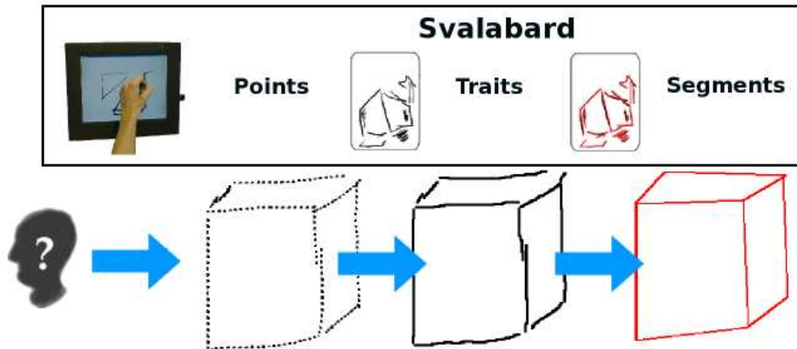
FIGURE 3.14 – De points aux segments. À gauche, les points reçus (dessin de l'utilisateur avec un périphérique d'entrée), transformés en traits au centre puis en segments géométriques à droite.
