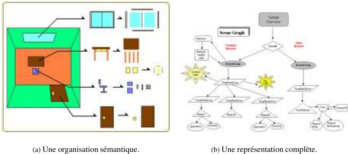
FIGURE 7.2 – Graphes de scènes. La figure (a) présente un graphe de scène ne représentant que les objets géométriques de la scène. Cette visualisation permet d’appréhender clairement l’organisation de la scène. La figure (b) est une représentation complète d’un graphe de scène, faisant apparaître les transformations et autres nœuds graphiques.
