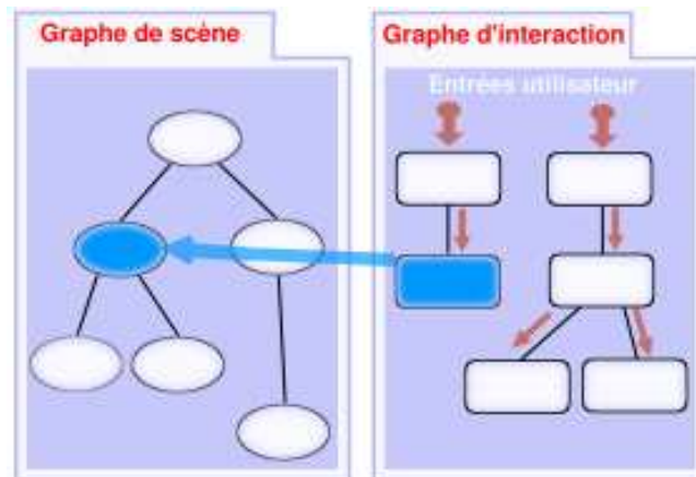
FIGURE 7.14 – Dispositifs manipulateurs. Un manipulateur communique avec un nœud spécifique et unique du graphe de scène.
