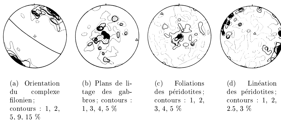
FIG. 1.12 – Diagrammes stéréographiques montrant l'orientation préférentielle des structures dans le Massif de Suma'il. Projection stéréographique dans l'hémisphère inférieur (extrait de Ceuleneer et al., 1988).
