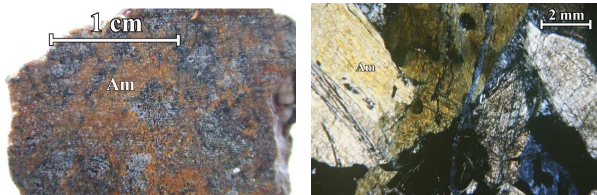
(a) Face sciée de l'échantillon
