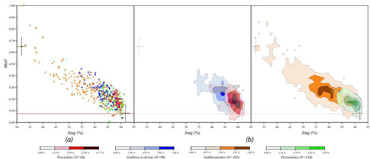
FIG. 3.21 – Diagrammes montrant l'évolution des compositions en manganèse des orthopyroxènes en fonction du Xmg et du type lithologique. (a) : Chaque point représente la composition moyenne pour un échantillon, la légende donnant la signification des symboles est donnée dans le tableau 2.3; (b) : les nuages de densité sont calculés sur l'ensemble des points d'analyse pour chaque famille lithologique.
