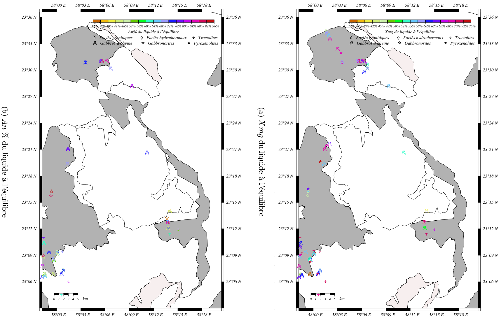
FIG. A.35 – Cartes géologiques des massifs de Kahwad et Musibit montrant les répartitions pour quelques caractères chimiques des liquides à l'équilibre.
