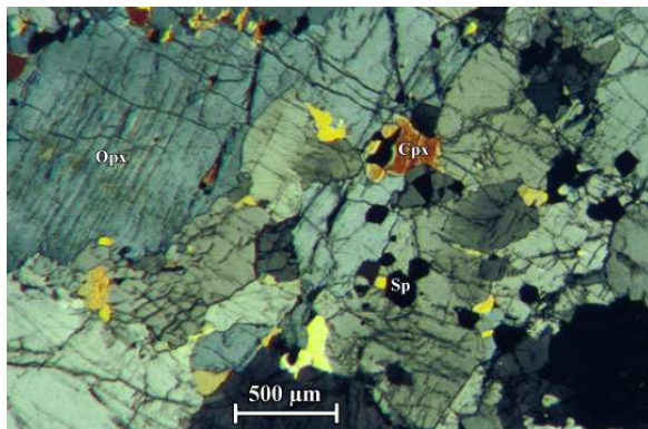
(a) Échantillon 00 FZ 30b
