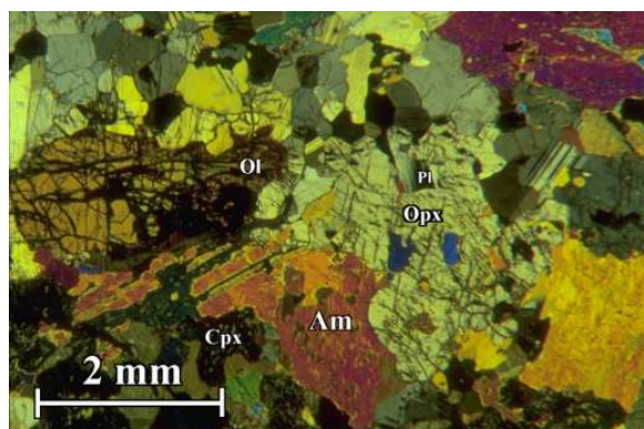
(b) Gabbrorite contenant de la hornblende, échantillon 01 MB 2
