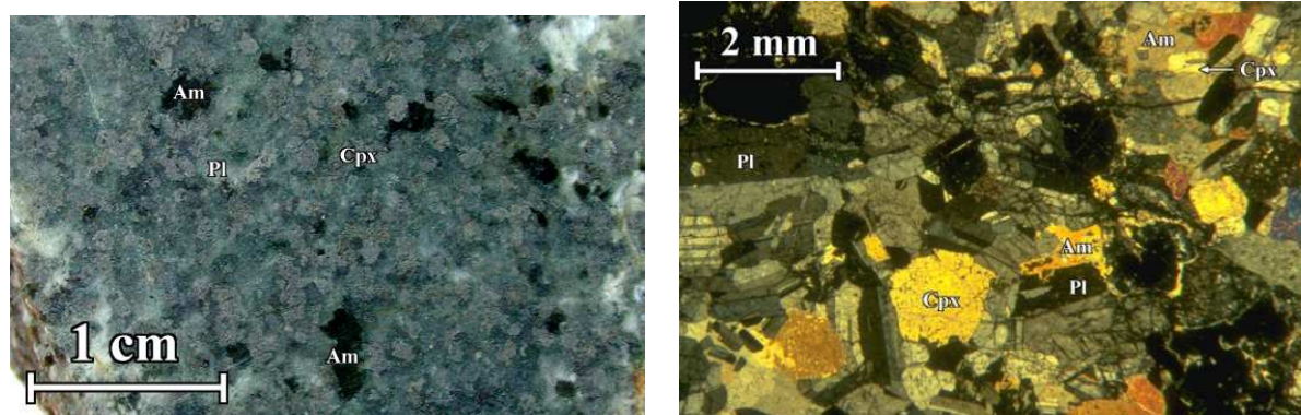
(a) Face sciée de l'échantillon
