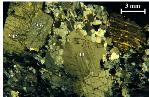
FIG. 2.68 – Échantillon de gabbro en cours de mylonitisation, la recristallisation se limite aux joints de grains et les grains les plus fins se trouvent à la limite entre les orthopyroxènes et les plagioclases (massif de Fizh, échantillon 00 FZ 33a). Lumière polarisée avec nicols croisés.
