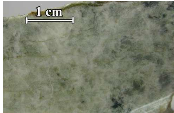
FIG. 2.141 – Face sciée d'un échantillon de clinopyroxénite formée de diopsides purs (massif de Samad, échantillon 99 SD 16).
