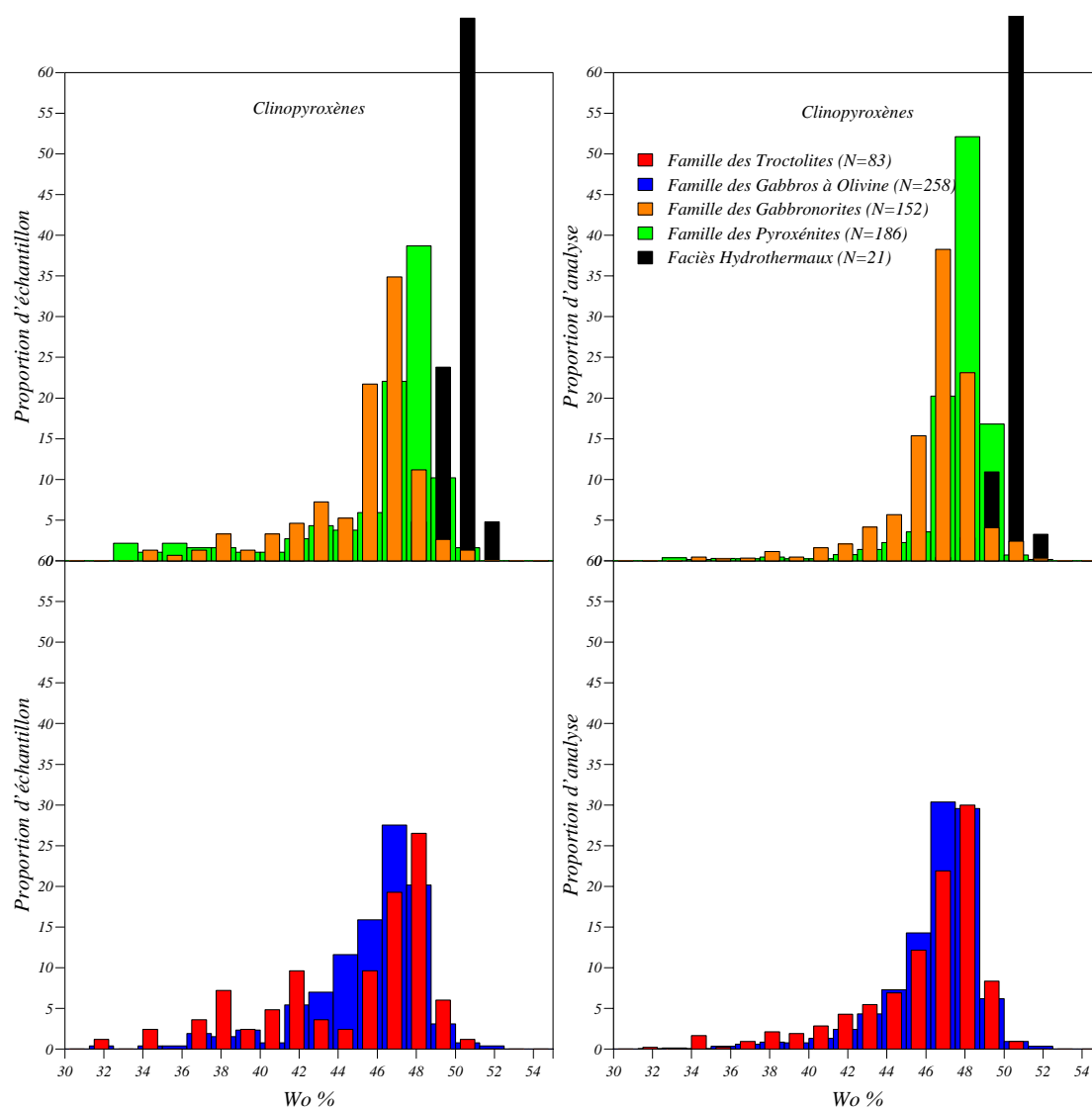
(a) Composition moyenne par échantillon
