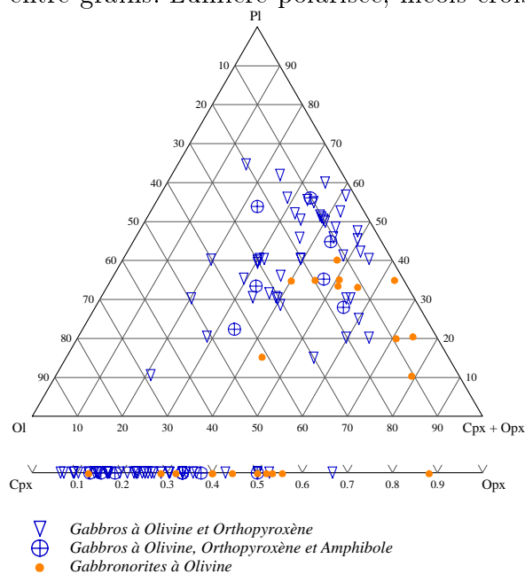
FIG. 2.54 – Diagramme représentant les compositions modales des gabbrorites à olivine (gabbros à olivine et orthopyroxène, gabbrorites à olivine dont l'orthopyroxène est précoce) dans le système ternaire plagioclase (Pl) – olivine (Ol) – pyroxènes (Cpx + Opx).
