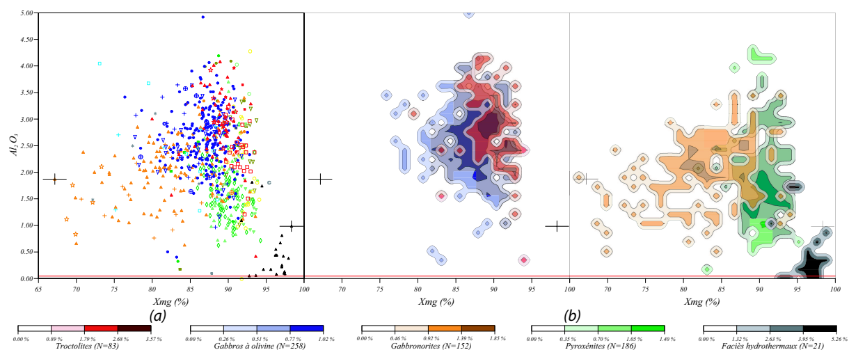
FIG. 3.39 – Diagrammes montrant l'évolution des compositions en aluminium des clinopyroxènes en fonction du Xmg et du type lithologique. (a) : Chaque point représente la composition moyenne pour un échantillon, la légende donnant la signification des symboles est donnée dans le tableau 2.3); (b) : les nuages de densité sont calculés sur l'ensemble des points d'analyse pour chaque famille lithologique.
