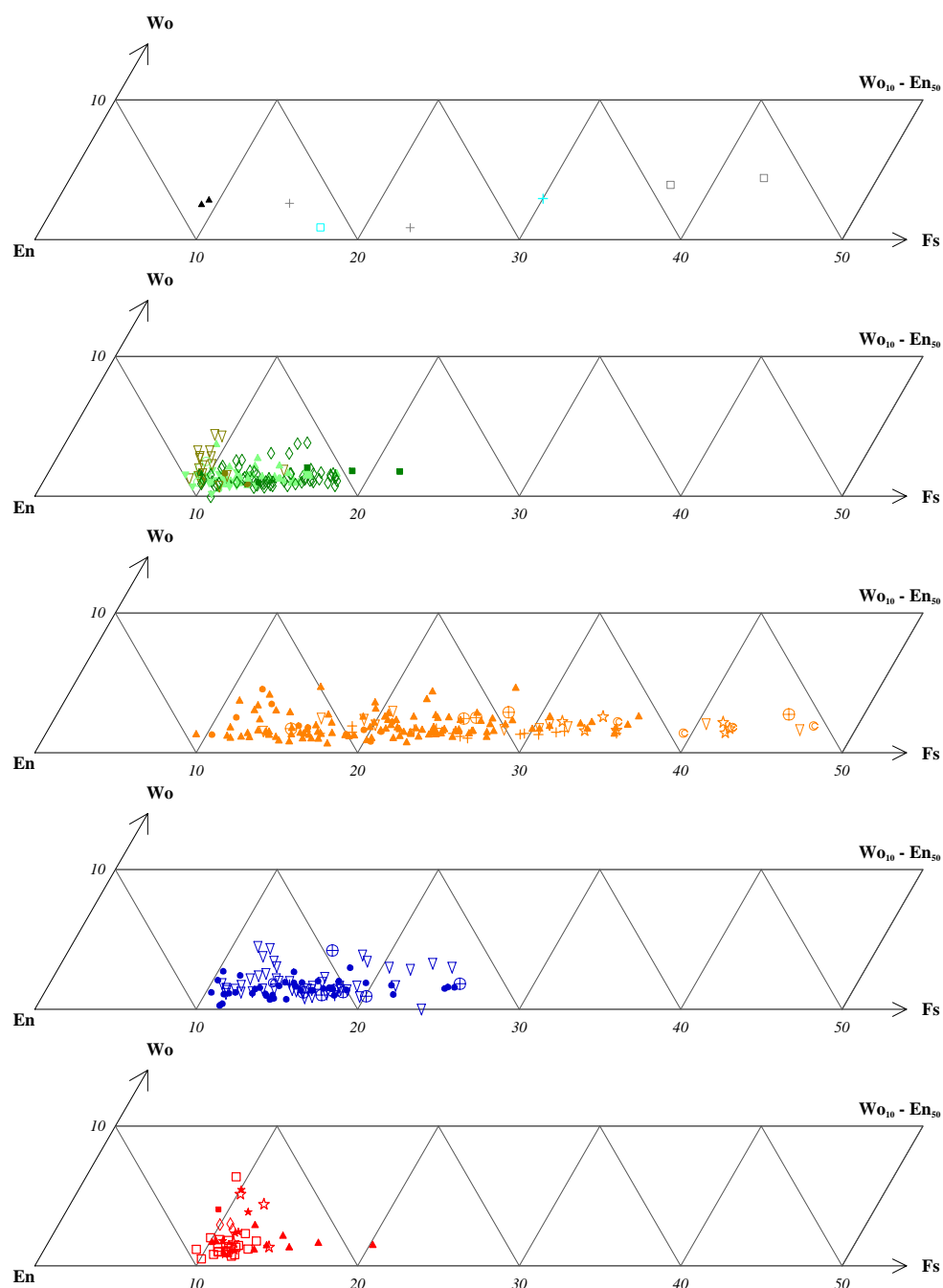
FIG. 3.13 – Détail du triangle En – Wo – Fs donnant les compositions des orthopyroxènes pour chaque famille lithologique (de haut en bas : granits, gabbros indifférenciés et faciès hydrothermaux; famille des pyroxénites; famille des gabbronorites; famille des gabbros à olivine; famille des troctolites).
