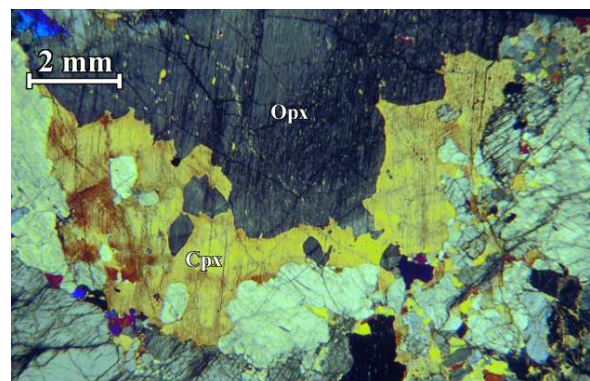
(b) Pegmatite du massif de Sarami, échantillon 00 SA 29
