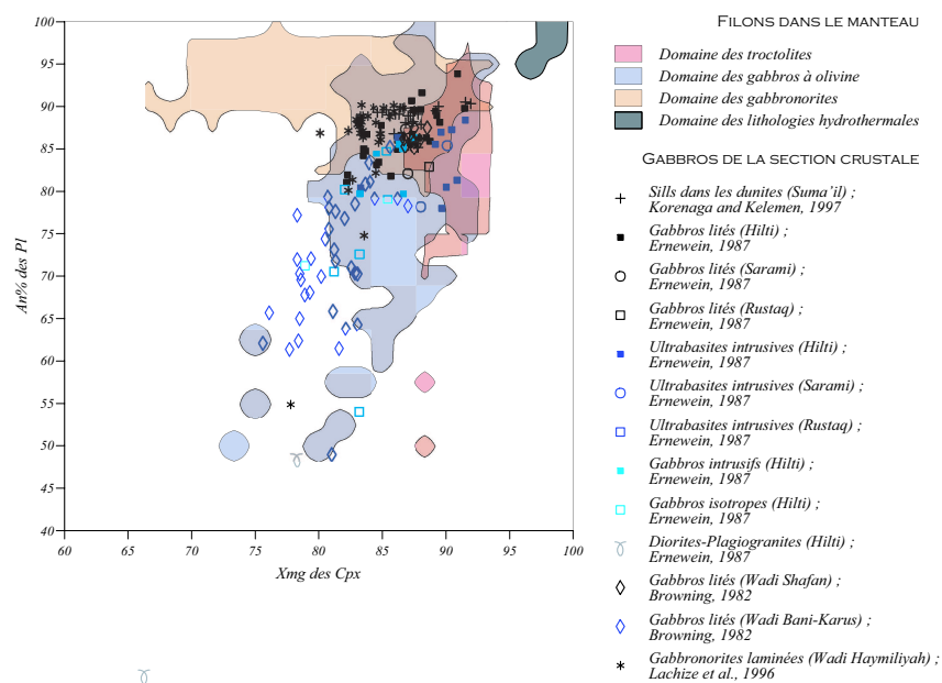
FIG. 4.3 – Teneurs en anorthite des plagioclases en fonction des X_{mg} des clinopyroxènes pour les cumulats de la section crustale d'Oman. Les domaines définis par les différentes familles de cumulats intra-mantelliques apparaissent en fond.
