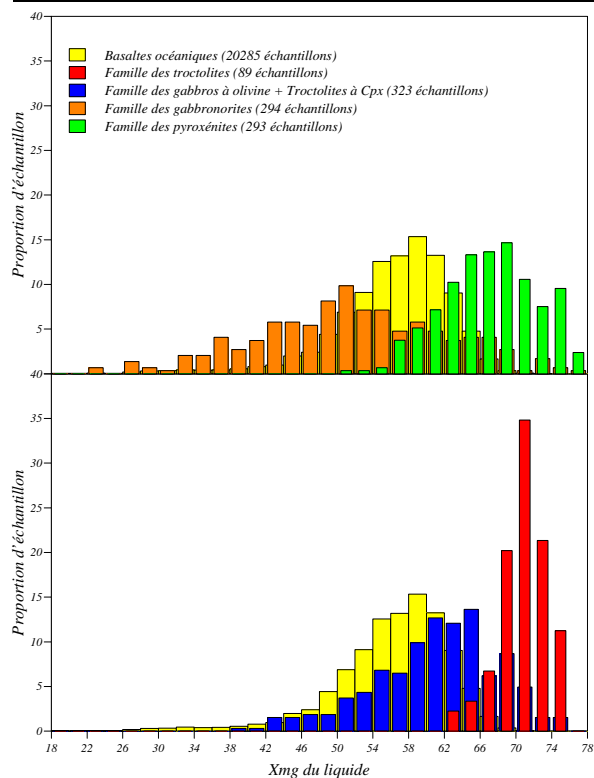
FIG. 4.9 – Histogrammes comparant les X_{mg} obtenus pour les liquides à l'équilibre avec les différentes familles lithologiques filoniennes et les données connues pour 20 285 MORBs. Les troctolites à clinopyroxène sont représentée dans la famille des gabbros à olivine.
