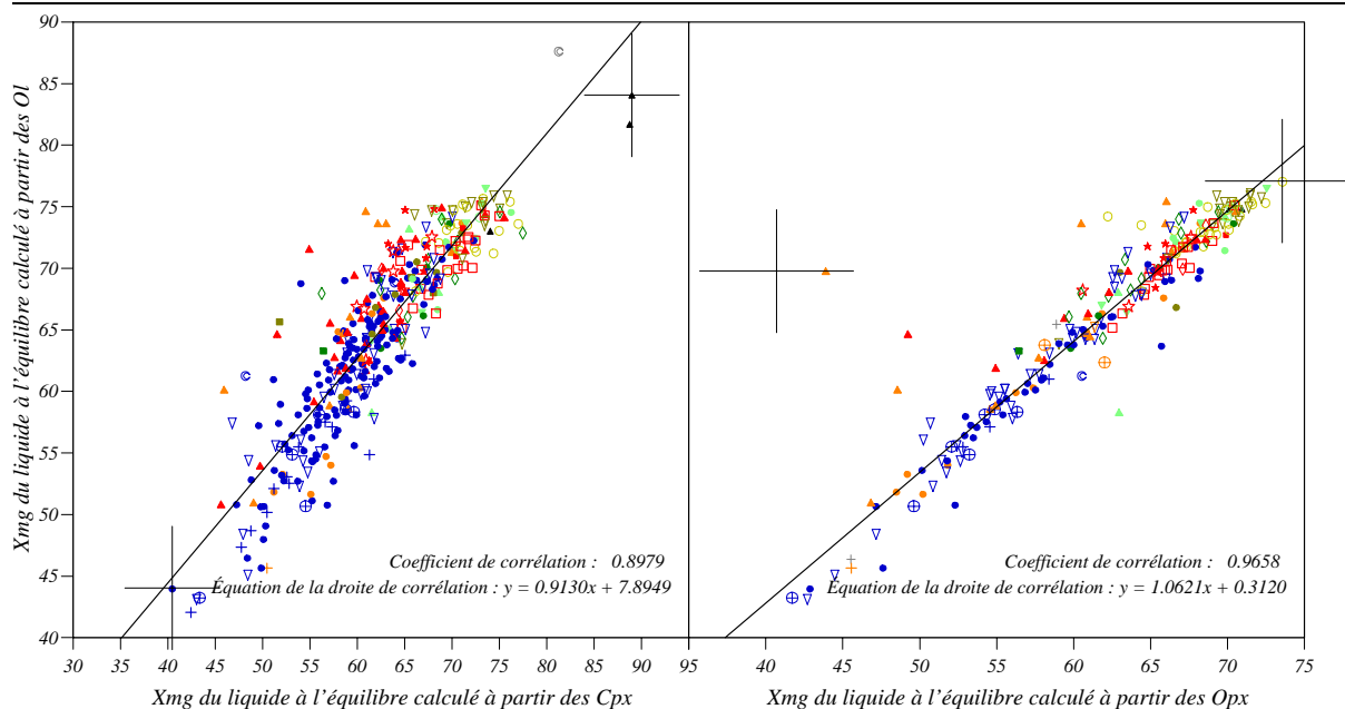
FIG. 4.7 – Graphique montrant les corrélations entre le X_{mg} des liquides à l'équilibre avec les olivines et le X_{mg} des liquides à l'équilibre avec les orthopyroxènes d'un côté, le X_{mg} des liquides à l'équilibre avec les clinopyroxènes de l'autre côté. La droite de corrélation et le coefficient de corrélation ont été calculés par la méthode des moindres carrés, le coefficient de corrélation est fort dans les deux cas et le X_{mg} du liquide à l'équilibre est pratiquement identique lorsqu'il est calculé à partir des olivines ou à partir des orthopyroxènes. Une légère dérive existe entre les calculs avec les olivines et les calculs avec les clinopyroxènes, elle peut être " corrigée " grâce à la corrélation observée.
