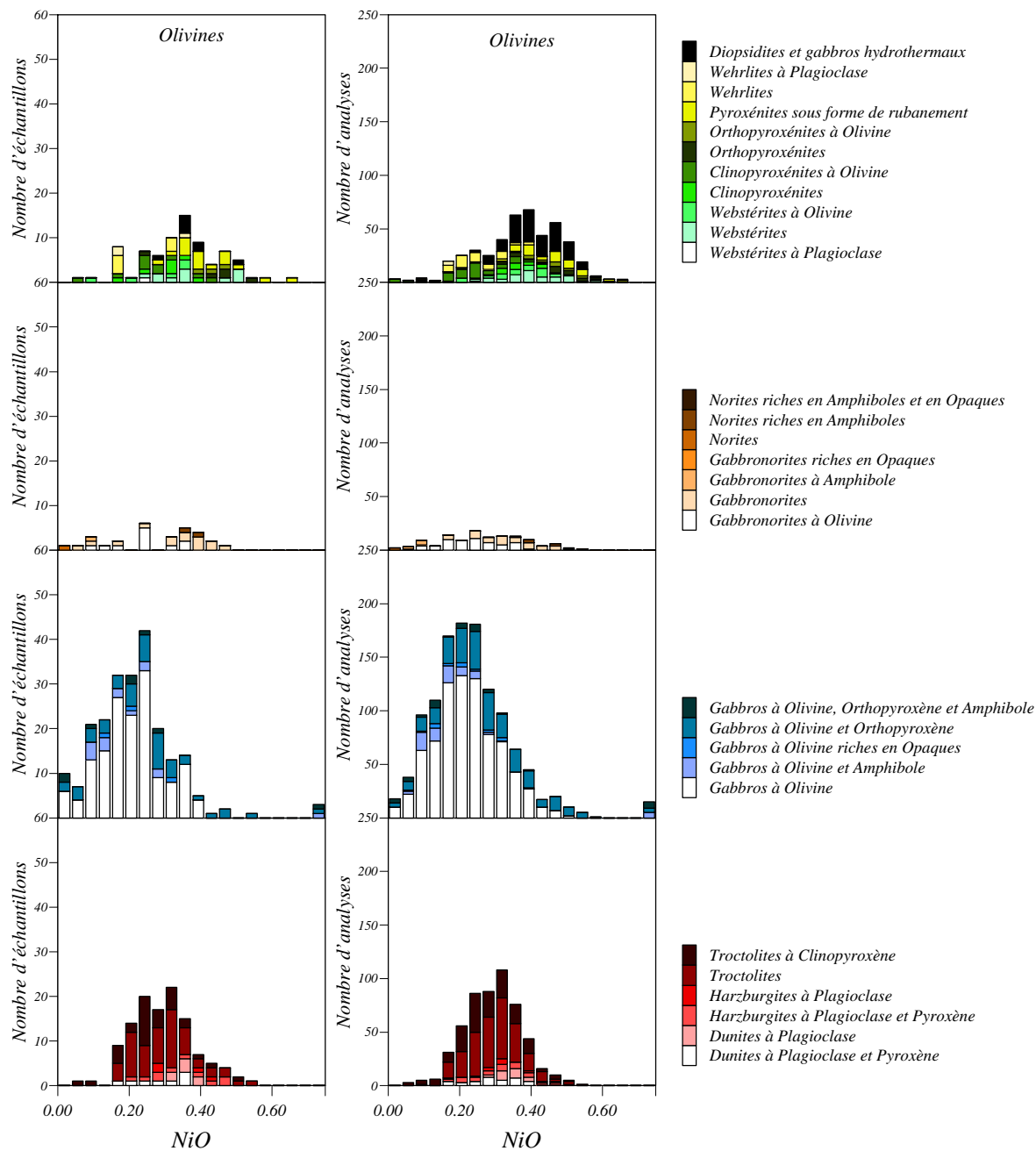
FIG. 3.7 – Histogrammes des teneurs en nickel des olivines analysées pour tous les faciès contenant ce minéral.
