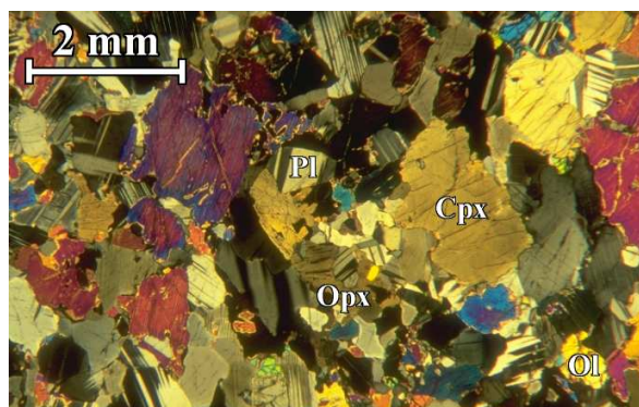
(a) Gabbrorite sans hornblende, échantillon 01 MB 6
