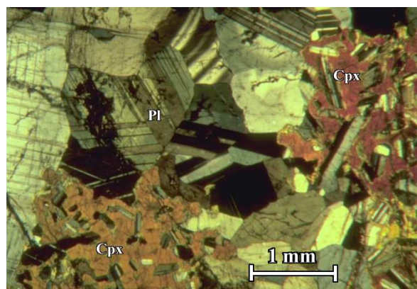
FIG. 2.6 – Texture partiellement recrystallisée d’une harzburgite à plagioclase, le clinopyroxène garde son caractère poecilitiques (massif de Hiliti, échantillon 99 HI 71c). Lumière polarisée, nicols croisés.
