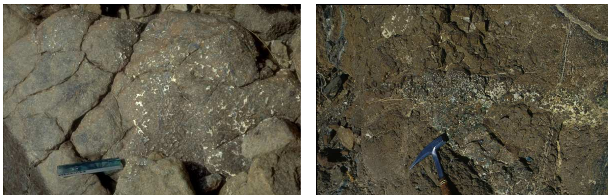
(a) Imprégnation diffuse dans la dunite du massif de Suma'il
