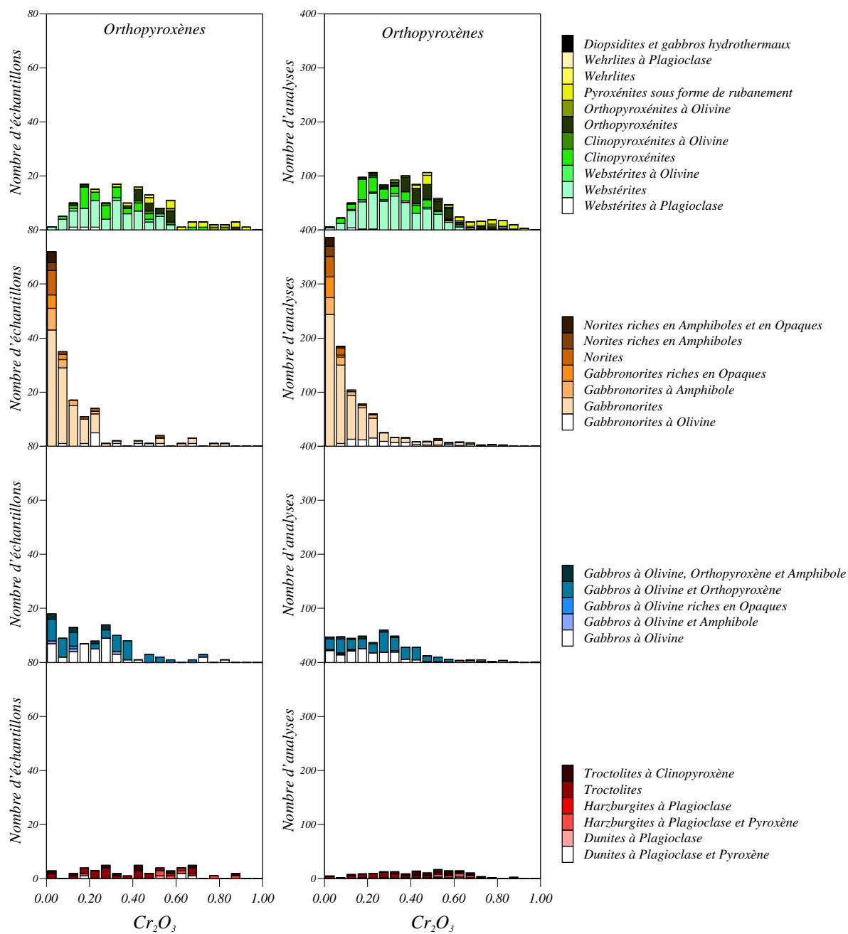
FIG. 3.17 – Histogrammes des teneurs en chrome des orthopyroxènes analysés pour tous les faciès contenant ce minéral.
