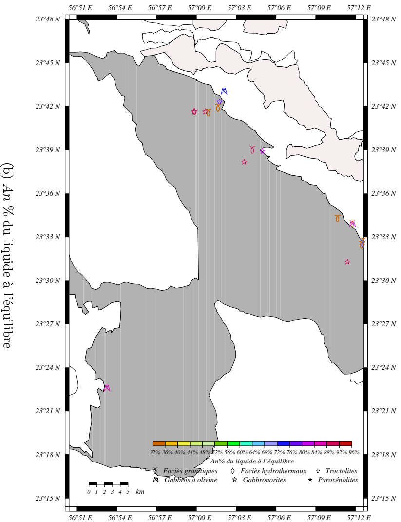
FIG. A.31 – Cartes géologiques d'une partie du massif de Rustaq et de l'extrémité est du massif de Wujbah montrant les répartitions pour le X_{mg} et le An\% des liquides à l'équilibre.
