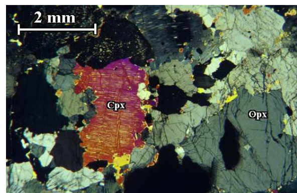
(b) Échantillon 00 FZ 3
