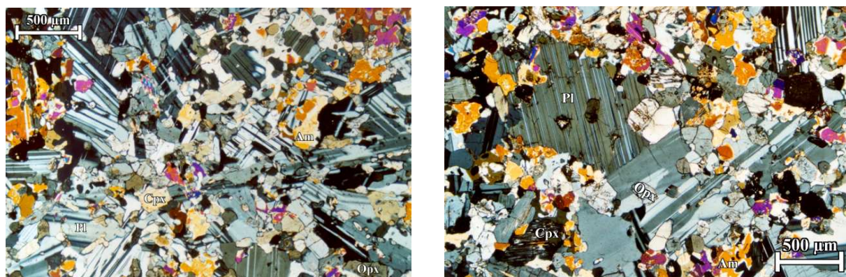
FIG. 2.70 – Deux lames minces d'un même échantillon de gabbro-norite à amphibole à texture de mésocumulus, le plagioclase apparaît en plage pœcilitique autour d'orthopyroxènes et de clinopyroxènes sub-automorphes (échantillon 00 NA 50). Lumière polarisée, nicols croisés.
