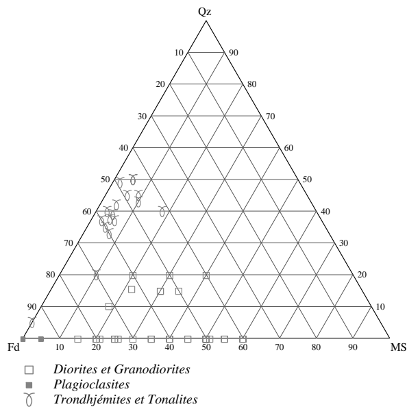
FIG. 2.134 – Diagramme triphasé Quartz (Qz) – Feldspaths (Fd) – Minéraux sombres (MS, amphiboles, opaques et biotites) représentant les composition modales des trondhjemites, diorites et granodiorites.
