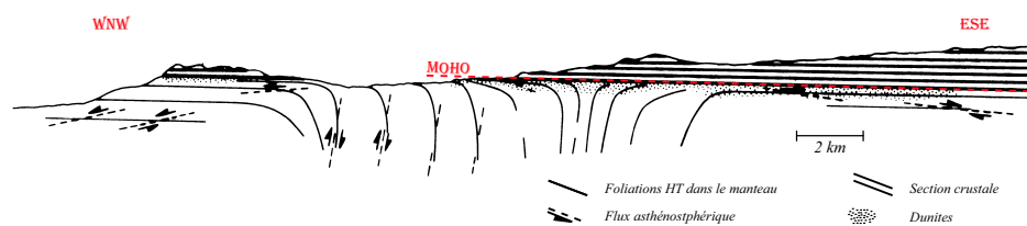
FIG. 1.11 – Coupe ouest-nord-ouest à est-sud-est dans le diapir de Maqsad parallèle à l'axe de la paléo-dorsale, cette coupe illustre la rotation rapide des structures mantellaires à l'aplomb du diapir (modifié d'après Ceuleneer et al., 1988 ; Nicolas, 1989)
