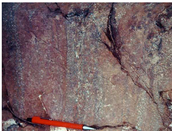
(a) Lentilles diffuses, massif de Suma'il (Amri, 1995)
