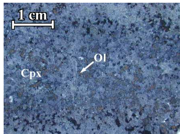
FIG. 2.84 – Face sciée d'un échantillon de clinopyroxénite à olivine à grains fins (massif du Wadi-Tayin, échantillon 00 WT 31 ).
