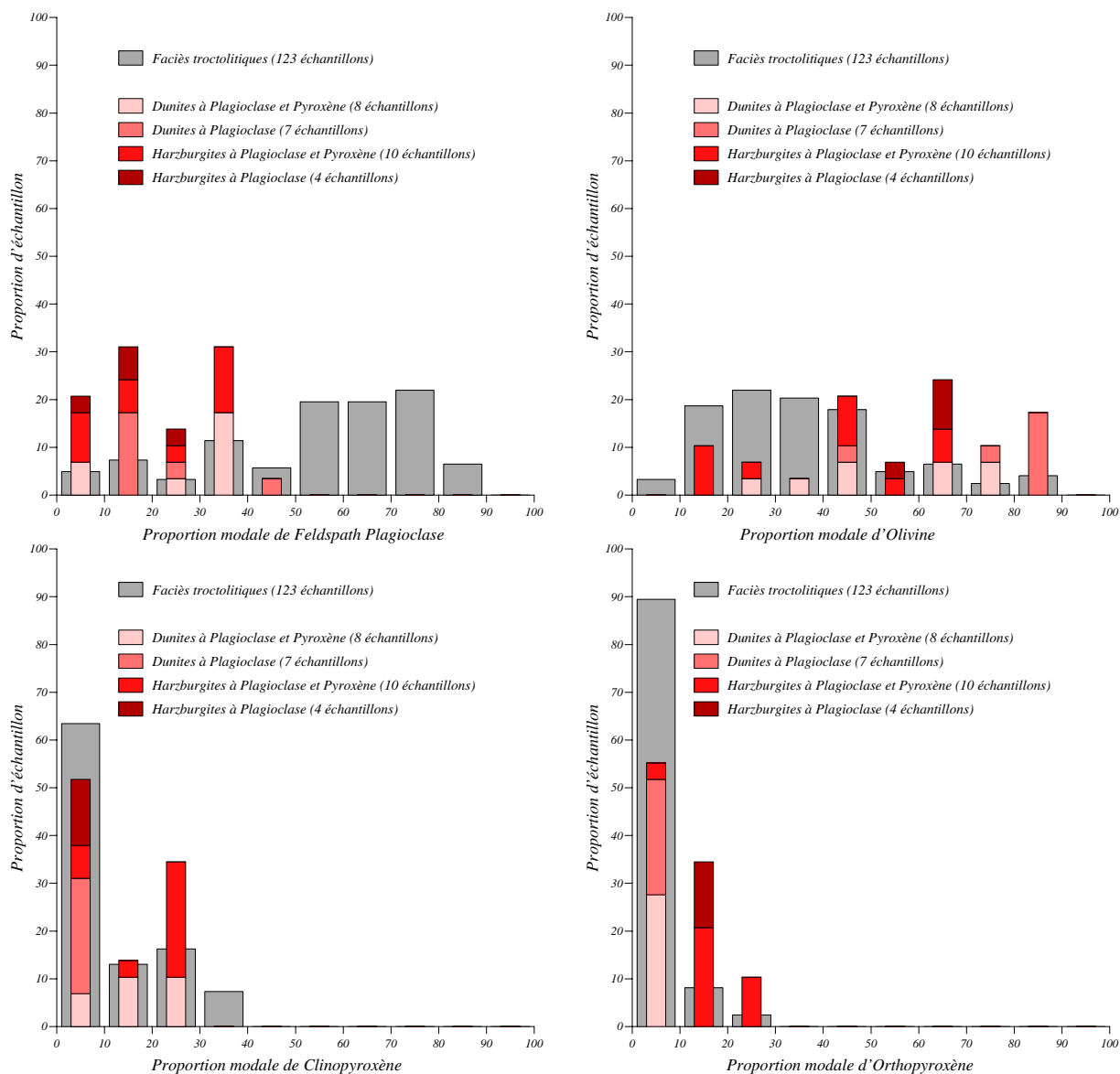
FIG. 2.8 – Histogrammes montrant les fréquences de pourcentage en plagioclases, olivines, clinopyroxènes et orthopyroxènes dans les faciès d'imprégnation (en rouge). En gris, pour comparaison, sont représentés l'ensemble des faciès troctolitiques (harzburgites et dunites à plagioclase et/ou clinopyroxène, troctolites et troctolites à clinopyroxène).
