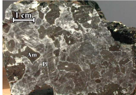
(b) Massif de Nakhl, échantillon 00 NA 53
