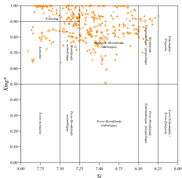
(b) Famille des gabbronorites
