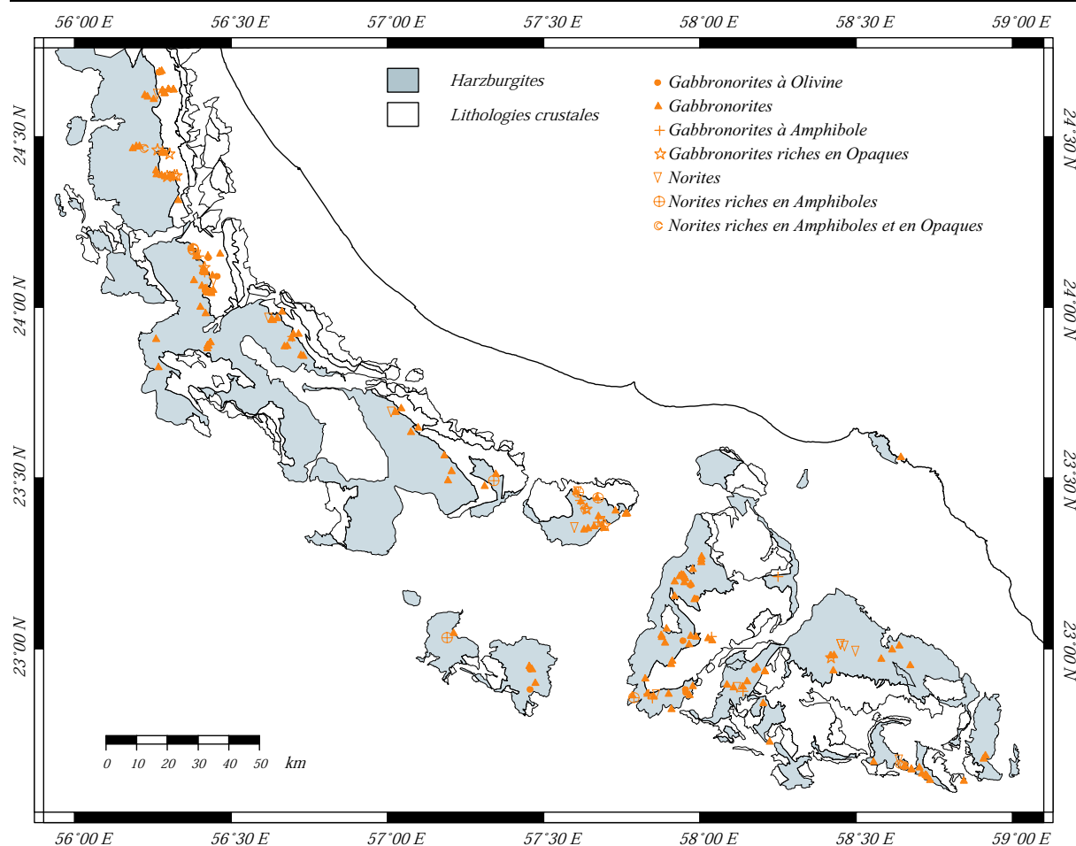
FIG. 3.52 – Carte géologique générale de l'ophiolite d'Oman où sont placés les échantillons de gabbronorite : gabbronorites et norites. Les contours géologiques dessinés ont été digitalisés à partir des cartes du B.R.G.M. au 250 000 ème .
