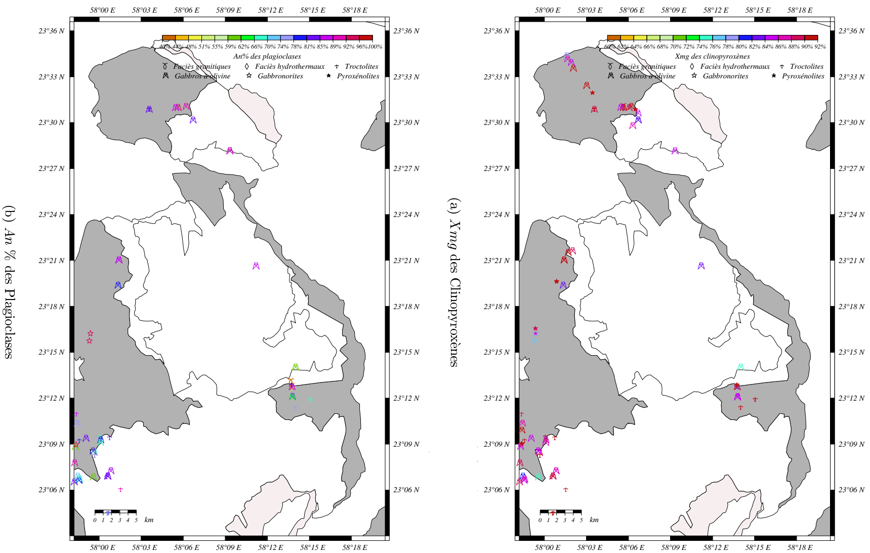
Fig. A.22 – Cartes géologiques des massifs de Kahwad et Musibit montrant les répartitions des Xmg des clinopyroxènes et des An % des plagioclases.
