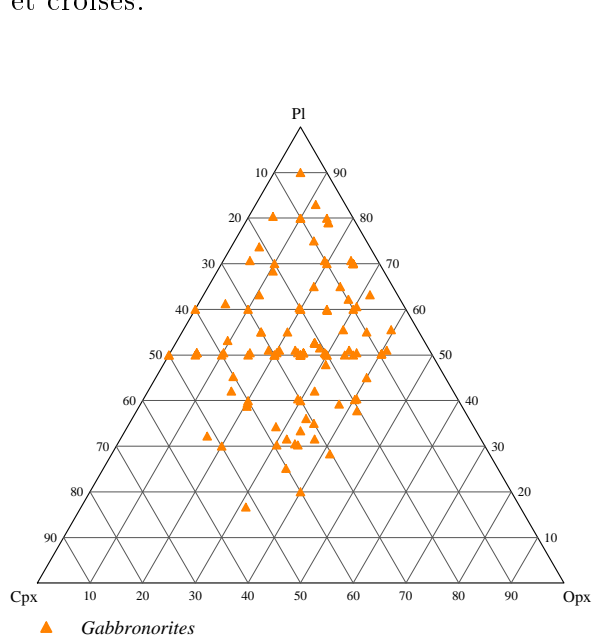
FIG. 2.74 – Diagramme représentant les compositions modales des gabbroites dont l'orthopyroxène est une phase précoce dans le système ternaire plagioclase (Pl) – clinopyroxène (Cpx) – orthopyroxène (Opx).
