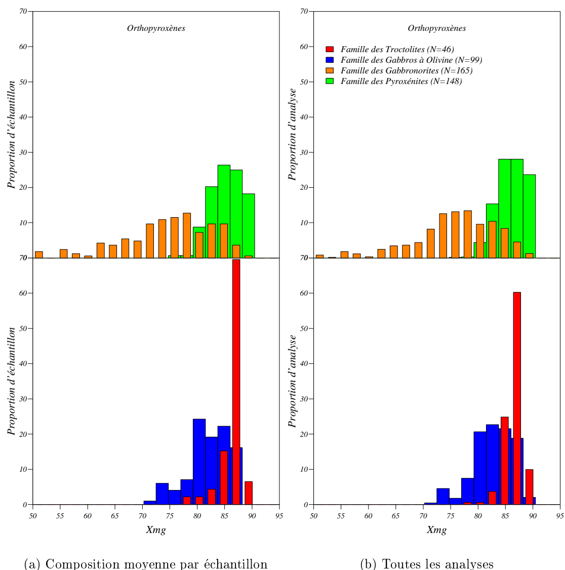
FIG. 3.14 – Histogrammes donnant les proportions d'échantillons (a) et d'analyses (b) de chaque famille de faciès pour un intervalle donné du X_{mg} = 100 \frac{Fe^e}{Fe^e + Mg} des orthopyroxènes analysés.
