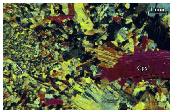
FIG. 2.143 – Lame de diopsidite montrant la variation de la texture : les gros grains en fibres semblent de déstabiliser et subir une recristallisation sur les bordures (massif de Haylayn, échantillon 00 RU 21). Lumière transmise polarisée, nicols croisés.
