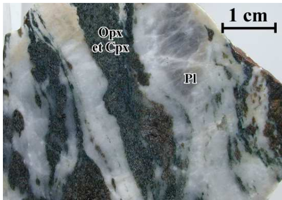
(a) Massif de Fizh, échantillon 00 FZ 25
