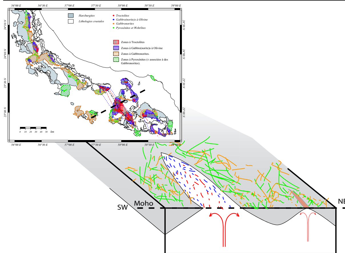
FIG. 4.14 – Coupe schématique à travers les massifs de Suma'il et Musibit montrant l'évolution possible d'un diapir du manteau. En gris (sur la coupe) est représentée la lithosphère ; en blanc, l'asthénosphère. Ce schéma résume le processus proposé en figure 1.14, le massif de Suma'il représenterait un stade développé du diapir (étape (c) dans la figure 1.14) tandis que les massifs de Hilti et la bande parallèle de Kahwad, Musibit et Wadi-Tayin correspondraient à un stade plus précoce (étape (b) dans la figure 1.14)
