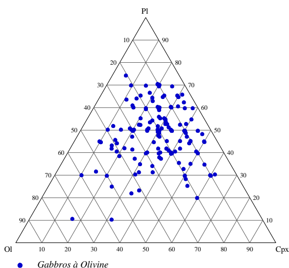
FIG. 2.35 – Diagramme représentant les compositions modales des gabbros à olivine dans le système plagioclase (Pl) - olivine (Ol) - clinopyroxène (Cpx).
