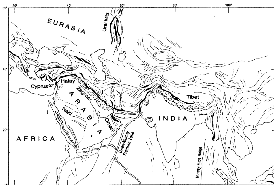
FIG. 1.2 – Carte structurale générale d'une partie de la chaîne plissée Alpino-Himalayenne montrant la localisation de la plaque Arabe et la répartition des ophiolites le long de la suture Alpine (extrait de Coleman, 1981).
