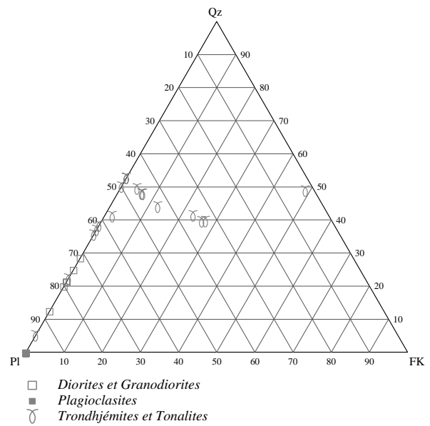
FIG. 2.135 – Diagramme triphasé Quartz (Qz) – PLAGioclases (Pl) – Feldspaths potassiques (FK) représentant les composition modales des trondhjemites, diorites et granodiorites.
