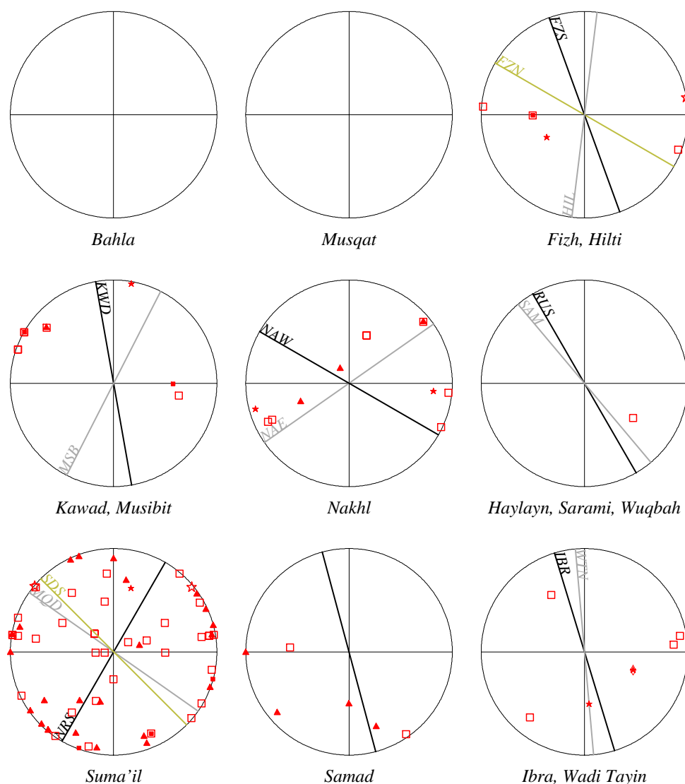
FIG. 2.12 – Projections stéréographiques montrant les orientations des faciès troctoliques en fonction des zones géographiques. Pour comparaison, l'orientation moyenne du complexe filonien pour les différentes régions est donnée sur chaque stéréogramme et est référencée comme suit : FZS : massif de Fizh sud (Ceuleneer, 1986) ; FZN : massif de Fizh nord (Smewing, 1980a; Reuber, 1988; MacLeod and Rothery, 1992) ; HIL : massif de Hilti (Ceuleneer, 1986) ; KWD : massif de Kahwad (Misseri, 1982) ; MSB : massif de Musibit (Misseri, 1982) ; NAW : massif de Nakhl ouest (Browning, 1982; Ceuleneer, 1986) ; NAE : massif de Nakhl est (MacLeod and Yaouancq, 2000) ; SAM : massif de Sarami (Ceuleneer, 1986) ; RUS : massifs de Haylayn et Wuqbah (Pallister, 1981; Browning, 1982; Dahl, 1984; Ceuleneer, 1986) ; SDS : massif de Suma'il sud (Misseri, 1982) ; NRS : massif de Suma'il nord (Misseri, 1982; Ceuleneer, 1986) ; MQD : massif de Suma'il, région de Maq-sad (Ceuleneer, 1986; MacLeod and Rothery, 1992; Nicolas and Boudier, 1995; Jous-selin et al., 1998) ; IBR : massif d'Ibra (Pallister, 1981; Misseri, 1982) ; WTN : massif du Wadi Tayin (Misseri, 1982; Ceuleneer, 1986). Pour le massif de Samad, voir Ceuleneer, 1986 et Misseri, 1982. Voir tableau 2.3 pour la légende des symboles.
