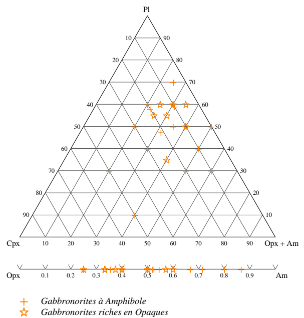
FIG. 2.75 – Diagramme représentant les compositions modales des gabbroites à hornblende et/ou à oxyde dont l'orthopyroxène est une phase précoce dans le système plagioclase (Pl) – clinopyroxène (Cpx) – orthopyroxène + amphibole (Opx + Hb).
