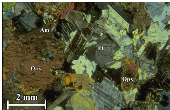
FIG. 2.153 – Échantillon de norite contenant de l'amphibole se développant en couronne autour des orthopyroxènes (échantillon 00 NA 43). Lumière polarisée, nicols croisés.
