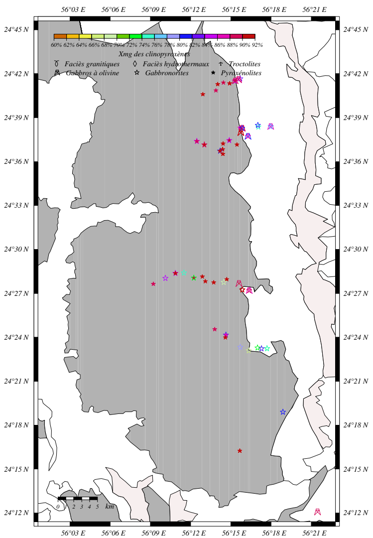
(a) Xmg des Clinopyroxènes
