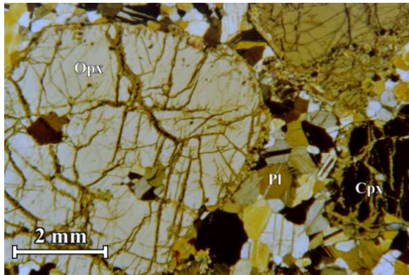
FIG. 2.67 – Échantillon de gabbro partiellement recristallisé dans le plagioclase, cet échantillon est sans doute une ancienne pegmatite qui a subi une déformation assez poussée à une température suffisamment élevée pour permettre la recristallisation (massif de Sumail, échantillon 90 OG 131c). Lumière polarisée, nicols croisés.
