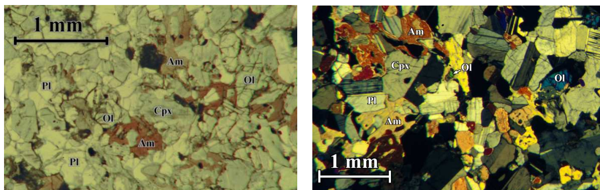
(a) échantillon 00 NA 63 (massif de Nakhl), nicols parallèles
