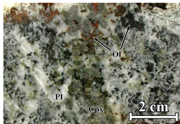
(b) Surface sciée
