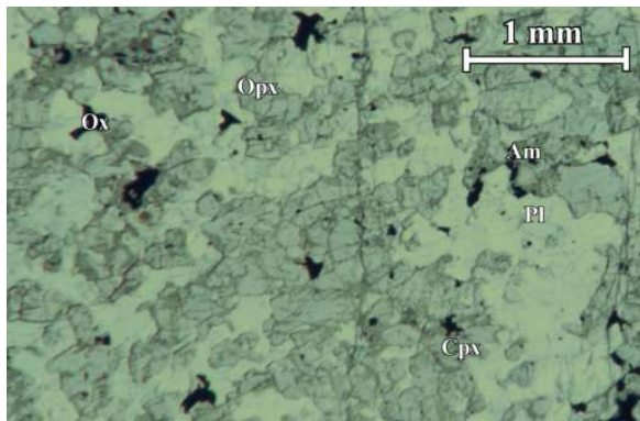
(a) Nicols parallèles
