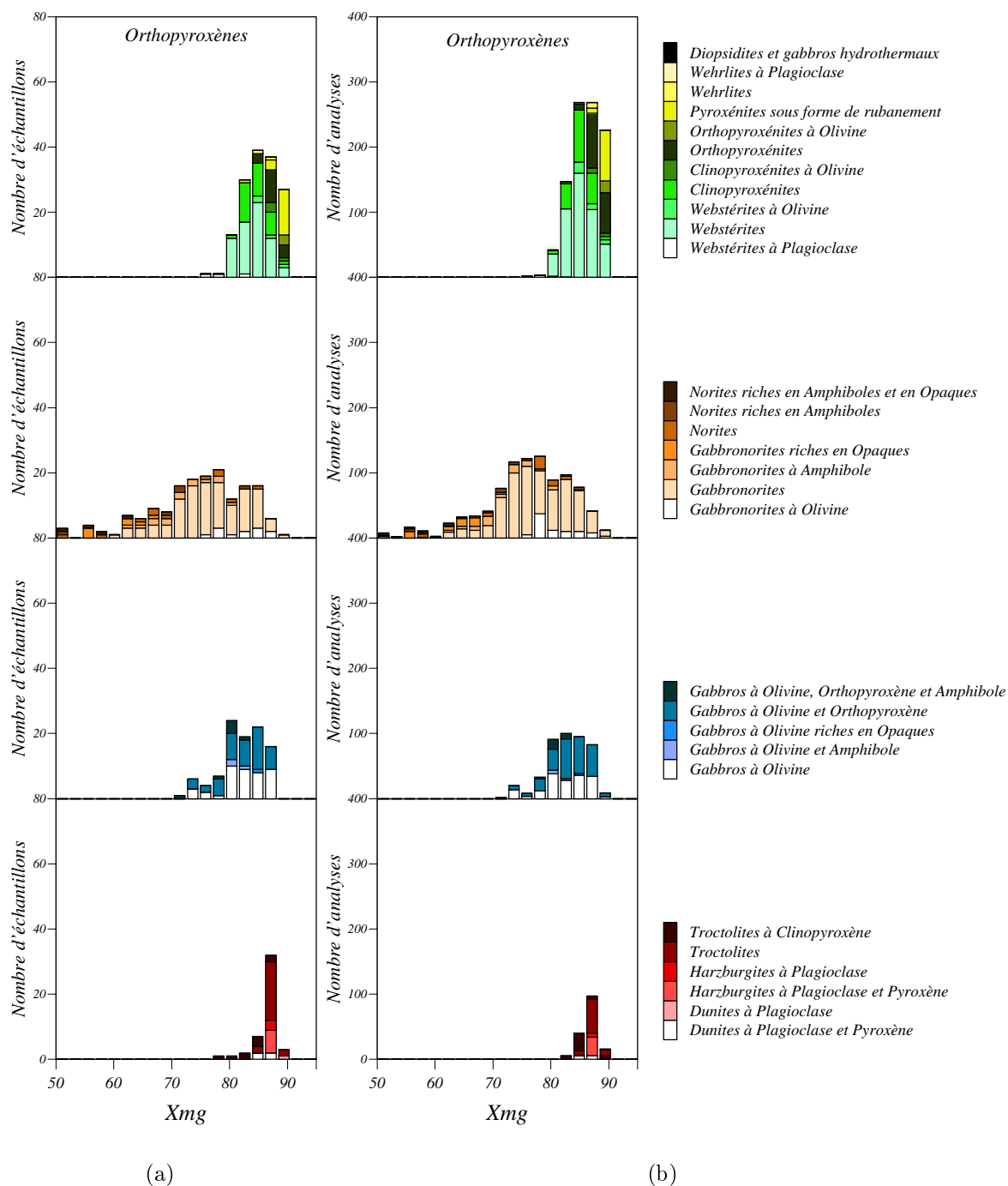
FIG. 3.15 – Histogrammes donnant les nombres d'échantillons (a) et d'analyses (b) pour chacun des types lithologiques définis et pour un intervalle donné du X_{mg} = 100 \frac{Fe}{Fe+Mg} des orthopyroxènes.
