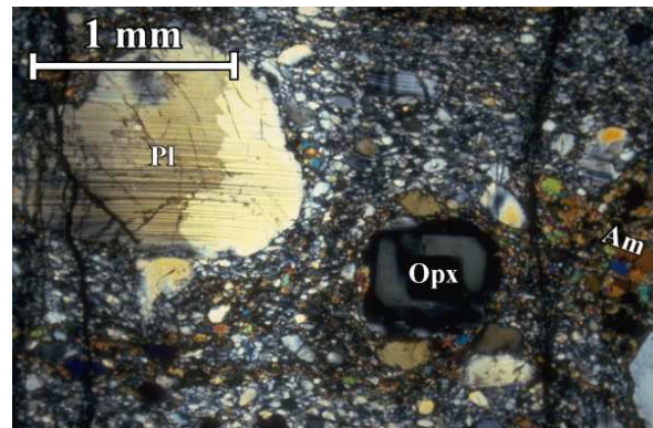
(b) Gabbro à amphibole du massif de Hilti, échantillon 99 HI 76
