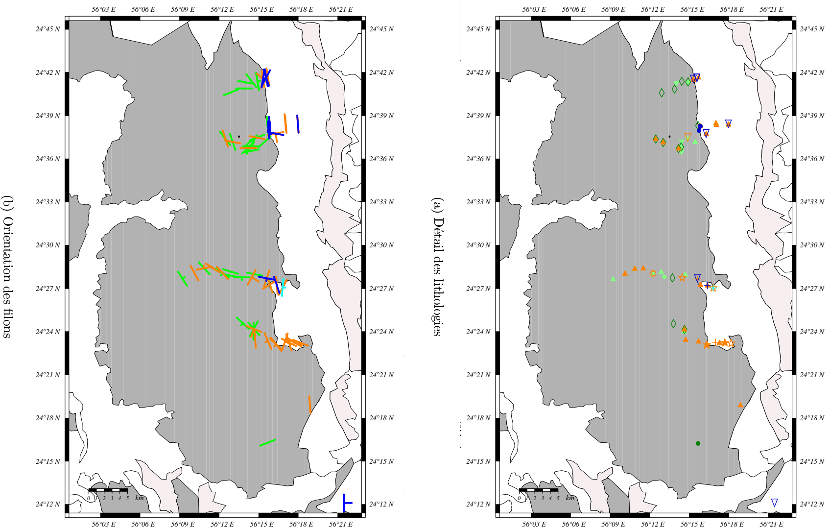
FIG. A.1 – Cartes géologiques du massif de Fizi montrant la localisation des diverses familles lithologiques et leurs orientations.
