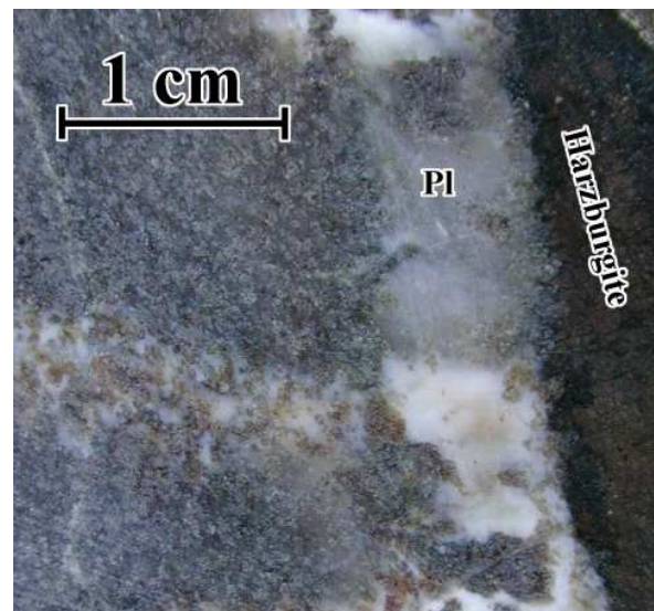
FIG. 2.61 – Exemple d'échantillon de gabbro-rite à grains fins avec croissance harzburgitique des cristaux aux épontes (massif de Fizh, échantillon 00 FZ 40b).
