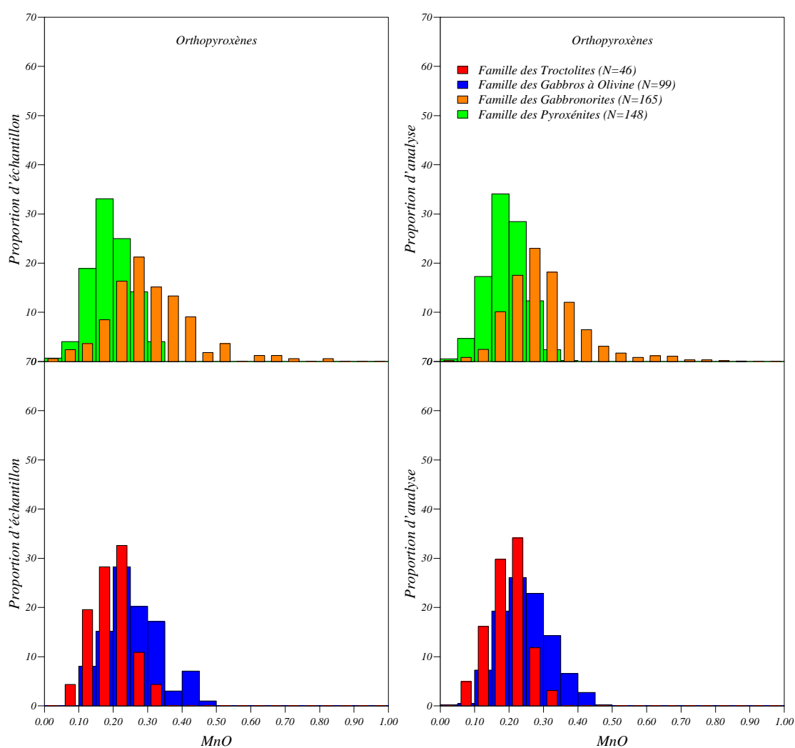
(a) Composition moyenne par échantillon
