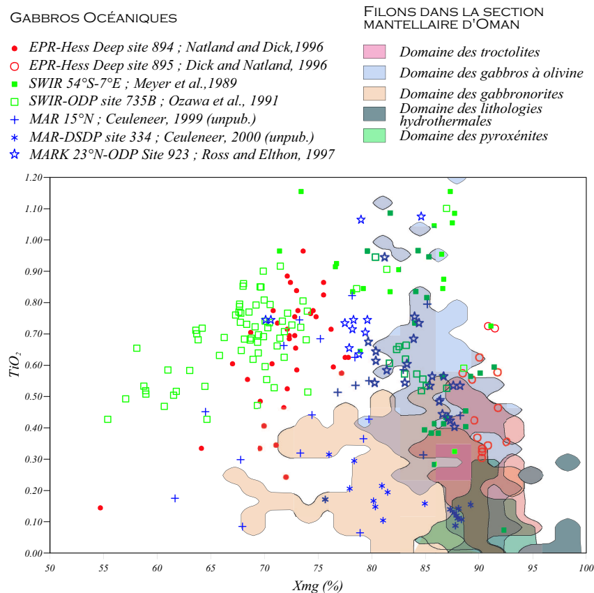
FIG. 4.6 – Teneur en titane des clinopyroxènes en fonction de leurs X_{mg} pour les gabbros océaniques ; les domaines de chimie des lithologies filoniennes d'Oman apparaissent en fond.
