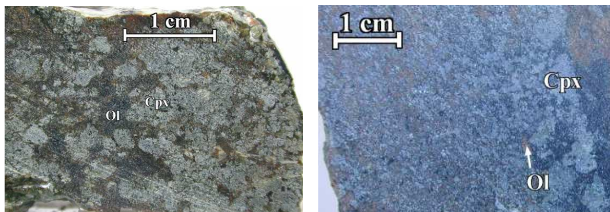
(a) Échantillon 00 FZ 40c , massif de Fizh
