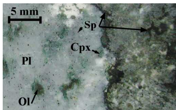
FIG. 2.29 – Échantillon de gabbro à olivine contenant plus de 15 % de spinelle (massif de Haylayn, échantillon 00 RU 23b ).
