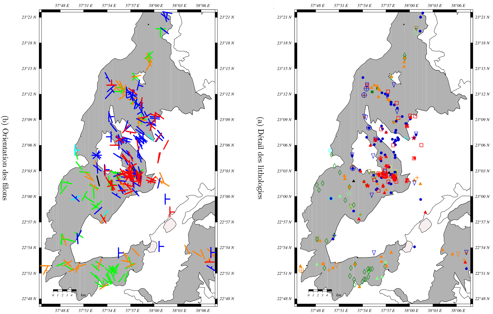
FIG. A.10 – Cartes géologiques du massif de Suma'il montrant la localisation des diverses familles lithologiques et leurs orientations.
