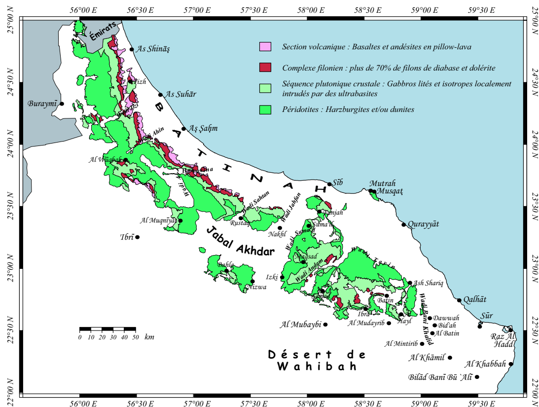
FIG. 1.10 – Carte géologique simplifiée de la séquence ophiolitique des nappes d’Oman localisant les principales villes et wadis (contours géologiques digitalisés d’après les cartes géologiques de l’ophiolite d’Oman du BRGM au 250 000 ème ).
