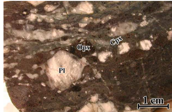
(b) Massif de Hilti, échantillon de gabbro- rite à amphibole 99 HI 76
