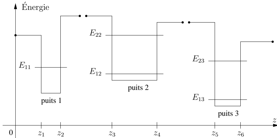
FIG. 3.2 – Bande de conduction faisant apparaître plusieurs puits quantiques; les états E_{ij} sont les états calculés dans chacun des puits découplé des autres
