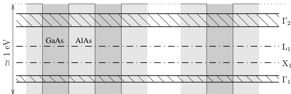
FIG. 7.3 – Diagramme de bande d'un super-réseau constitué de GaAs et d'AlAs
