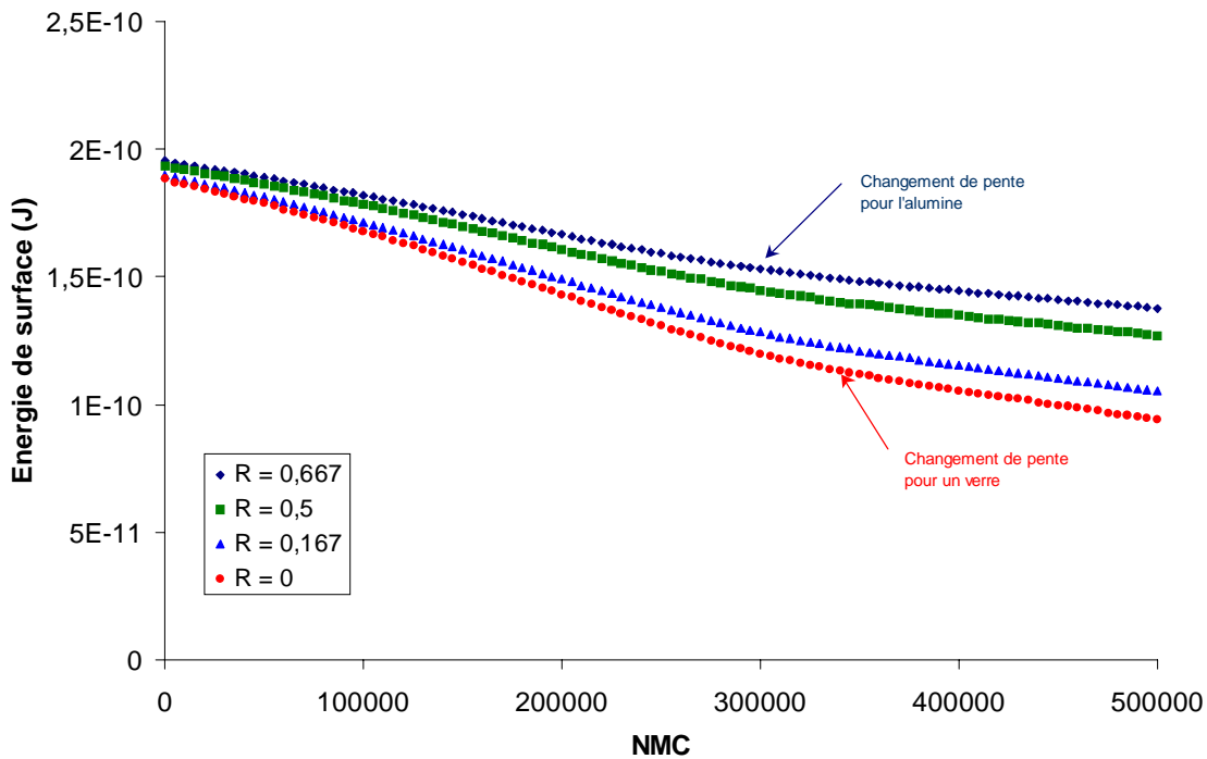
Figure V-14 : Evolution de l'énergie de surface en fonction du nombre de boucles Monte Carlo pour différents rapports de tension de surface R . Le changement de pente correspond au changement de régime des flux.
