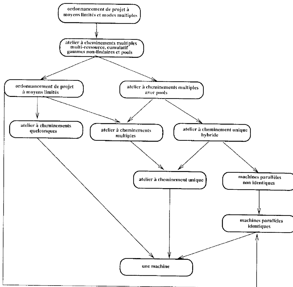
FIG. I.2 – Hiérarchie des modèles
