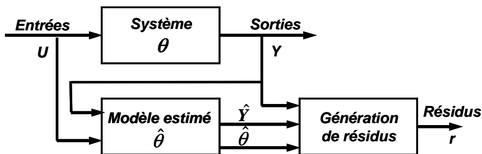
Figure 1.2. Principe de génération des résidus
