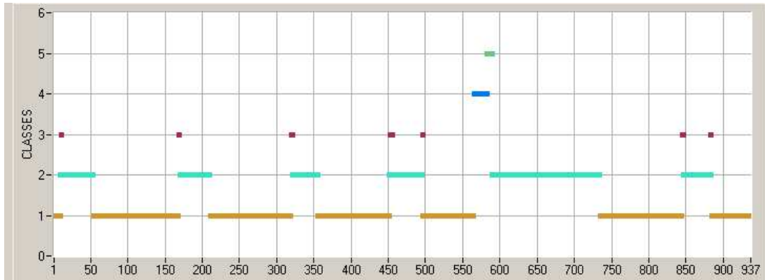
a) Classes générées pour le bouilleur en régime normal (données brutes)
