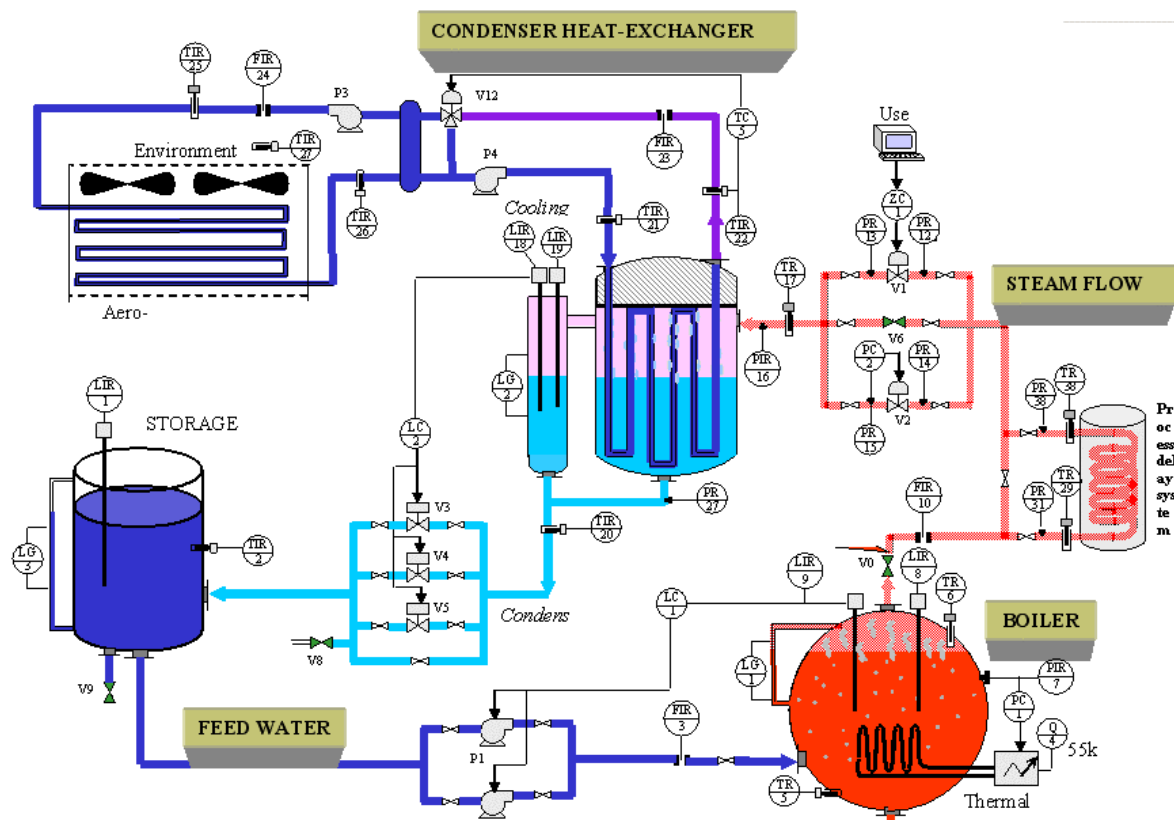
Figure 5.13. Schéma général de l'installation
