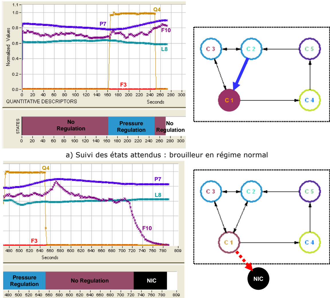
a) Suivi des états attendus : brouilleur en régime normal b) Détection d'une déviation : observations non reconnues Figure 5.18. Identification en ligne des états du brouilleur
