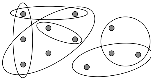
FIG. A.9 – Exemple d'hypergraphe.
