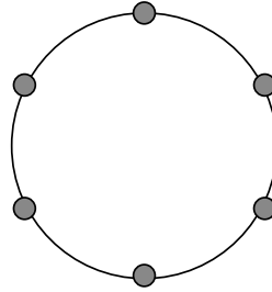
FIG. 1.7 – L'ensemble des sommets du cycle forme un code (1, \leq 2) -identifiant du cycle.
