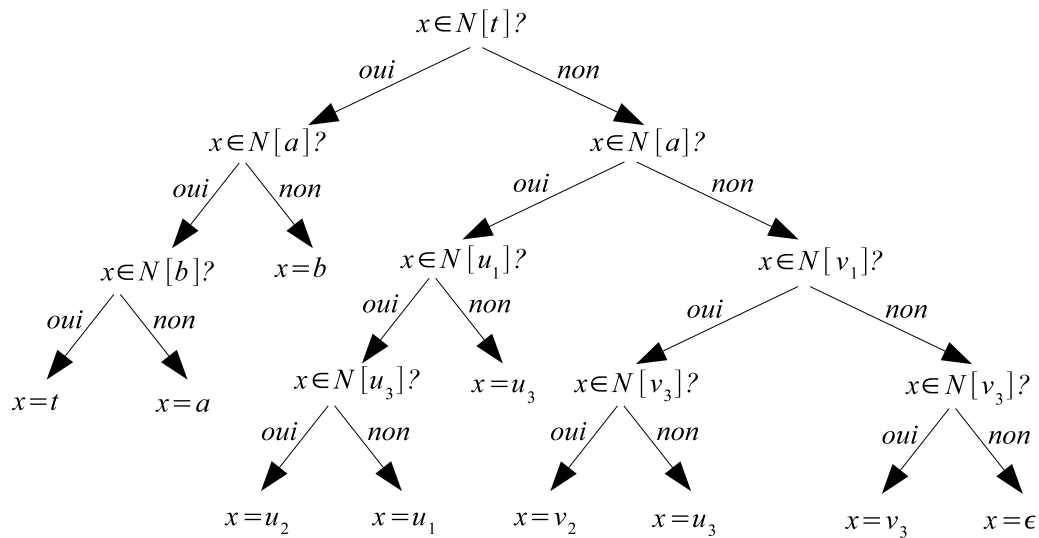
FIG. 1.16 – Exemple de stratégie adaptative dans le cas déterministe : nous pouvons concevoir une stratégie adaptative nécessitant au plus quatre questions, alors que la cardinalité minimum d'un code identifiant du graphe considéré est cinq.
