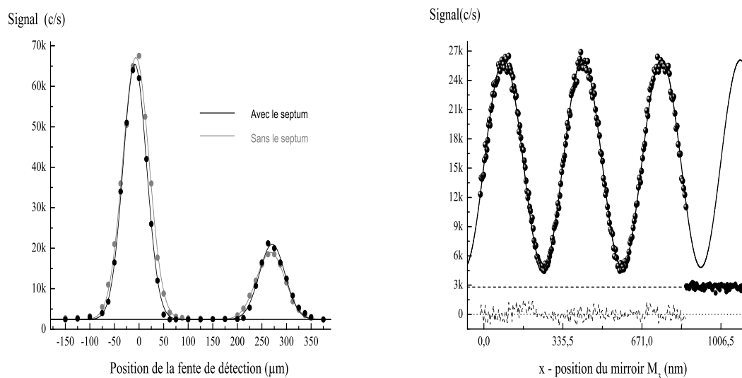
FIG. 6.13 – A gauche : Profils de diffraction de l'onde atomique au premier ordre par la première onde laser stationnaire. La courbe noire (resp. grise) correspond au cas où les deux chemins sont situés de part et d'autre du septum (resp. du même côté du septum). A droite : Franges d'interférence atomique en présence du septum : la visibilité atteint 84 \pm 1\% .
