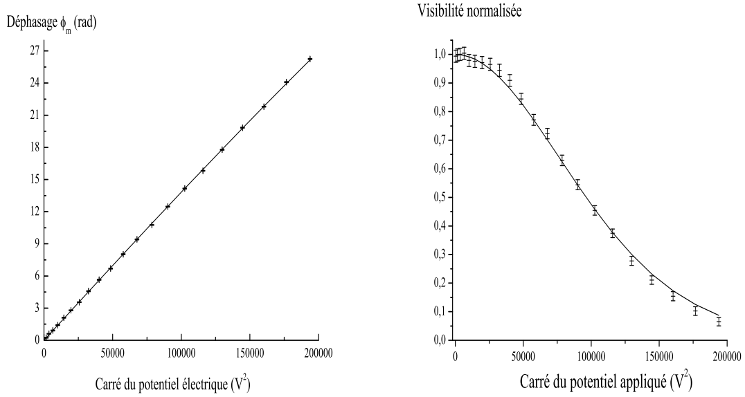
FIG. 6.19 – Déphasage et visibilité des franges atomiques en fonction du carré du potentiel V_0 appliqué : les points sont expérimentaux et les courbes représentent le meilleur ajustement.
