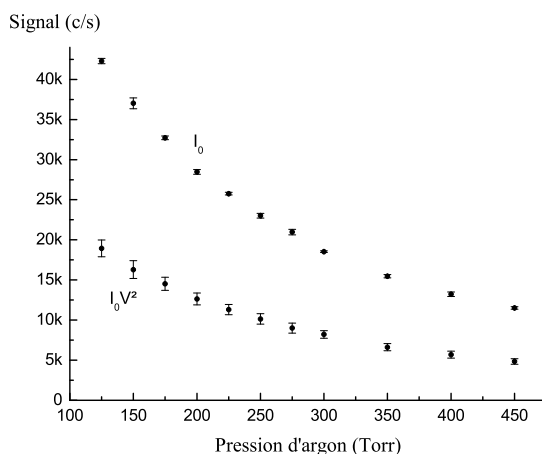
FIG. 4.22 – Flux moyen I_0 en sortie de l'interféromètre et facteur de mérite I_0 \mathcal{V}^2 pour différentes pressions d'argon. La meilleure sensibilité en phase est obtenue pour la pression d'argon la plus faible. En pratique une pression de 125 Torr semble la plus appropriée.
