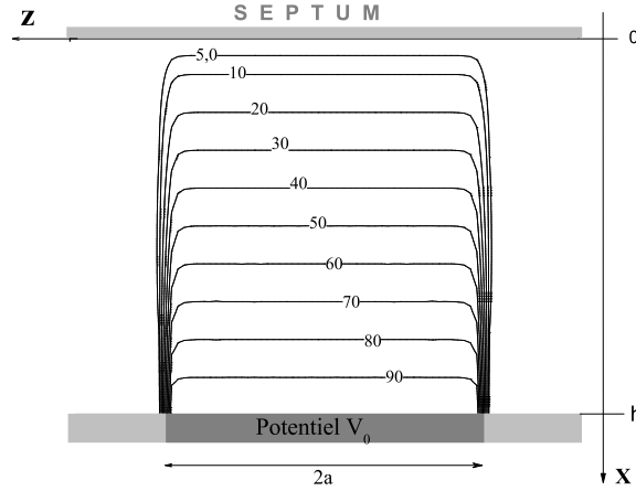
FIG. 6.6 – Courbes équipotentiellles dans le condensateur. Le potentiel est nul partout sauf dans l'interface entre l'électrode de potentiel V_0 et la feuille qui sépare les deux chemins atomiques. Dans cette zone, son intensité est exprimée en pourcentage de l'intensité du potentiel V_0 .
