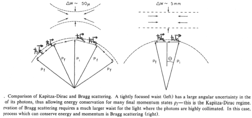
FIG. 2 – Schéma tiré de l'article [38] illustrant les deux régimes de diffraction d'une onde atomique par une onde stationnaire laser quasi-résonante: à gauche, le régime de Kapitza - Dirac, à droite le régime de Bragg, \hbar\mathbf{k}_L désignant l'impulsion du photon.
