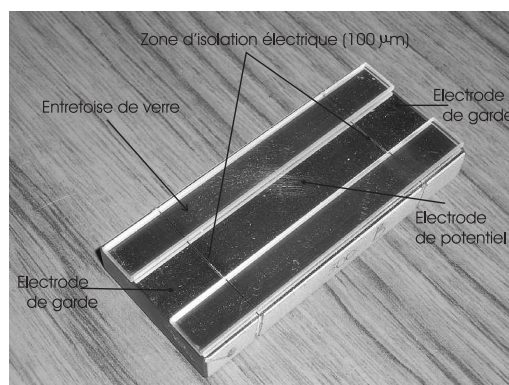
FIG. 6.8 – Photographie de l'électrode de potentiel et des deux électrodes de garde situées à l'entrée et à la sortie du condensateur. L'isolation électrique est assurée par deux zones de 100 \mu m de large obtenues par évaporation laser.
