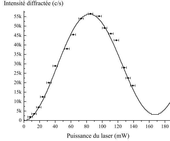
FIG. 3.6 – Intensité d'atomes diffractés en fonction de la puissance du laser au premier ordre de diffraction pour un jet atomique pompé optiquement dans un seul niveau hyperfin F = 2 .
