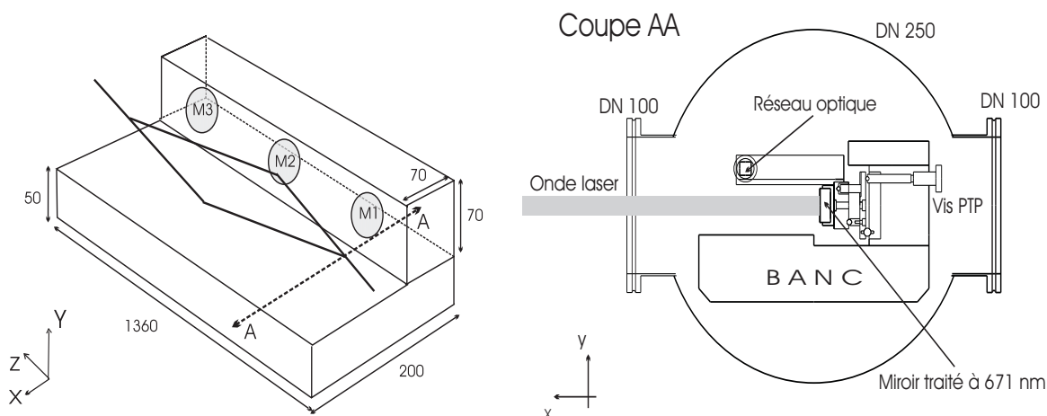
FIG. 1.7 – Schéma du banc avec les trois miroirs servant à la réalisation des ondes stationnaires laser. Dans la vue en perspective, on a volontairement exagéré la séparation des deux chemins atomiques pour améliorer la visibilité du dessin. Les distances sont exprimées en millimètres.
