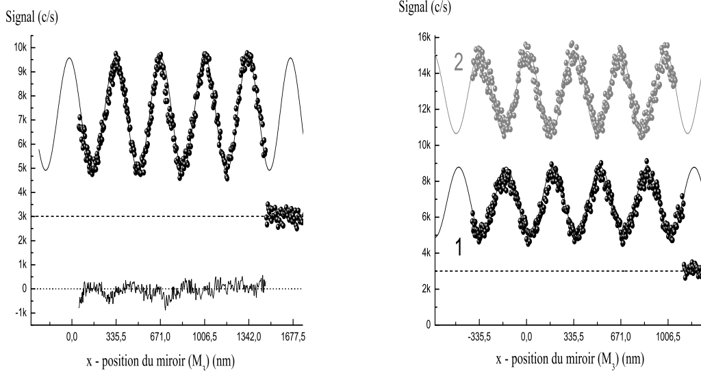
FIG. 4.15 – Graphe de gauche : Franges d'interférence atomique de l'isotope de lithium 6, minoritaire, par diffraction de l'onde atomique au premier ordre. La visibilité atteint 55 % et le flux moyen est I_0 = 4240 c/s. La sortie 1 (noir) est celle dont la visibilité est la plus élevée, l'opposition de phase des deux sorties principales étant visibles sur le graphe de droite.
