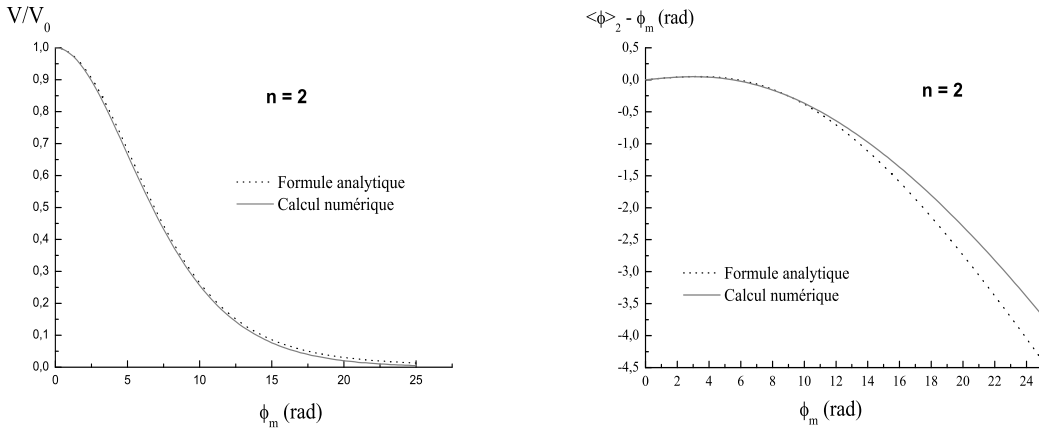
FIG. D.2 – Visibilité et déphasage des franges atomiques obtenus en calculant l'intégrale (D.3) ou par la formule approchée des équations (D.12) et (D.13) pour n = 2 (effet Zeeman). L'accord entre les deux expressions est excellent jusqu'à \phi_m = 25 radians pour la visibilité et jusqu'à 10 radians pour le déphasage (on a représenté l'écart à la phase moyenne \phi_m ).
