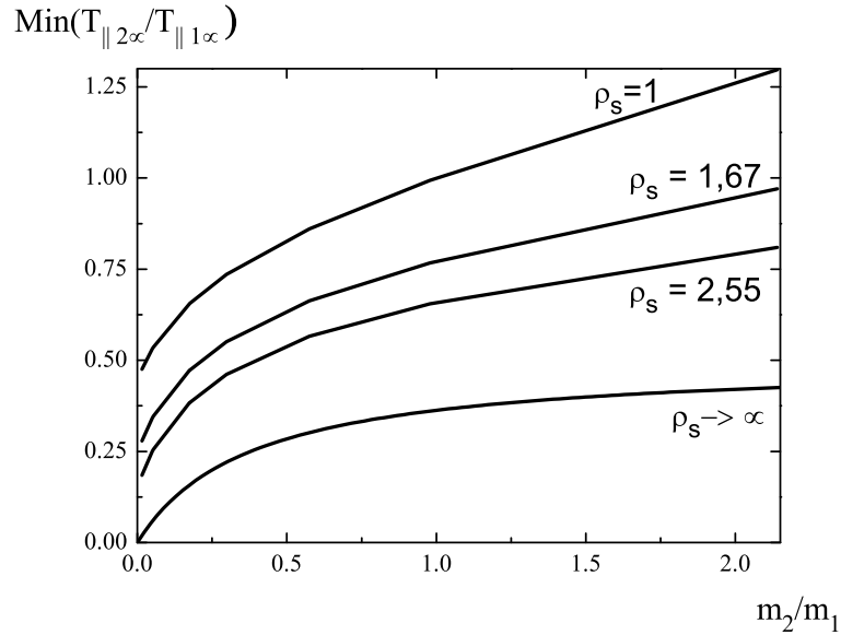
FIG. 2.6 – Rapport des températures terminales T_{||2\infty}/T_{||1\infty} en fonction du rapport des masses pour différentes valeurs de \rho_s . Le rapport m_2/m_1 croît de 0,025 (hydrogèneensemencé dans l'argon) à 2,175 (rubidium dans l'argon), \rho_o restant fixé à 1,32. De bas en haut, on décrit successivement \rho_s \rightarrow \infty , \rho_s = 2,55 (lithium dans argon), \rho_s = 1,67 (sodium dans l'argon) et \rho_s = 1 .
