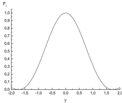
FIG. 3.5 – Probabilité de diffraction en fonction du paramètre de sélectivité y = 2|\kappa - 1|/q pour \phi_r = \pi = 2q\tau .
