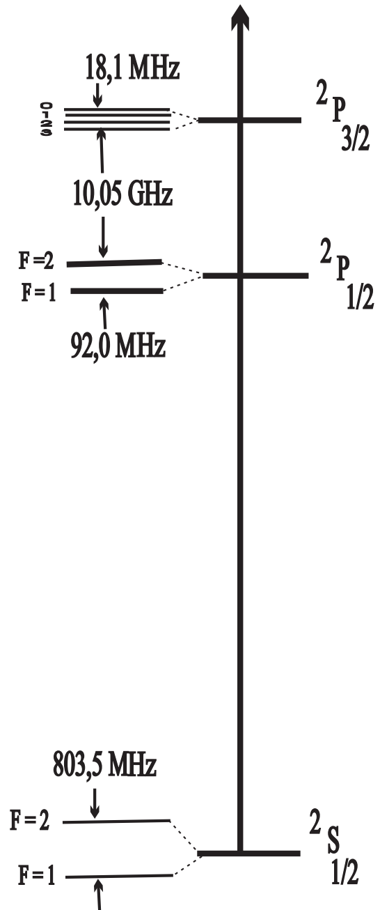
FIG. A.2 – Structure énergétique des premiers niveaux des deux isotopes du lithium tirée des références ([245, 246, 247, 248]). Les écarts énergétiques sont connus avec une très grande précision. Toutefois, seuls les premiers chiffres significatifs sont donnés dans cette figure. Pour chaque isotope, on a représenté par une flèche la transition laser utilisée pour la diffraction de l'onde atomique : l'onde laser est désaccordée vers le bleu de la transition D_2 pour l'isotope 7, vers le rouge de la transition D_1 pour l'isotope 6.
