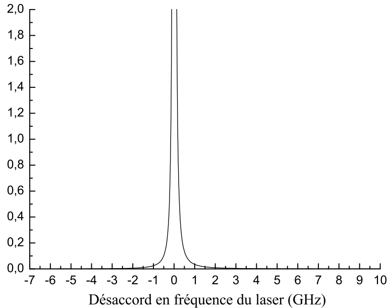
FIG. 3.7 – Emission stimulée (en haut) et émission spontanée (en bas) en fonction du désaccord en fréquence du laser au premier ordre de diffraction. Le jet atomique est pompé optiquement dans le niveau hyperfin F = 1 de l'état fondamental et les données sont calibrées à l'aide d'une cavité confocale. Les courbes en trait plein sont le résultat de la simulation numérique.
