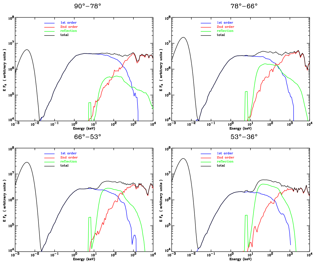
Fig. 8.13: s=3
