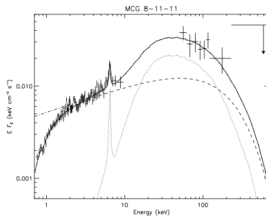
Fig. 8.5: Ajustement des spectres large bande de IC 4329a, MCG 8-11-11 et NGC4151. La composante réfléchie est représentée en pointillés, le direct en tirets
