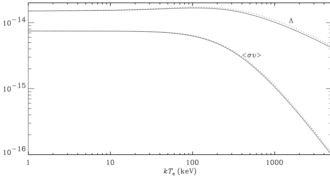
Fig. 1.7: Taux d'annihilation par paire moyen \langle\sigma v\rangle et taux de refroidissement par paire \Lambda en fonction de la température d'un plasma Maxwellien. Les approximations de Svensson (1982) sont montrées en pointillés.
