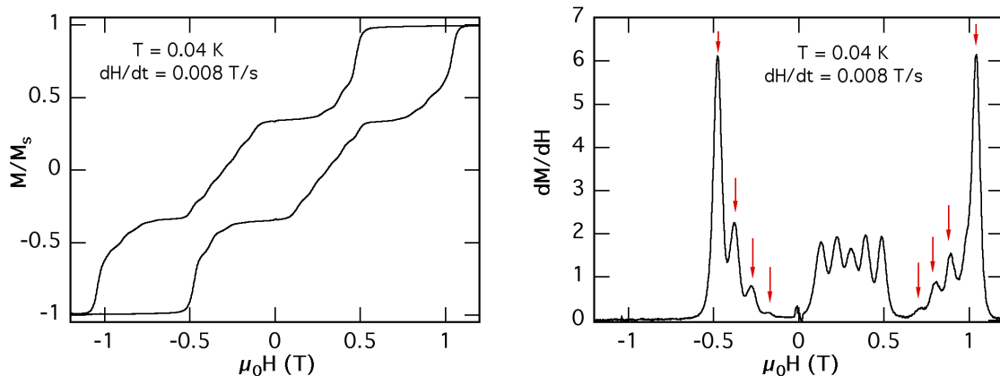
Figure VI-3 : Cycle d'hystérésis (à gauche) et sa dérivée (à droite) mesurés à T = 0,04 K et à une vitesse de balayage du champ dH/dt = 0,008 T/s. On distingue la structure fine des marches en plusieurs sauts.
