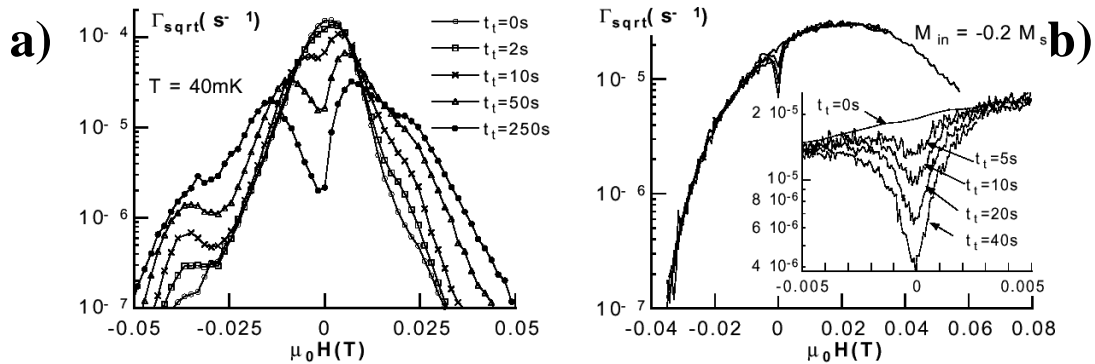
Figure II-12 : Variation du taux tunnel en fonction du champ magnétique appliqué pour différentes valeurs du temps de « digging » t_{\text{digging}} , pour deux valeurs de l'aimantation initiale a) M_{\text{in}} = -0,89 M_s et b) M_{\text{in}} = -0,2 M_s . Le champ de « digging » est H_{\text{dig}} = 0 . Pour le cas b) le profil est gaussien avec une largeur à mi-hauteur de 0,03 T. Dans le cas a) la courbe est déformée par rapport à une gaussienne. Le retournement des moments magnétiques moléculaires (dû au couplage hyperfin) induit un changement important dans le champ interne et certaines molécules sont repoussées loin de la résonance. D'après [Wernsdorfer99c].
