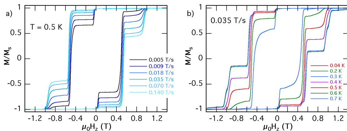
Figure IV-2 : Cycles d'hystérésis d'un échantillon de Mn_4 . a) pour différentes vitesses de balayage du champ et b) pour différentes températures. Les cycles présentent des marches au voisinage du champ nul, autour de 0.5 T et autour de 1 T.
