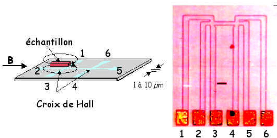
Figure I-3 : À gauche : vue schématique d'un réseau des croix de Hall. Le champ magnétique est appliqué dans le plan de la croix. Le dispositif est sensible au flux de fuite de l'échantillon, perpendiculaire au plan des croix. À droite : image obtenue par microscopie optique. On reconnaît les deux croix lithographiées et les six plot en or, destinés à la prise des contacts électriques. Les croix sont alimentées en courant par les contacts 2 et 5. Le signal correspondant au moment magnétique de l'échantillon est V_1 - V_3 + V_4 - V_6 , où V_i est le potentiel du plot i .
