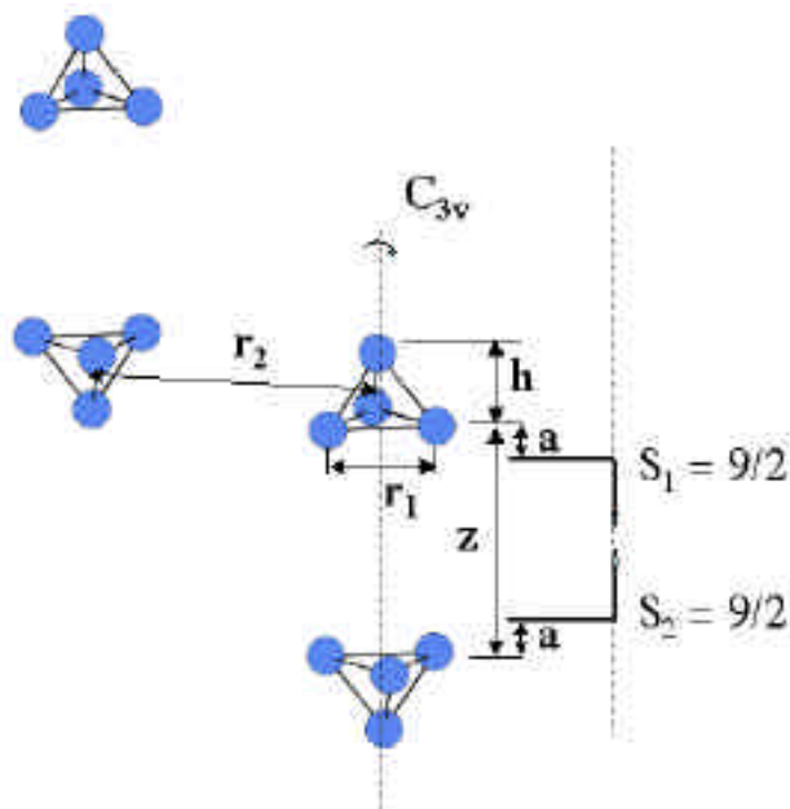
Figure III-3 : Schéma simplifié du dimère : chaque molécule de Mn_4 est représentée par le tétraèdre des quatre ions Mn. Les ions Mn^{3+} se trouvent à la base de la pyramide et l'ion Mn^{4+} au sommet. On définit h , comme la hauteur de chaque tétraèdre de Mn, z la distance entre les deux molécules à l'intérieur du dimère, r_1 l'arrête de chaque tétraèdre et r_2 la distance entre deux molécules appartenant aux dimères voisins.
