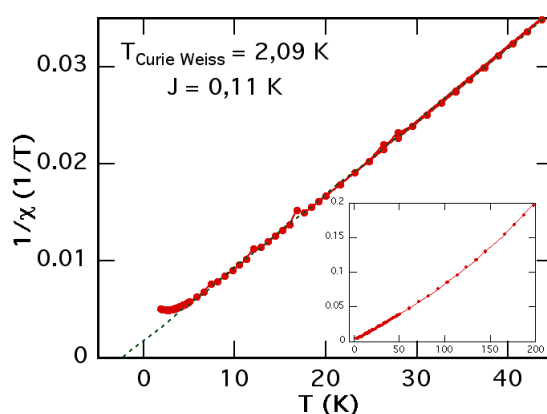
Figure IV-8 : Susceptibilité magnétique mesurée suivant l'axe de facile aimantation pour un cristal moléculaire de (Mn_4)_2 . La ligne en pointillés représente l'ajustement par une loi de Curie-Weiss. La constante de Curie-Weiss est négative - 2,09 K, signature d'un couplage anti-ferromagnétique.
