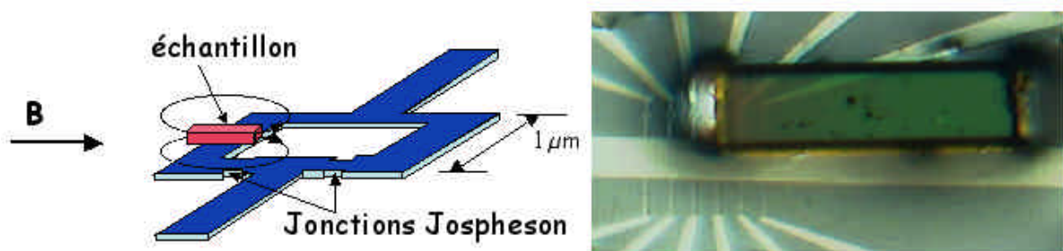
Figure I-1 : À gauche : représentation schématique d'une boucle SQUID ; les constriction sont aussi appelés des micro-ponts. Le champ est appliqué dans le plan du SQUID. Le dispositif est sensible au champ de fuite de l'échantillon. À droite : image par microscopie optique d'un cristal moléculaire posé sur un réseau de douze micro-SQUIDS. La piste centrale est la piste de masse. Le cristal est fixé avec de la graisse.
