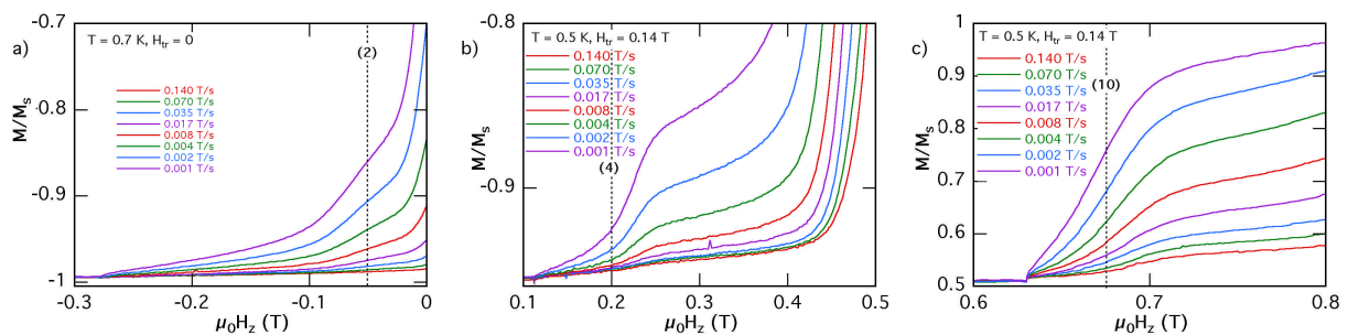
Figure V-7 : Mise en évidence de résonances (2), (4) et (10) dans Mn_4 . Les différentes courbes correspondent à différentes vitesses de balayage du champ. La résonance (2) dans le premier graphique correspond à l'effet tunnel entre les états (-9/2, +5/2) et (+7/2, +7/2) ; la résonance (4) dans le deuxième graphique correspond à l'effet tunnel entre les états (-9/2, +5/2) et (+9/2, +3/2) et la résonance (10) dans le dernier graphique correspond à l'effet tunnel entre les états (-7/2, +9/2) et (+7/2, +7/2) . Ces résonances ne sont pas directement accessibles dans le cycle d'hystérésis total. Elles ont été mises en évidence sous l'effet de la température et à l'aide du champ transverse. Pour plus de détails voir le texte.
