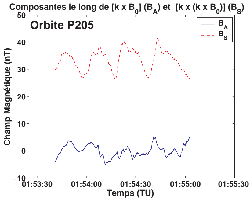
Figure V.36. Champ magnétique le long de k \times B_0 et k \times (k \times B_0) ( B_A et B_S , respectivement), pour un événement en aval de la MPB [Bertucci et al., 2004a].
