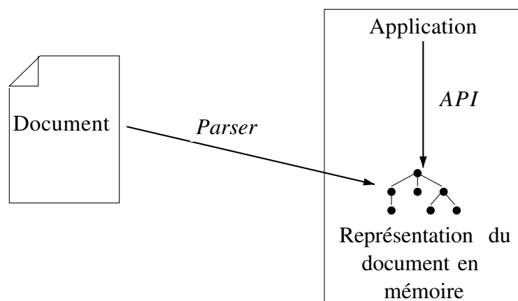
Figure 7 : Application de traitement de documents structurés
