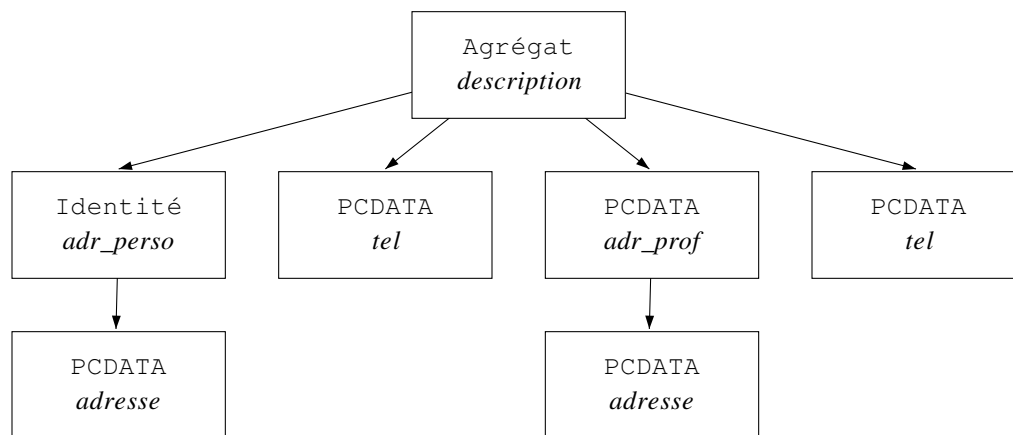
Figure 29 : Arbre canonique du type description
