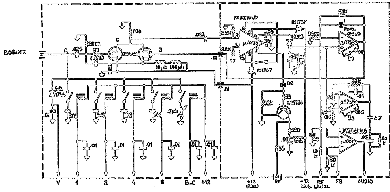
Oscillateur Anderson
