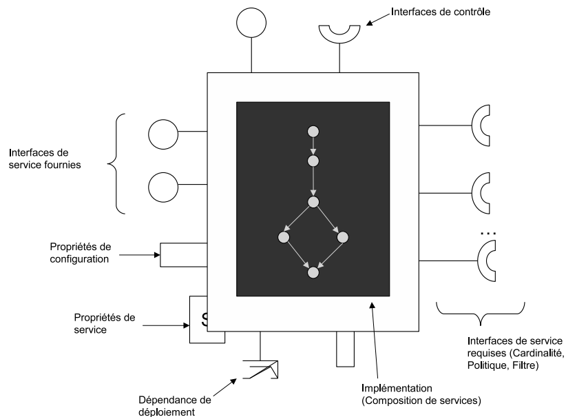
FIGURE 5.10 – Classe de composant de service selon [Cervantes, 2004]
