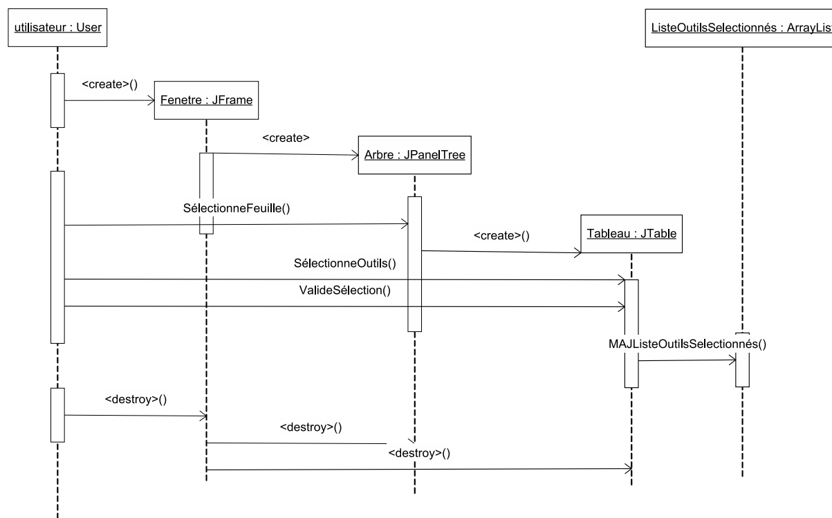
FIGURE 4.32 – Diagramme de séquence montrant les méthodes à développer pour réaliser l'activité "Afficher le mode par thème"
