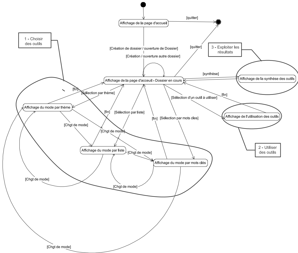
FIGURE 4.25 – Diagramme états-transitions pour la spécification des IHM
