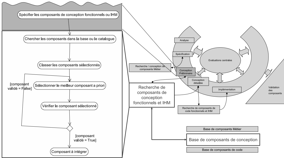
FIGURE 3.27 – Etape de recherche de composants de conception
