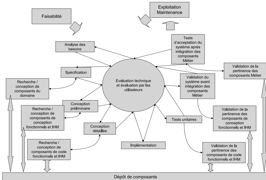
FIGURE 3.4 – ADESIAD : le modèle, vue complète
