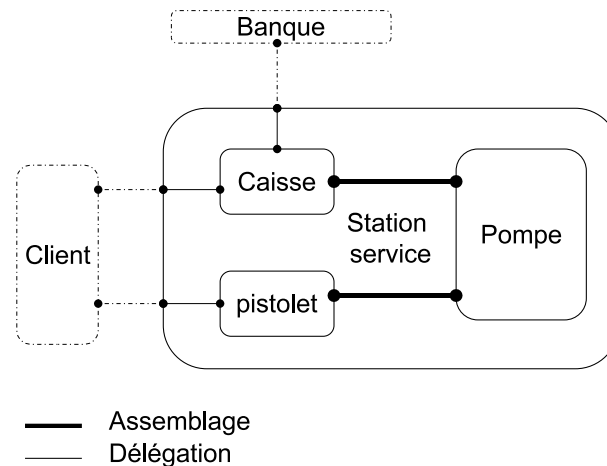
FIGURE 2.19 – Exemple d'architecture proposé par [Barais and Duchien, 2004]
