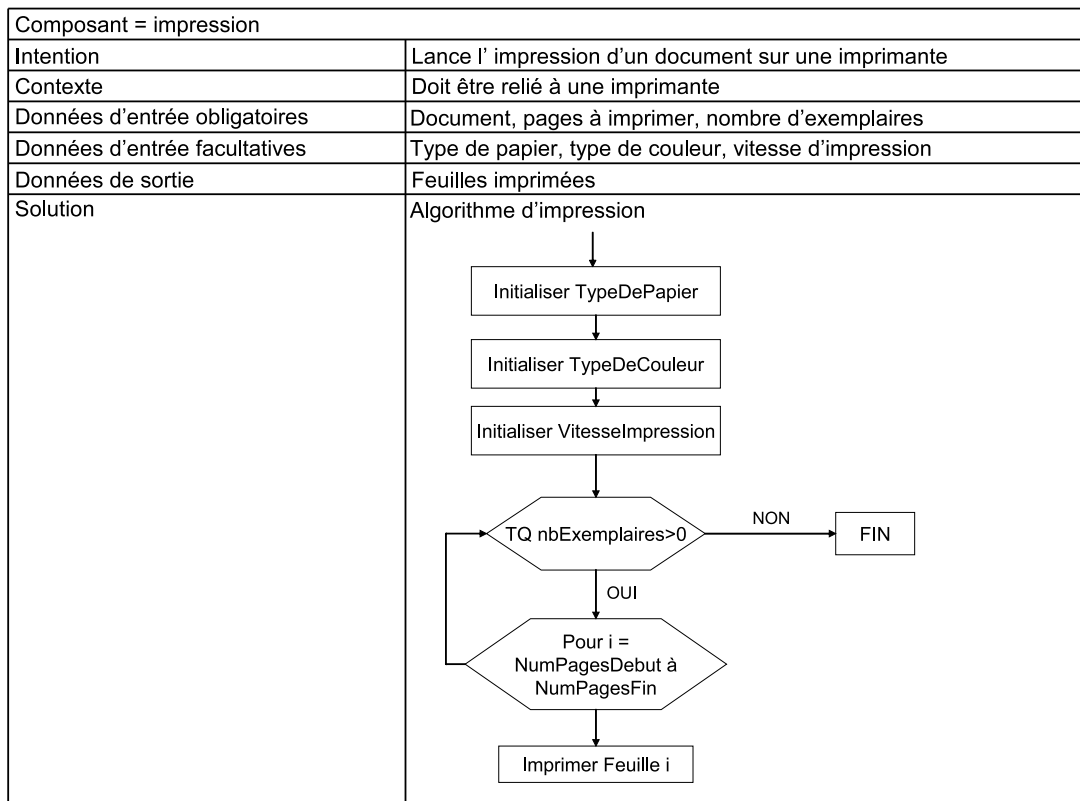
FIGURE 3.17 – Exemple d’instanciation du patron de composant au logiciel d’impression
