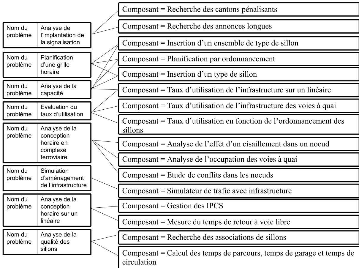
FIGURE 4.17 – Association des composants métier aux problèmes non décomposables correspondant à la seconde décomposition vue en Figure 4.7
