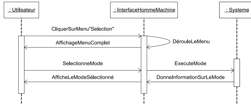
FIGURE 4.21 – Diagramme de séquence modélisant les interactions de la tâche "Choix du mode de présentation"
