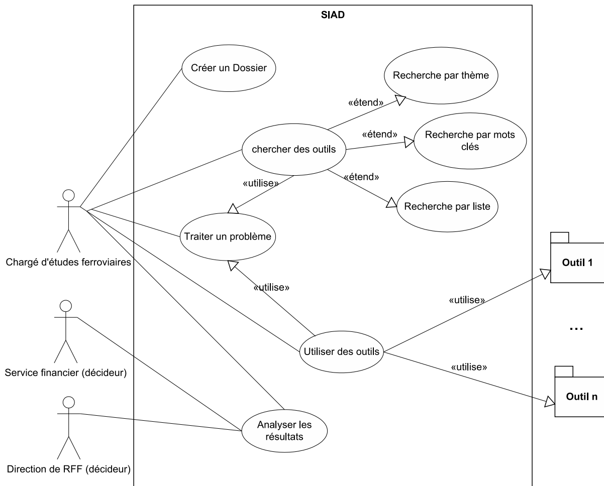
FIGURE 4.13 – Diagramme des cas d'utilisation du SIAD
