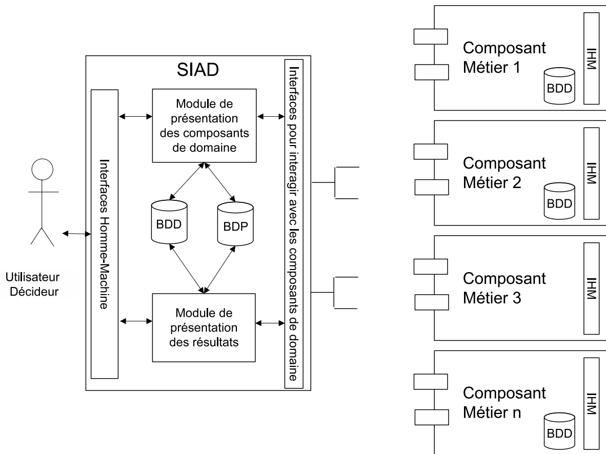
FIGURE 3.32 – Architecture de SIAD basé sur les composants
