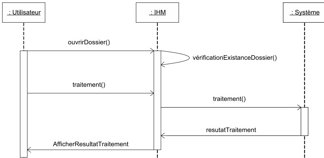
FIGURE 4.23 – Scénario d'utilisation correcte du système
