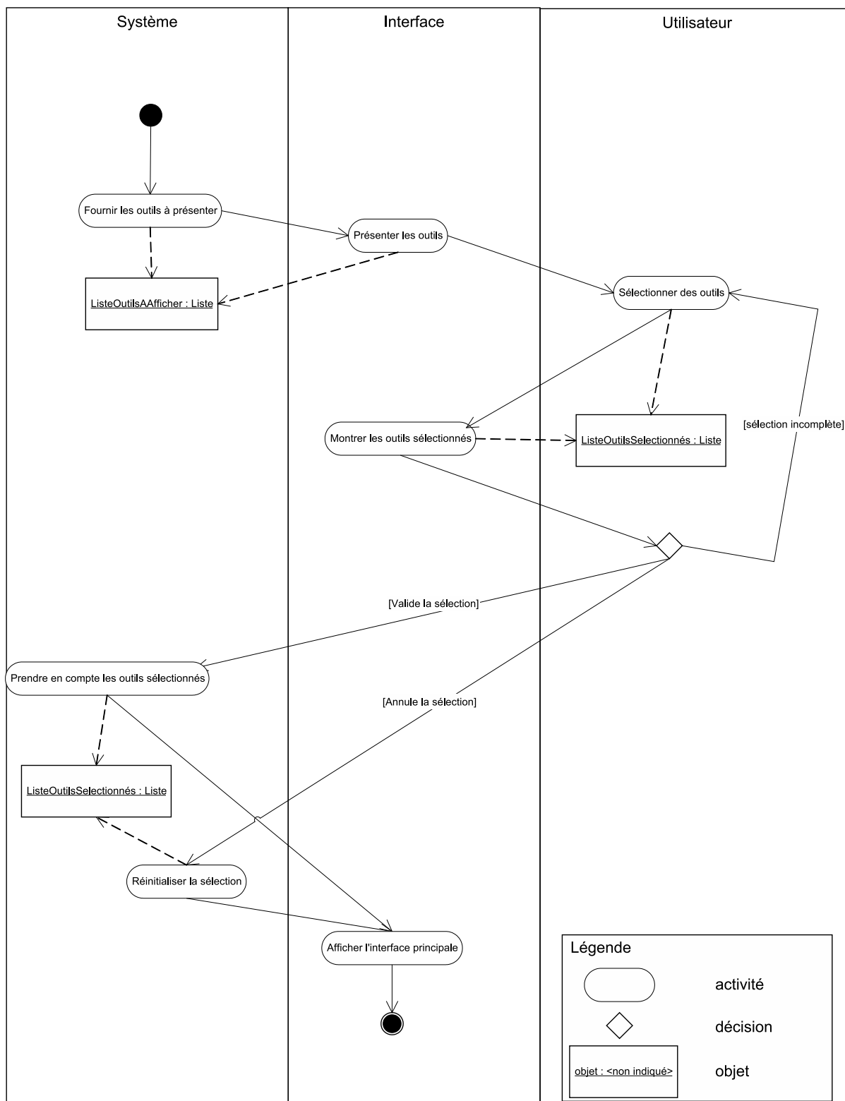
FIGURE 4.22 – Diagramme d’activités modélisant la dynamique de la tâche interactive "Sélectionner les outils"
