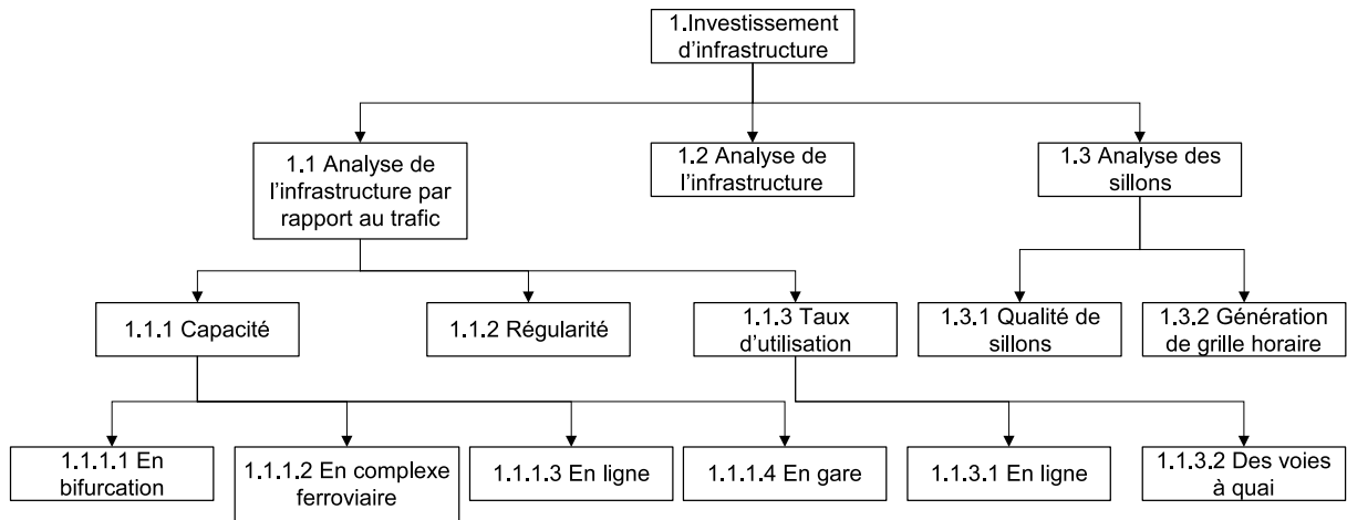
FIGURE 4.8 – Troisième décomposition du problème d'investissement faite à l'aide des patrons
