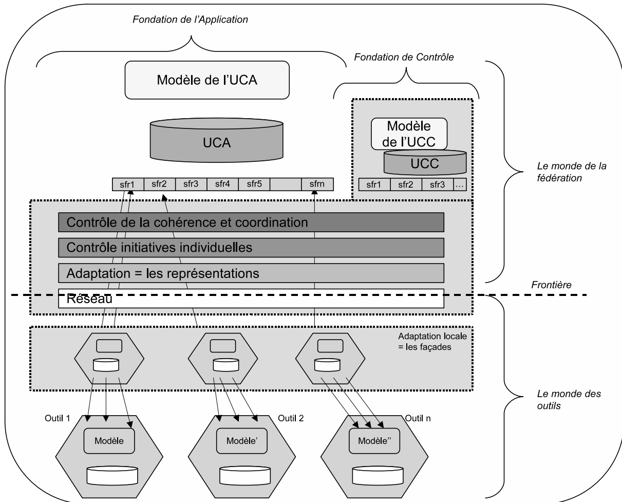
FIGURE 5.9 – Architecture pour fédération d'outils [Le et al., 2003]
