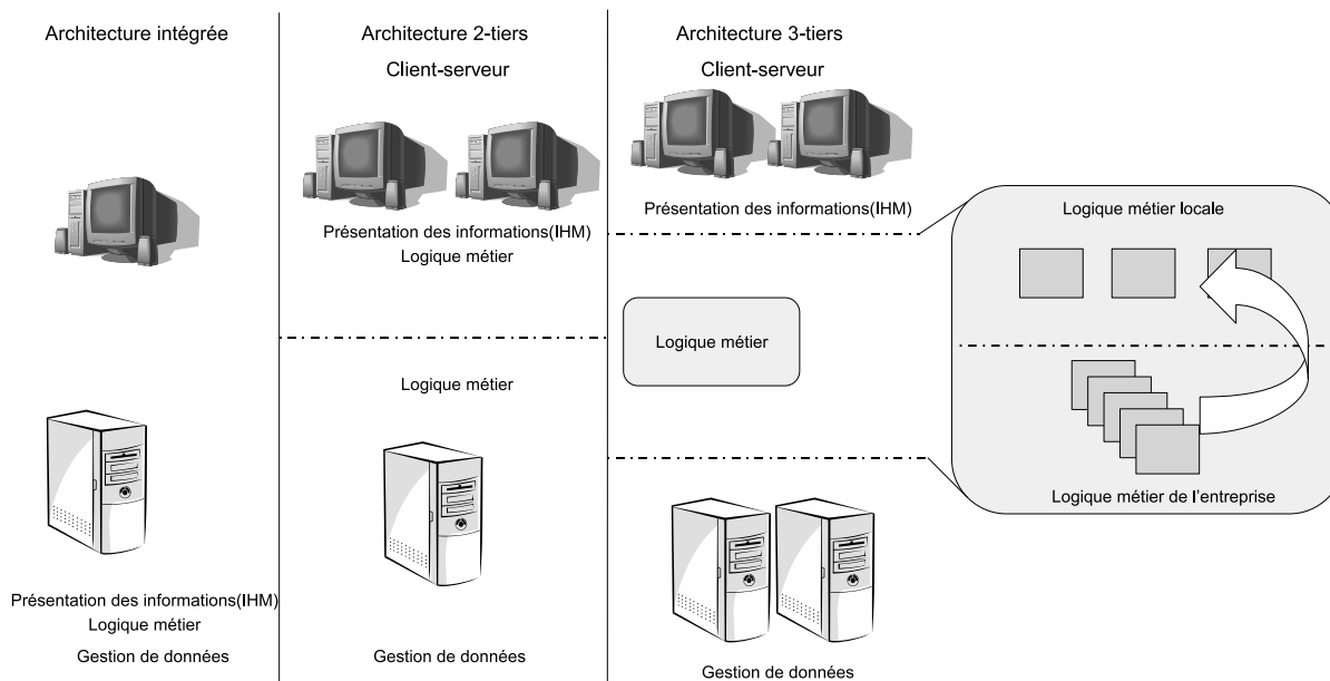
FIGURE 2.18 – Evolution des architectures vers une architecture logicielle orientée métier, traduit de [Allen and Frost, 1998]
