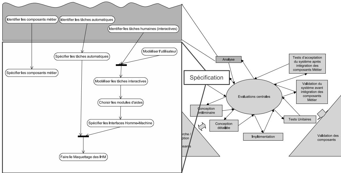
FIGURE 3.15 – Etape de spécification
