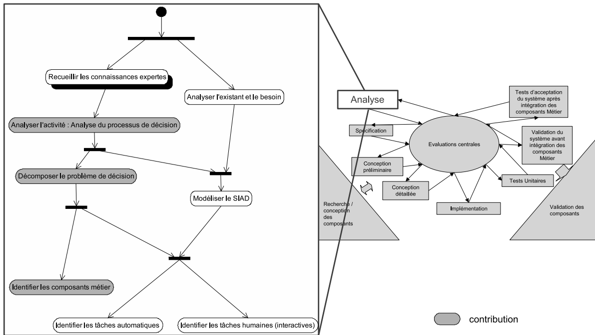
FIGURE 3.6 – Diagramme d'activité de l'analyse des besoins
