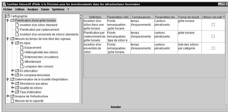
FIGURE 4.28 – Maquettage "dynamique" de la sélection d'outil selon le mode par thèmes
