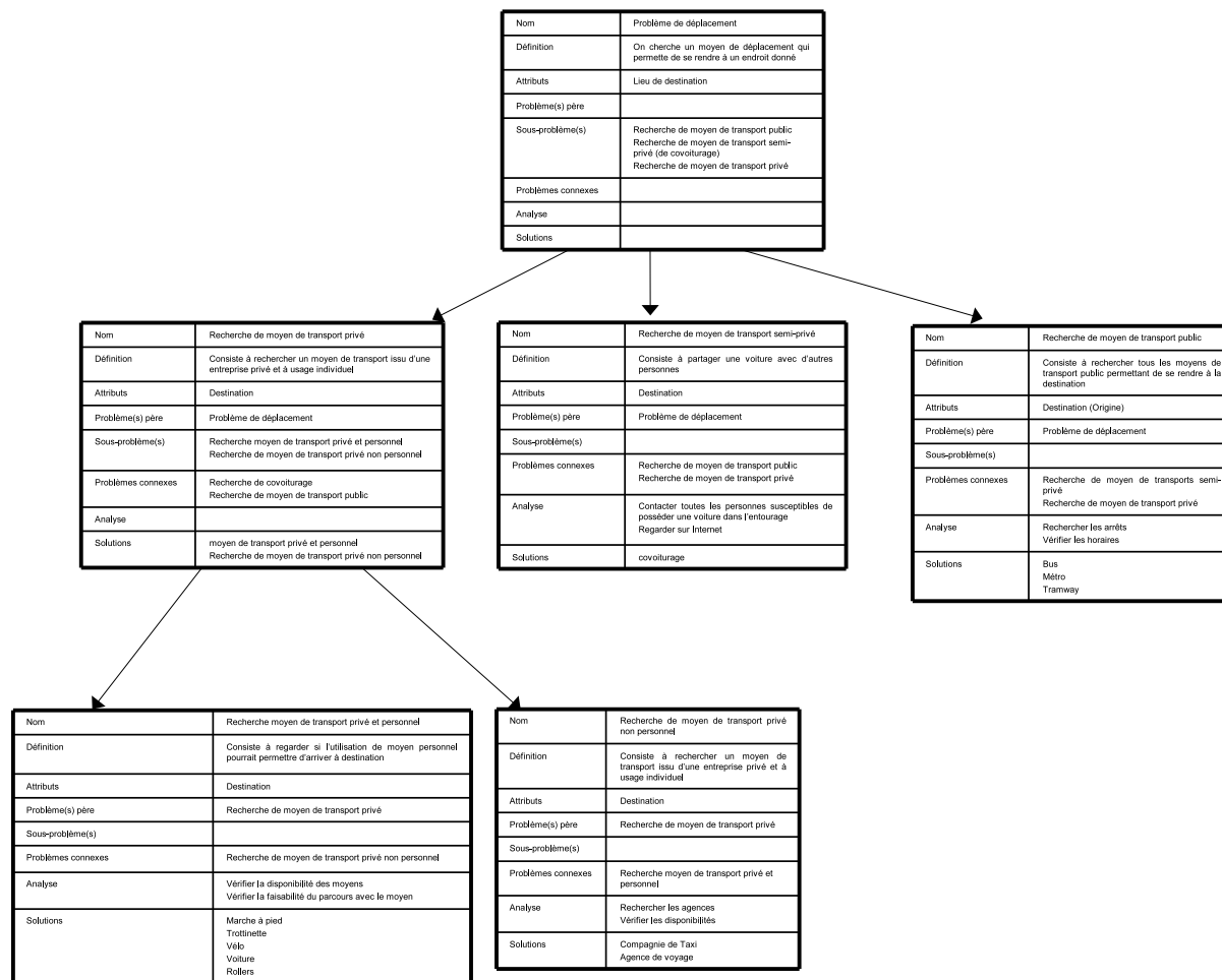
FIGURE 3.13 – Exemple de décomposition d'un problème de déplacement, mise en forme à l'aide du diagramme de patron de problème
