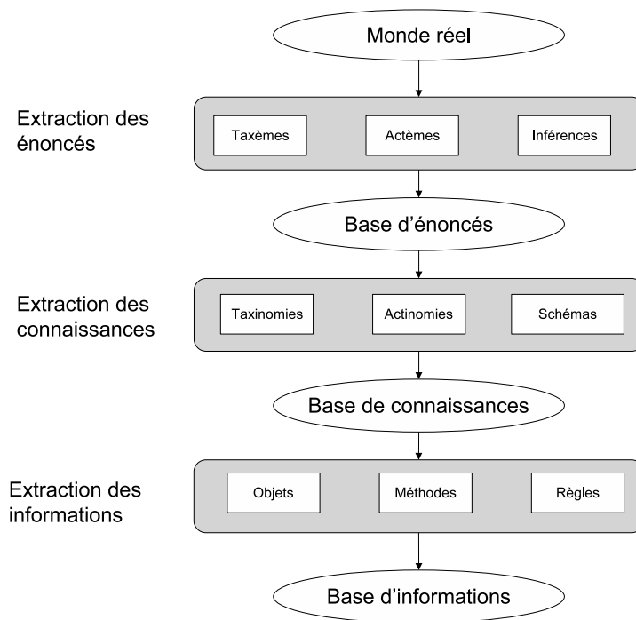
FIGURE 2.21 – Les trois niveaux de KOD [Vogel, 1988]
