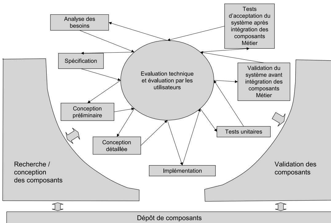
FIGURE 3.2 – ADESIAD : le modèle, vue des étapes de développement du SIAD
