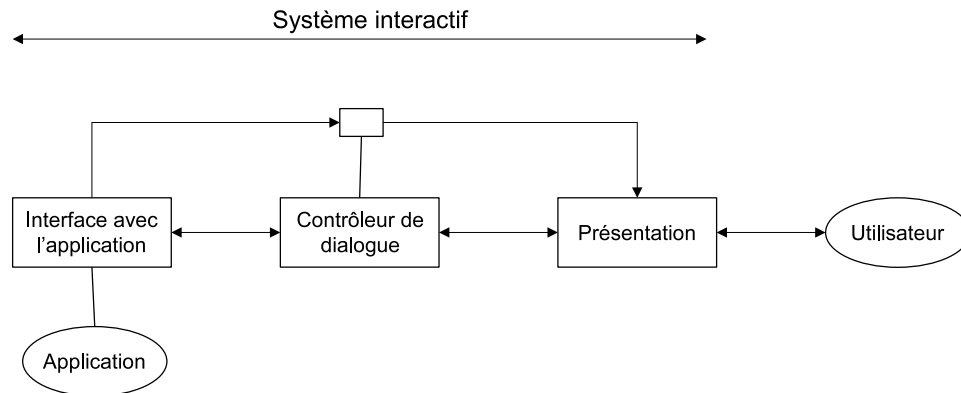
FIGURE 2.11 – Modèle de Seeheim
