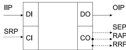
FIGURE 1.4 – Interface d'un composant selon [Aniorté, 2002]
