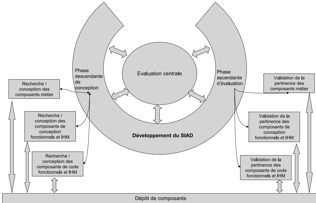
FIGURE 3.3 – ADESIAD : le modèle, vue de la réutilisation
