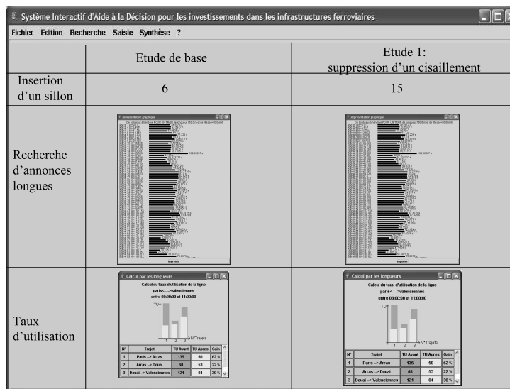
FIGURE 4.29 – Maquettage "mixte" de l'affichage correspondant à la synthèse
