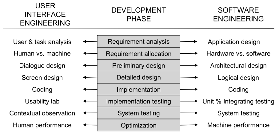
FIGURE 2.7 – Modèle de Curtis et Hefley [Curtis and Hefley, 1994]
