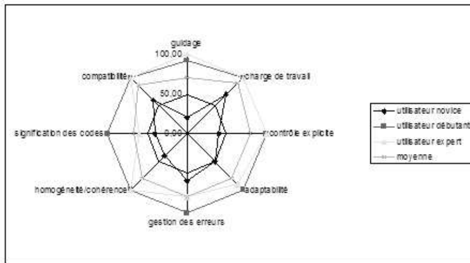
FIGURE 4.36 – Résultats globaux relatifs à l'utilisabilité du système
