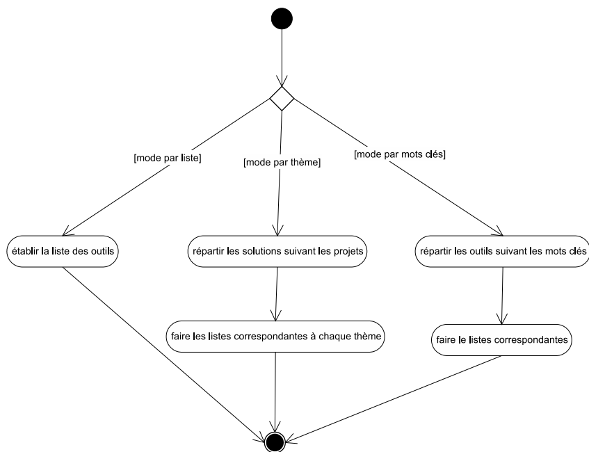
FIGURE 4.20 – Diagramme d'activités de la tâche automatique "Présenter les outils"
