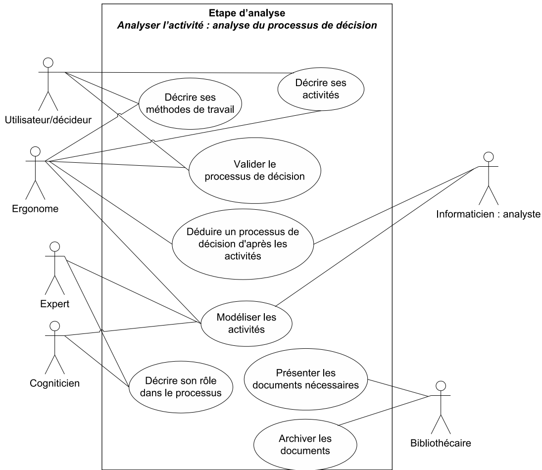
FIGURE 3.9 – Diagramme des cas d'utilisation de l'analyse des activités, du processus de décision
