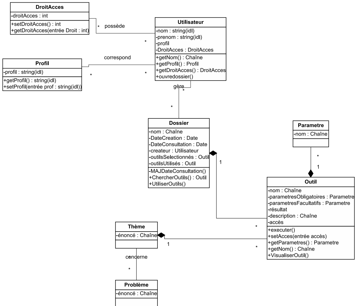
FIGURE 4.15 – Diagramme de Classes conceptuel de SIADIF
