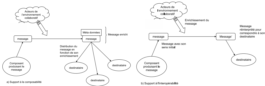
FIGURE 5.6 – Enrichissement de message d'après [Payet, 2003]
