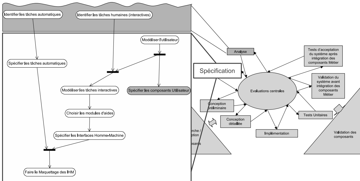
FIGURE 5.3 – Modification possible de la méthode d'ADESIAD pour intégrer les composants utilisateur
