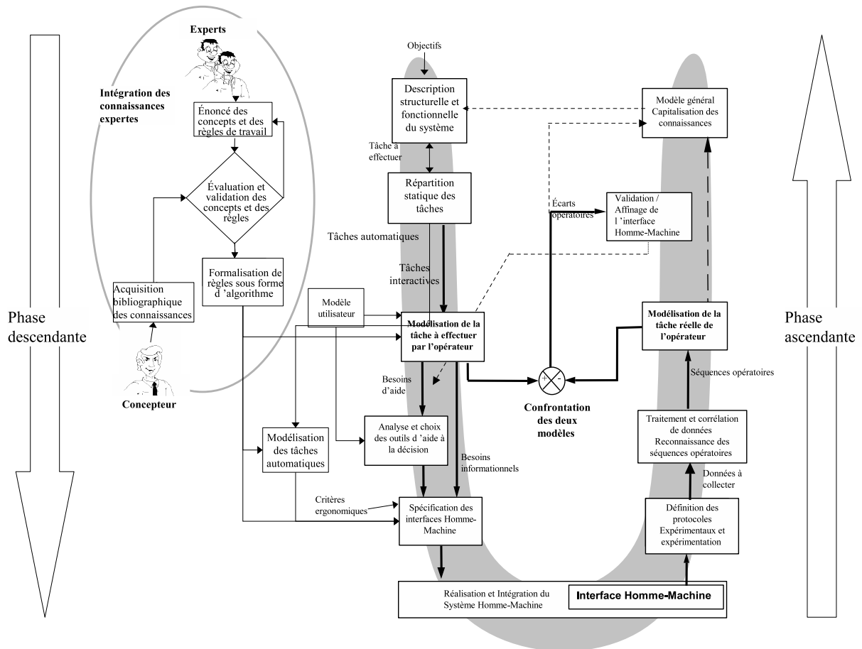
FIGURE 4.1 – Modèle en U adapté pour la prise en compte d'experts [Lepreux et al., 2001a]
