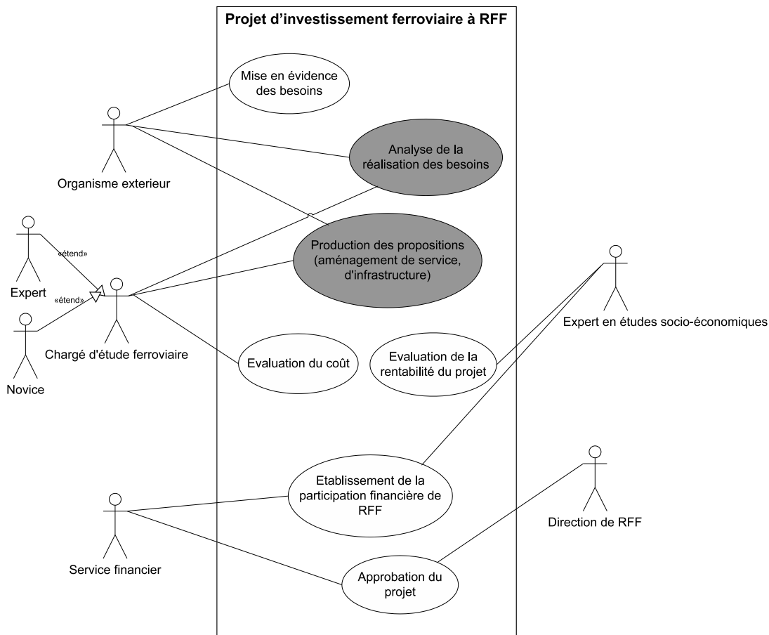
FIGURE 4.3 – Diagramme des cas d’utilisation pour la réalisation d’un projet d’investissement (les cas grisés sont ceux pris en compte dans la conception de SIADIF)
