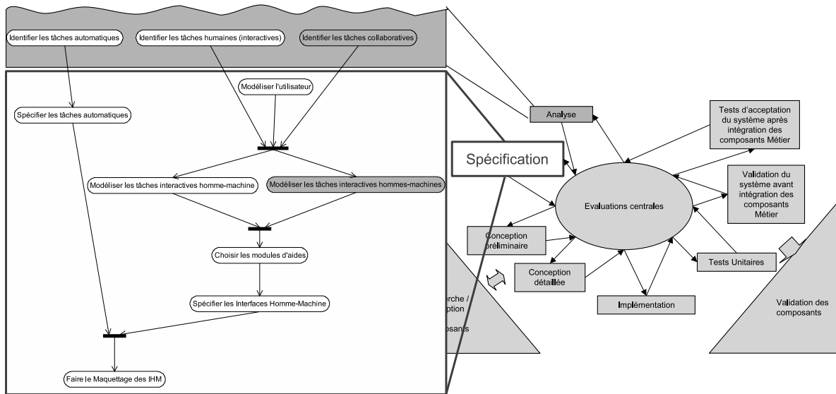
FIGURE 5.2 – Modification possible de la méthode d'ADESIAD pour intégrer les tâches collaboratives
