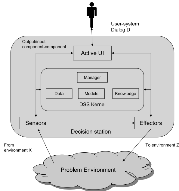
FIGURE 2.24 – Architecture générale pour un SIAD [Vahidov and Kersten, 2004]
