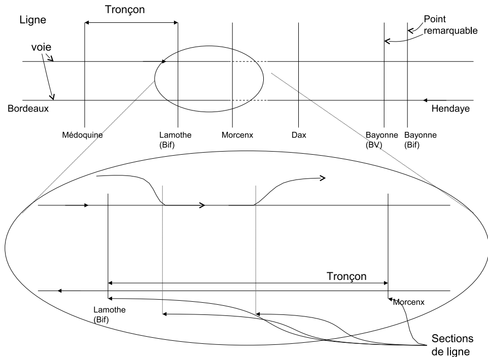
FIGURE 1.11 – Schéma ferroviaire
