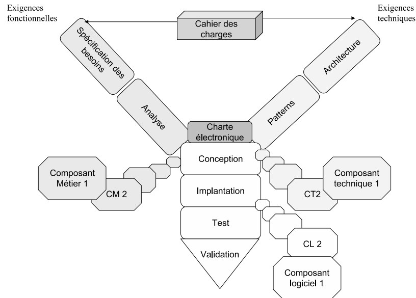
FIGURE 2.16 – Modèle en Y [Hassine et al., 2002b]
