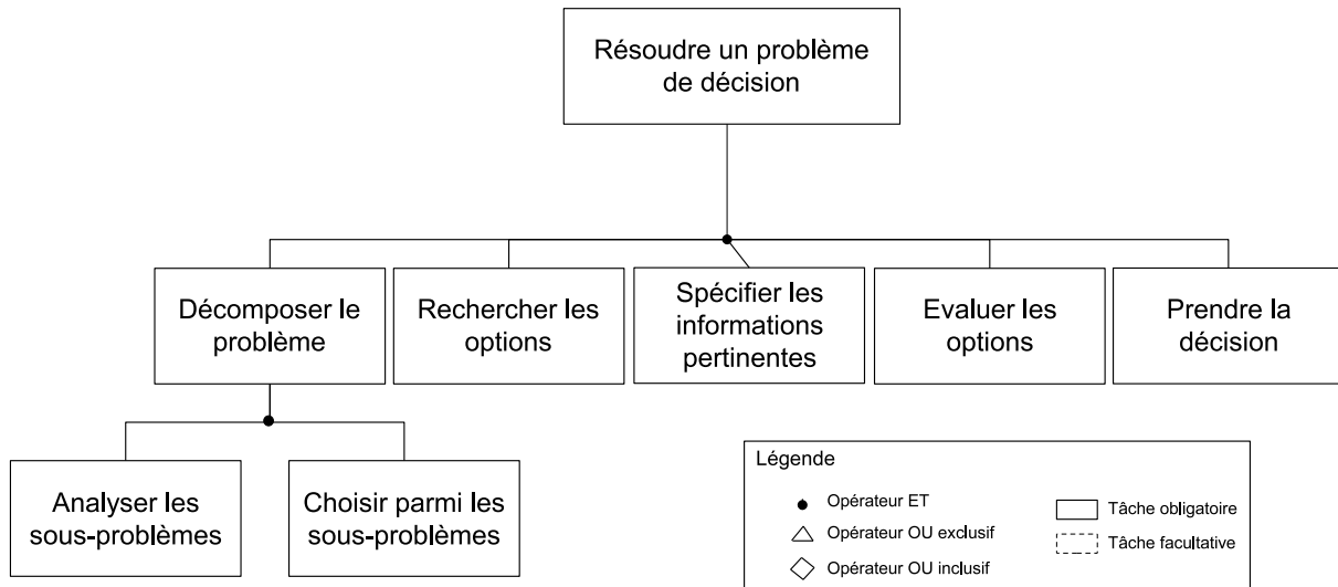
FIGURE 3.14 – Exemple d'arborescence de tâches de "Résoudre un problème" selon [Buisine, 1999]
