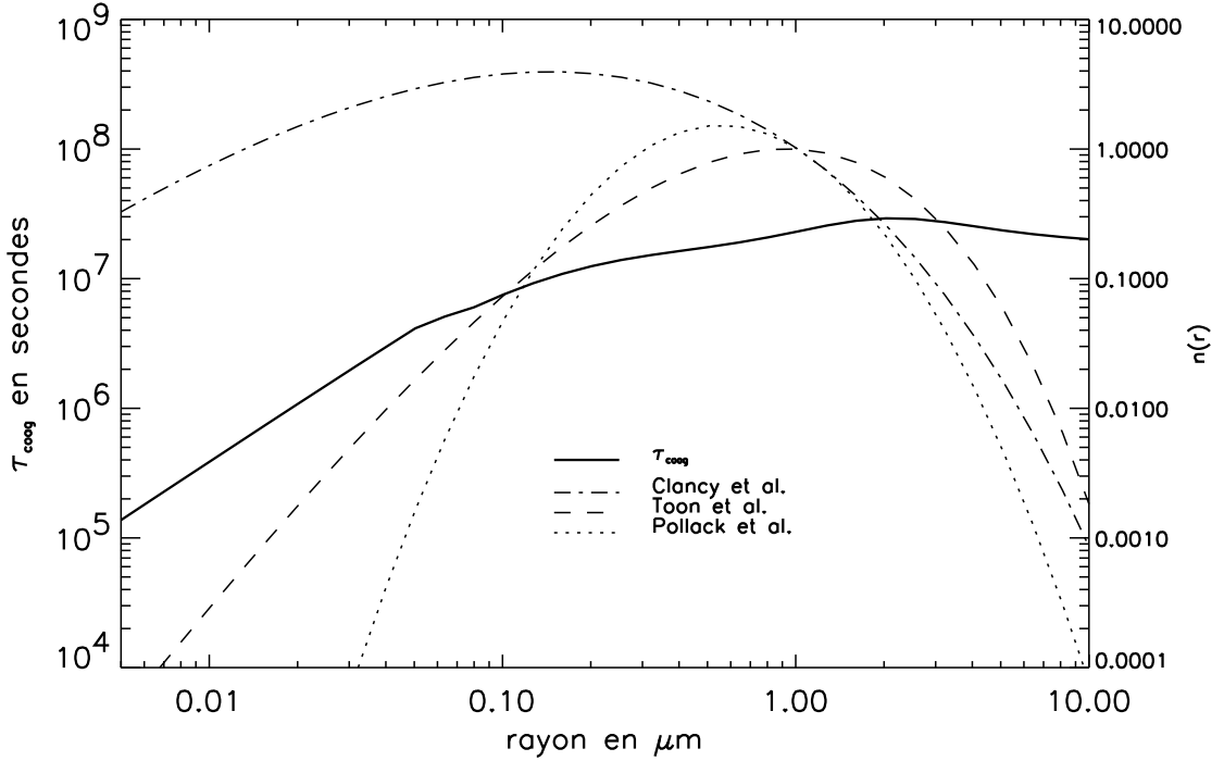
Figure 2.8 : \tau_{\text{coag}} estimé de la poussière martienne en fonction de son rayon. Trois distributions en taille ont été superposées (normalisées à leur densité numérique à 1 \mu\text{m} ) afin d'illustrer la réponse de l'accrétion à un spectre donné. Sans commettre d'erreur notable, on peut supposer les particules uniformément mélangées ( n \propto \rho_a ). Puisque (5.16) et (5.18) donnent une dépendance de K en \rho_a^{-1} , le terme \int nK ne dépend pas, en première approximation, de l'altitude.
