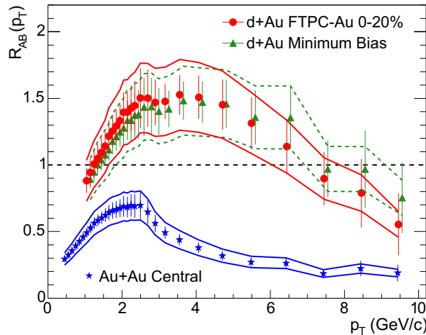
FIG. 1.11 – Rapport R_{AB}(p_T) des hadrons chargés obtenu en collision d -Au et Au-Au à 200 \text{ GeV}/c/\text{nucléon} [32].
