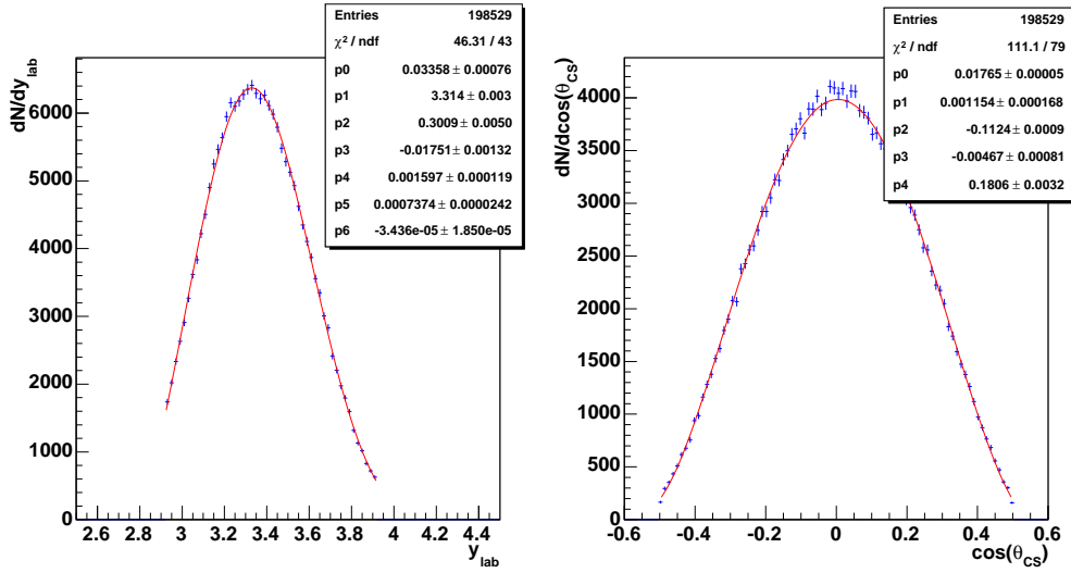
FIG. 7.3 – Ajustement des distributions en rapidité (à gauche) et en \cos\theta_{CS} (à droite) des événements J/\psi simulés avec NaGenParam.
