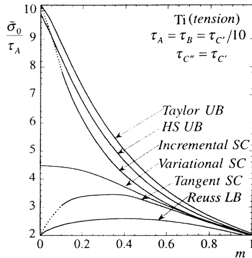
FIG. 3.10 – Contrainte de référence macroscopique en fonction du taux de sensibilité à la contrainte m=1/n . Pour une déformation en traction uniaxiale d'un polycristal isotrope de titanium. Comparaison entre différentes approches auto-cohérentes. D'après Gilormini et al. (2001).
