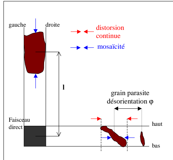
FIG. 2.8 – Schéma de principe de mesure des distorsions : mosaïcité et distorsion continue de part et d'autre de l'échantillon, et détection d'un grain parasite ou d'un sous grain. l est la distance faisceau direct-tâche de diffraction. Ces tâches fournissent aussi une localisation dans l'échantillon, de gauche à droite de l'échantillon sur la tâche du haut (par rapport au faisceau direct), de bas en haut de l'échantillon sur la tâche de droite.
