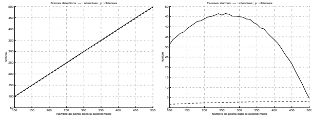
FIG. B.11 – Méthode de KAPUR, SAHOO et WONG – Premier test
