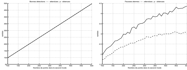
FIG. B.14 – Méthode des deux gaussiennes – Premier test
