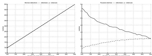
FIG. B.19 – Méthode isodata – Premier test
