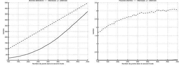
FIG. B.13 – Méthode des moments – Premier test
