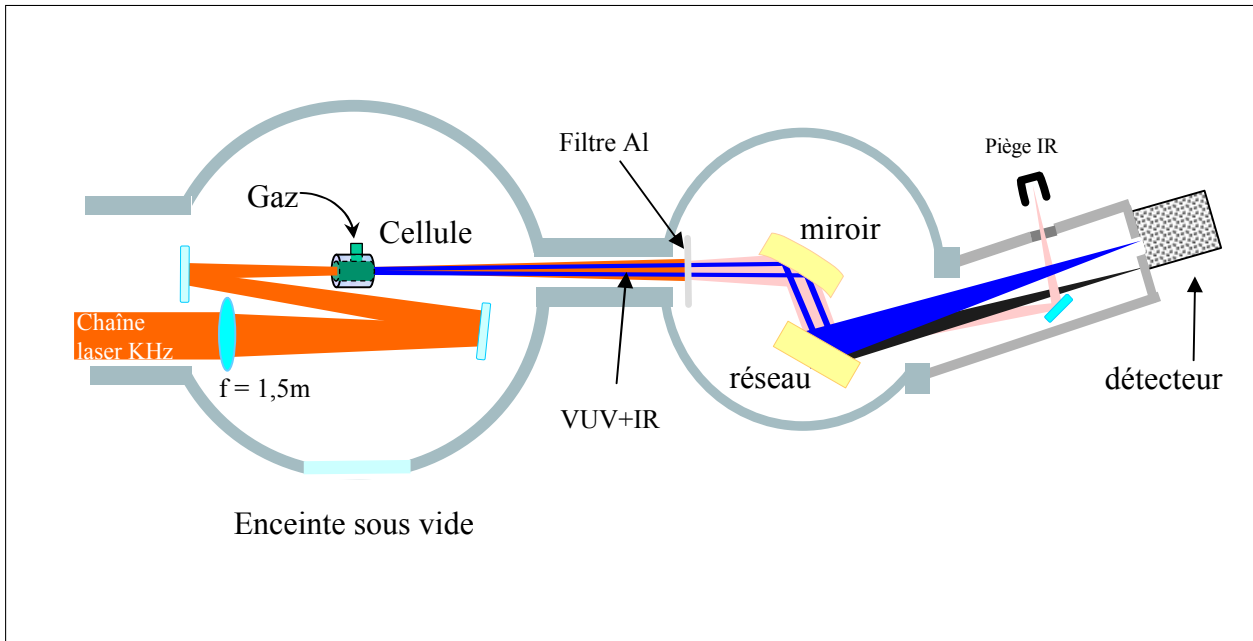
Fig. 3.5 : Dispositif expérimental pour la génération d'harmoniques d'ordres élevés à CELIA.
