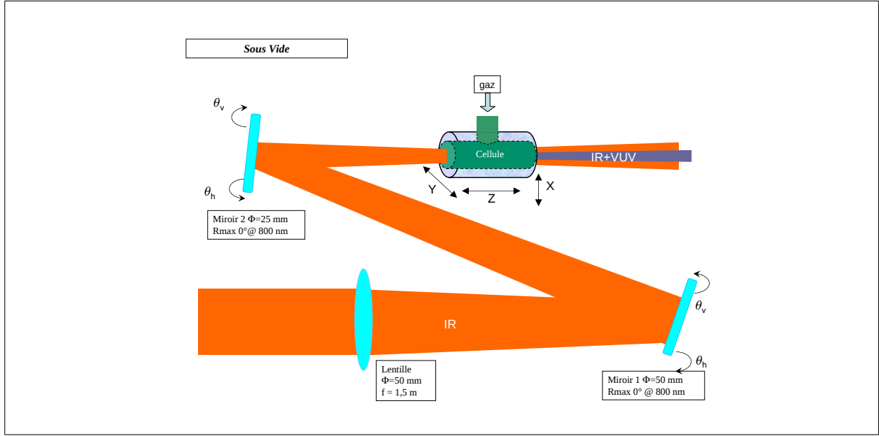
Fig. 3.6 : Détail du dispositif avec la lentille.
