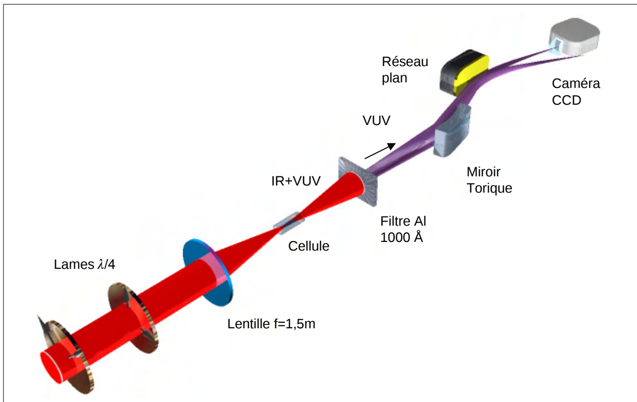
Fig. 3.1 : Dispositif expérimental.
