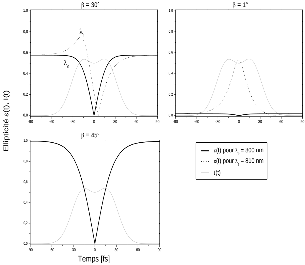
Fig. 2.11 : Ellipticité du champ en fonction du temps pour \lambda_0 (trait plein épais) et \lambda_1 (trait plein fin). L'intensité en sortie de la lame ne change pas (trait pointillé). L'impulsion est Gaussienne \tau = 35 fs, t_e = 35 fs, \theta = 45^\circ .
