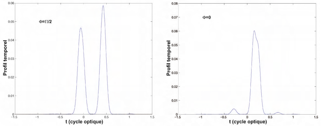
Fig. 1.3 : Profils temporels des harmoniques de la coupure sélectionnées par un filtre Gaussien de largeur 9\omega_0 pour \Phi = \pi/2 (à gauche) et \Phi = 0 (à droite) [de Bohan et al. 98].
