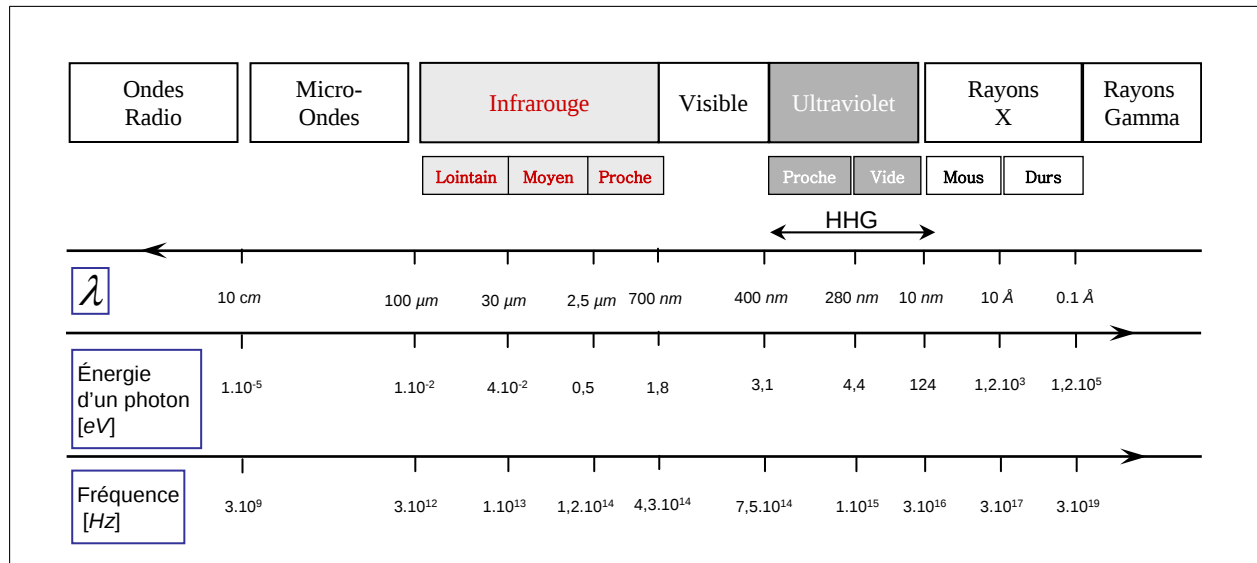
Fig. 3 : Spectre électromagnétique.
