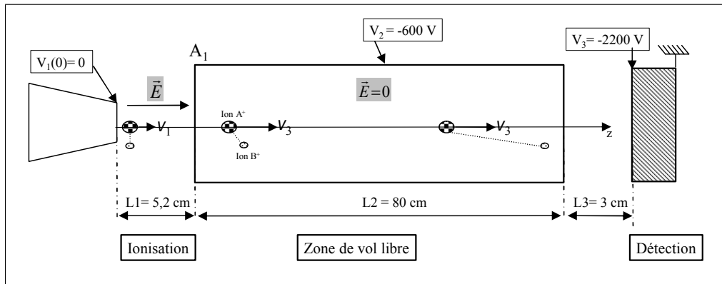
Fig. 2.8 : Spectromètre à temps de vol. L'ion A^+ , plus lourd que l'ion B^+ , a un temps de vol plus long que l'ion B^+ .
