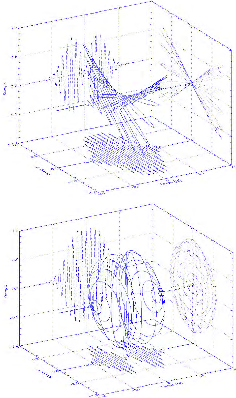
Fig. 2.8 : Évolution du champ électrique en 3D en porte large (haut) et en porte étroite (bas). L'impulsion incidente est Gaussienne de durée à mi-hauteur en intensité \tau = 10 fs, t_e = 13 fs.
