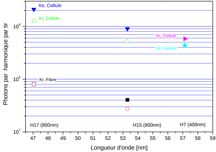
Fig. 3.11 : Nombre de photons par harmonique en fonction de la longueur d'onde des harmoniques pour différents dispositifs expérimentaux:
