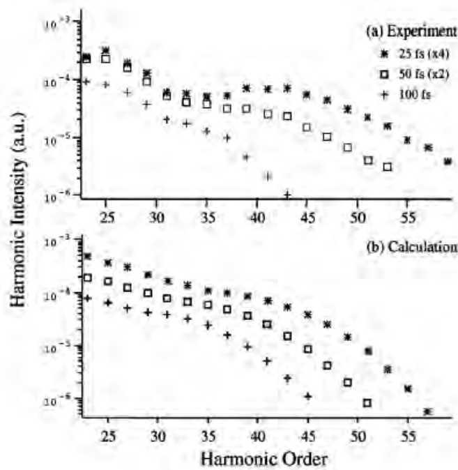
Fig. 2.5 : (a) Harmoniques générées dans l'argon par une impulsion de durée proche de la limite de fourier de 25 fs (*), 50 fs (□) et 100 fs (+) avec une intensité de 4 \times 10^{14} \text{ W/cm}^2 . La cellule de gaz de longueur 1 mm est placée 2,5 cm après le foyer. D'après [Christov et al. 96].
