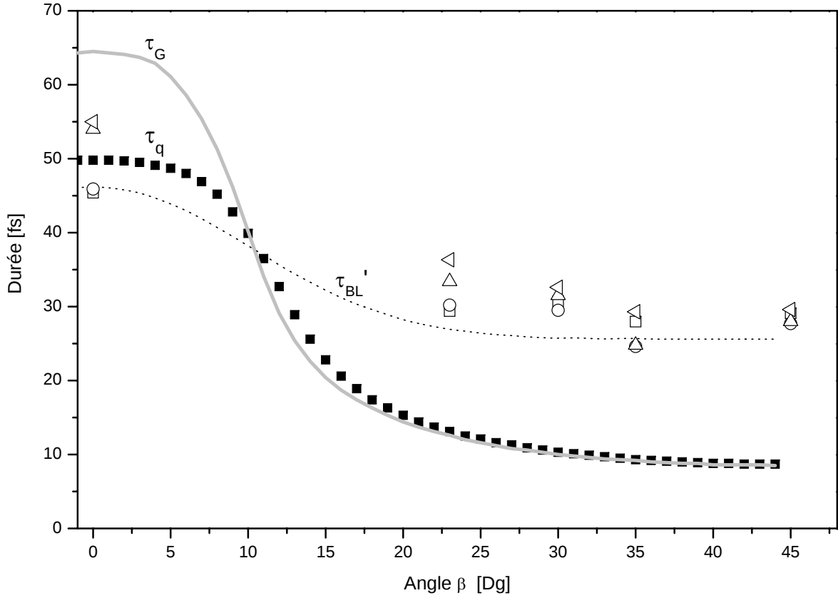
Fig. 4.9 : Largeur à mi-hauteur des bandes latérales expérimentales de 14 à 20 en fonction de l'angle \beta (respectivement \square , \circ , \triangle , \diamond ). La largeur de la porte d'ellipticité \tau_G est représentée (trait gris) ainsi que la largeur à mi-hauteur de l'émission harmonique ( \blacksquare ) et enfin la largeur de la fonction d'inter-corrélation attendue (trait noir pointillé).
