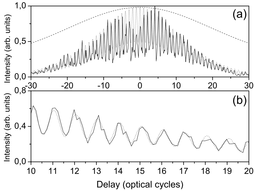
Fig. 3.9 : (a) Variation du signal de l'harmonique d'ordre 11 en fonction du délai t_e . En présence de la porte d'ellipticité (trait plein), la simulation (trait pointillé) et sans porte (trait pointillé long).
