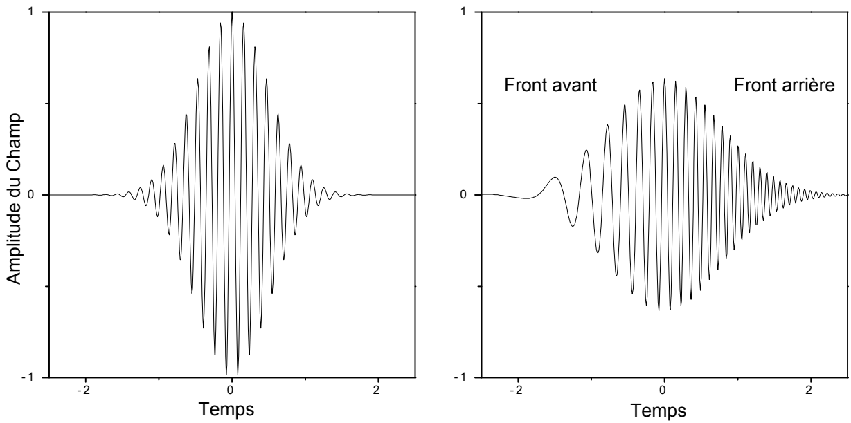
Fig. A.2 : Champ électrique initiale et après propagation dans un milieu dispersif , on note dans le dernier cas l'étalement des fréquence et l'allongement de la durée
