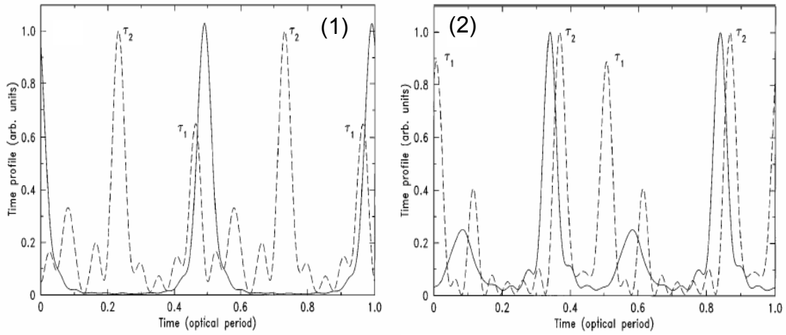
Fig. 1.17 : (1) Profil temporel de l'émission harmonique après propagation dans le milieu atomique, le jet atomique de longueur 1mm est placé 2 mm après le foyer [ z = 2 mm] (trait plein). (2) Profil temporel de l'émission harmonique après propagation dans le milieu atomique le jet atomique est au foyer [ z = 0 ] (trait plein). La réponse de l'atome unique est représentée en pointillé.
