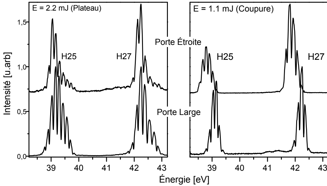
Fig. 3.4 : Spectres des harmoniques 25 et 27 générées dans 30 mbar d'argon en porte étroite (haut de la figure) et porte large (bas de la figure). Les harmoniques 25, 27 sont dans le plateau (Å gauche) et dans la coupure (Å droite).
