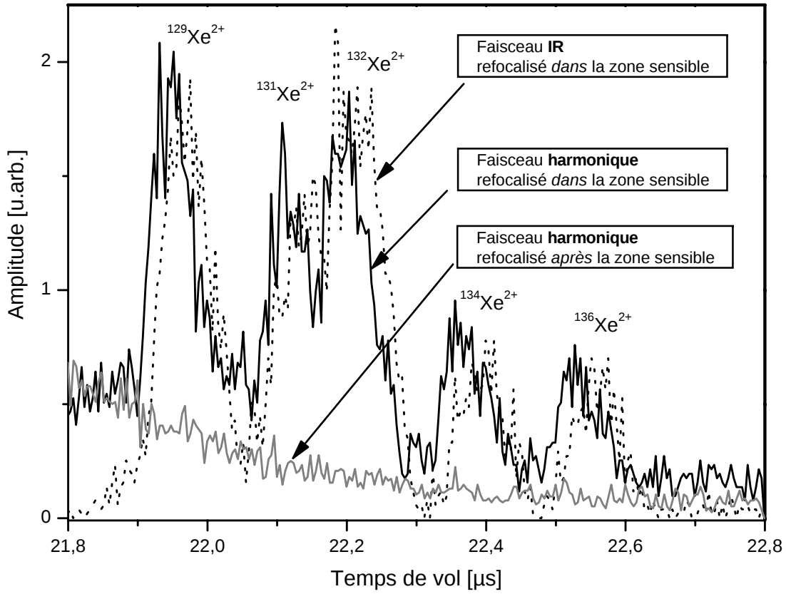
Fig. 2.16 : Temps de vol des ions \text{Xe}^{2+} . Signal d'ions (trait plein) dû au faisceau harmonique refocalisé dans la zone sensible ( z=0 mm). Signal d'ions (trait gris) dû au faisceau harmonique refocalisé hors de la zone sensible ( z=6 mm). La pression dans la zone sensible est de P(\text{Xe})=3.10^{-4} mbar. La pression dans la cellule de génération d'harmoniques remplie de xénon est P(\text{Xe})=8 mbar. Énergie incidente sur la cellule E=2.5 mJ. Le signal d'ions dû au faisceau IR refocalisé dans la zone de détection ( z=0 mm) (trait pointillé). La pression dans la zone sensible est P(\text{Xe})=6.10^{-7} mbar.
