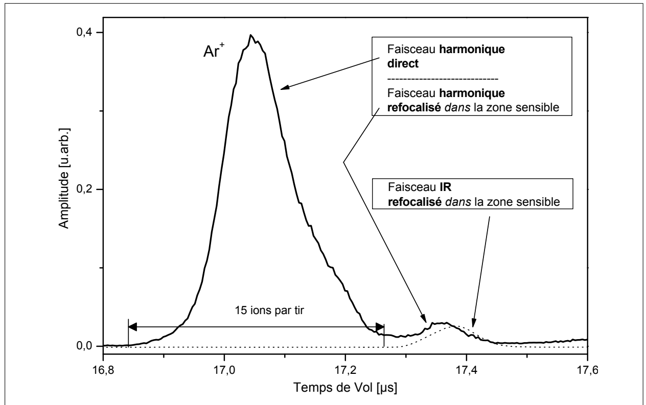
Fig. 2.12 : Temps de vol de \text{Ar}^+ . Signal d'ions dû au faisceau harmonique refocalisé dans la zone de détection ( z=0 \text{ mm} , P(\text{Ar})=1,2 \cdot 10^{-6} \text{ mbar} ) (trait plein). La pression dans la cellule remplie de xénon est P(\text{Xe})=8 \text{ mbar} . L'énergie laser incidente sur la cellule est de 3 mJ.
