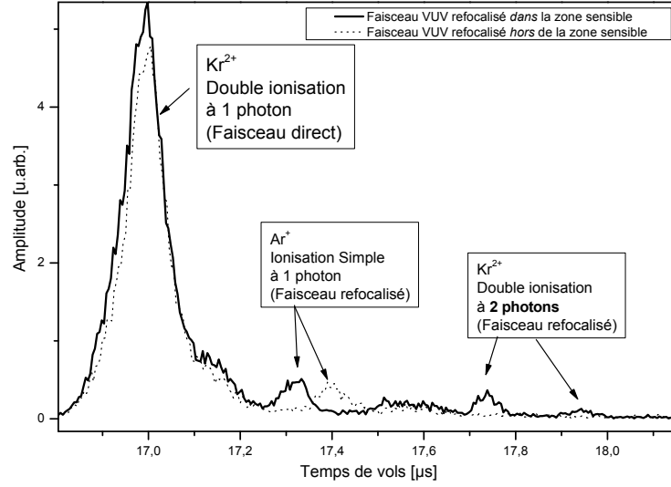
Fig. 2.18 : Temps de vol des ions \text{Kr}^{2+} et \text{Ar}^+ . Signal d'ions (trait plein) dû au faisceau harmonique refocalisé dans la zone sensible ( z=0 mm). Signal d'ions (trait pointillé) dû au faisceau harmonique refocalisé hors la zone sensible ( z=6 mm). La pression dans la zone sensible est de P(\text{Kr})=2.10^{-4} mbar. La pression dans la cellule de génération d'harmoniques remplie de xénon est P(\text{Xe})=14 mbar. Énergie incidente sur la cellule E=2.5 mJ.
