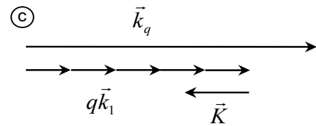
Fig. 1.10 : Distribution spatiale dans la région du foyer du vecteur d'onde laser \mathbf{k}_1 (1) et du vecteur d'onde \mathbf{K} associé la phase atomique (2) d'après [Balcou et al. 97].
