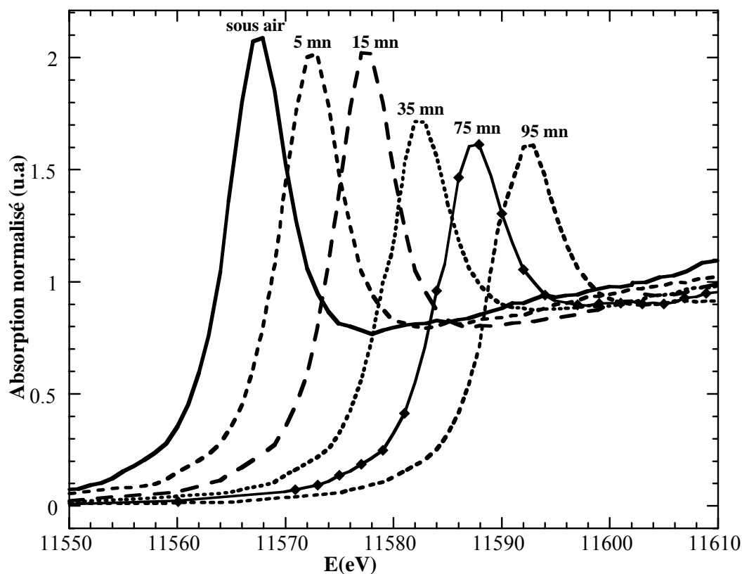
Figure V.18 : Evolution de la hauteur de la raie blanche en fonction du temps, en présence de N_2 + CO à 200^\circ C (cas SnO_2 + 3\%Pt ). Celle de la raie blanche sous air est indiquée à titre de comparaison. Un décalage en énergie est ajouté (par rapport à la raie blanche sous air) entre les différents spectres pour une meilleure lecture.
