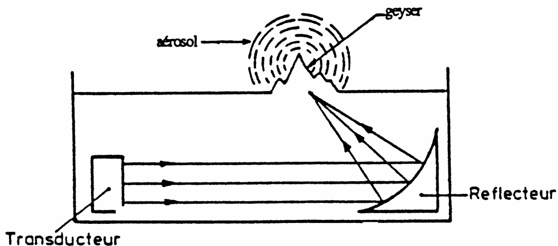
Figure II.1 : Principe de la pulvérisation ultrasonore.
