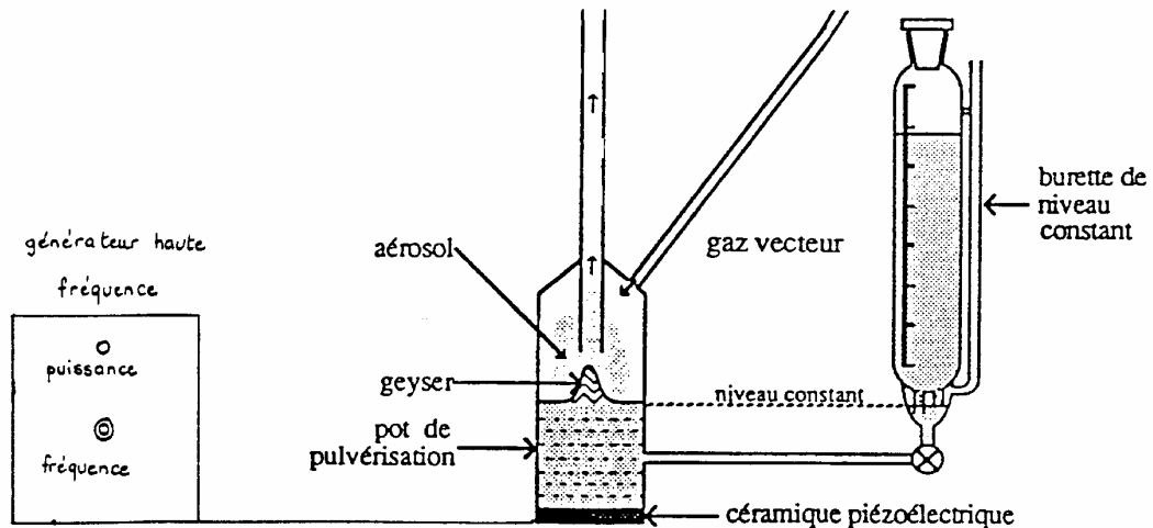
Figure.II-7 : Système de pulvérisation ultra-sonore.
