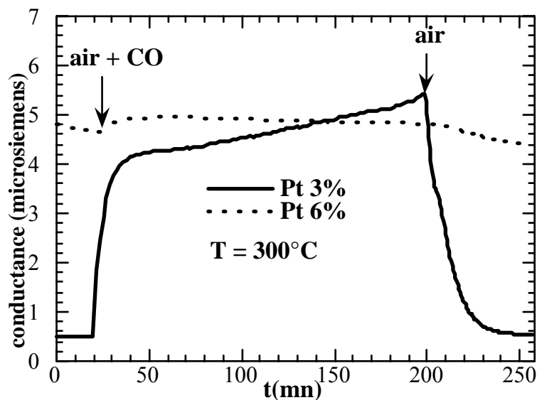
Figure IV.18 : Mesure électrique en cinétique, d'une couche de SnO 2 + 3 ou 6 % de Pt, sous air + CO (T = 300°C).
