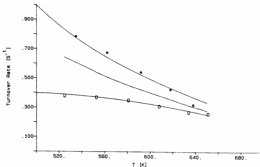
Figure I.18 :Vitesse d'oxydation de CO sur Pd déposé sur \text{Al}_2\text{O}_3 en fonction de la température : (o) D = 3.7 \text{ nm} , n = 1,3 \times 10^{12} \text{ cm}^{-2} et (*) D = 3,9 \text{ nm} , n = 1,6 \times 10^{10} \text{ cm}^{-2} , n : densité des particules, D : taille des particules. D'après [RUM88].
