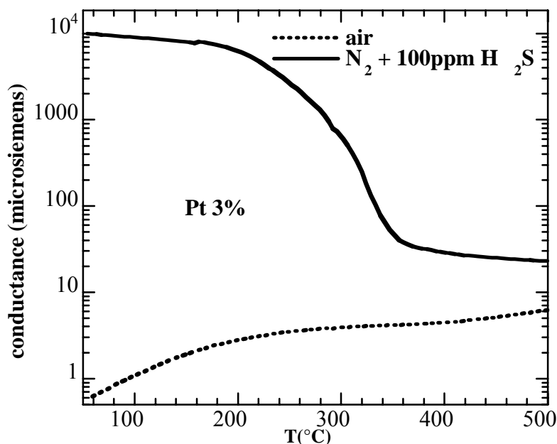
Figure VI.1 : Réponse électrique d'une couche de \text{SnO}_2 dopé Pt (3%) sous \text{N}_2 + 100\text{ppm H}_2\text{S} .
