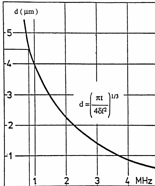
Figure II.2 : Variation du diamètre moyen des gouttelettes d'aérosol en fonction de la fréquence du signal ultrasonore au sein du liquide (eau).
