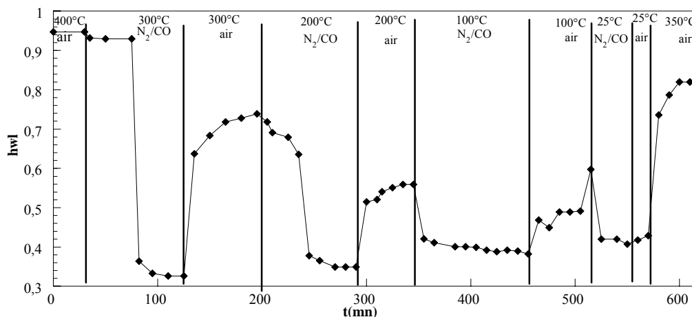
Figure V.16 : Evolution de la hauteur de la raie blanche (hwl) en fonction du gaz, de la température et du temps. Cas de SnO 2 + 6 % Pt.
