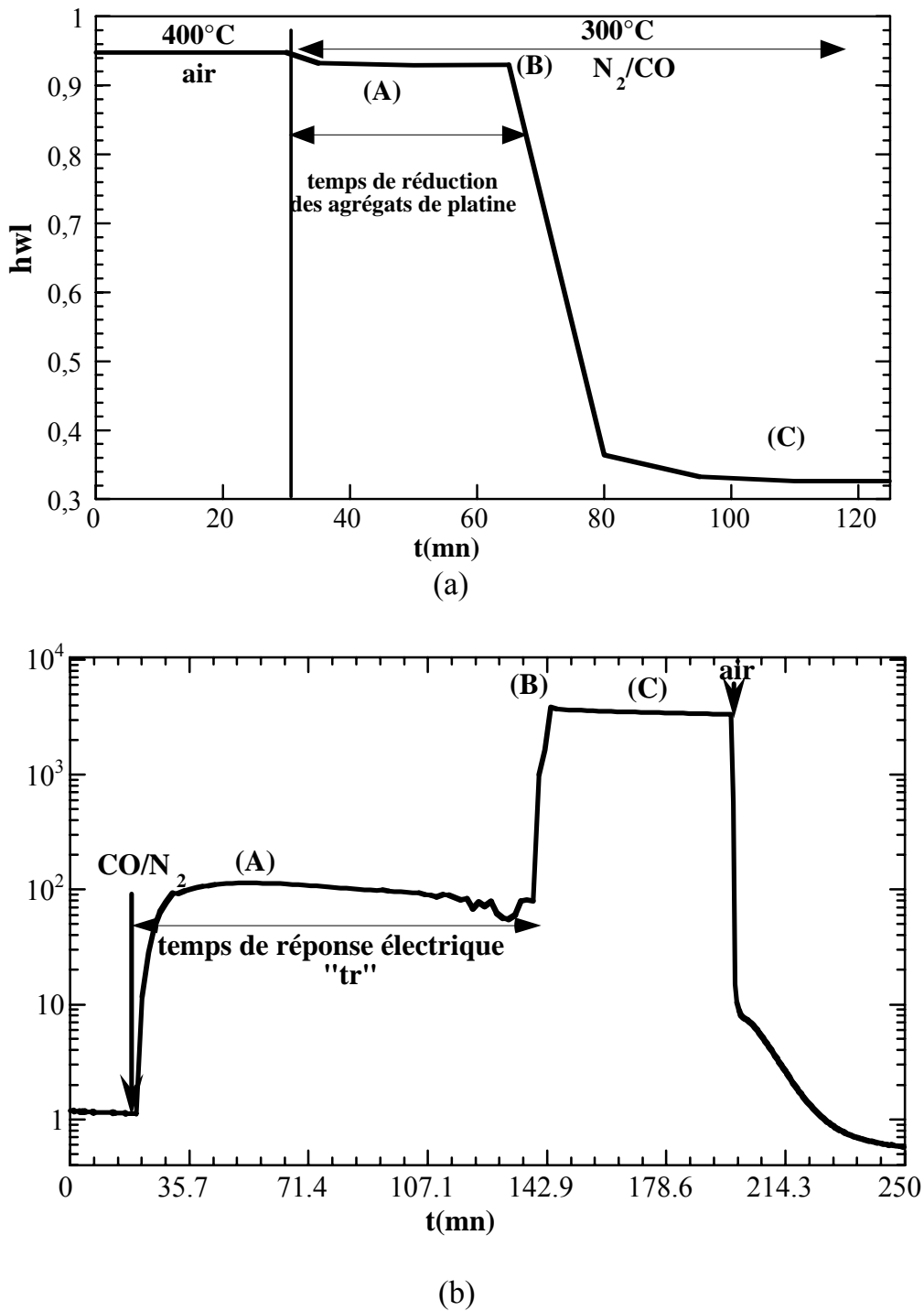
Figure V.17 : Les différentes étapes de réduction des agrégats de platine à 300°C (a) et l'évolution de la conductance électrique en présence de N 2 +CO (b) .
