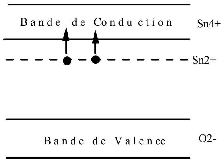
Figure I.2 : Diagramme énergétique de SnO 2 . D'après [PIJ86].
