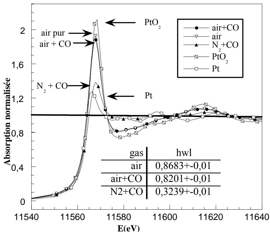
Figure V.15 : Evolution de la hauteur de la raie blanche (hwl) au seuil L_{III} du platine ( \text{SnO}_2 + 6\% \text{ Pt} ) en fonction de la nature du gaz : air pur, air + CO (300 ppm) et \text{N}_2 + \text{CO} (900 ppm).
