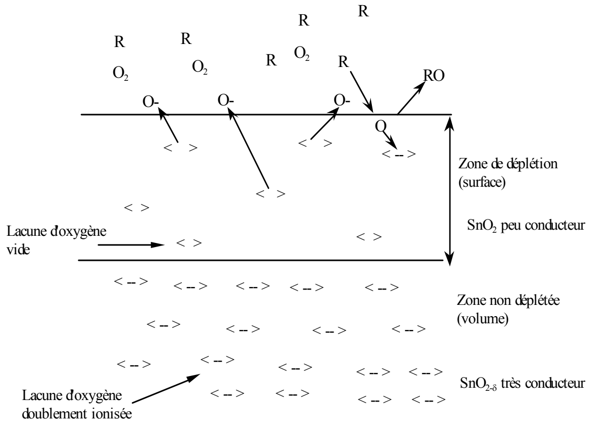
Figure I.4 : Formation d'une zone de déplétion à la surface de SnO 2 .
