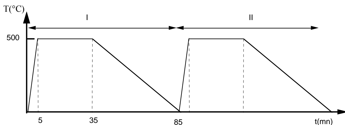
Figure IV.3 : Cycle thermique pour les mesures G(T) .
