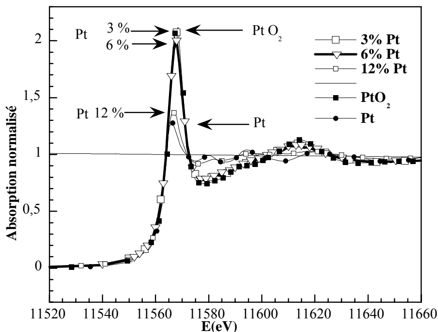
Figure V.12 : Evolution de l'état d'oxydation du platine sous air en fonction de sa concentration dans la solution source (le trait horizontal représente l'absorption atomique après seuil).
