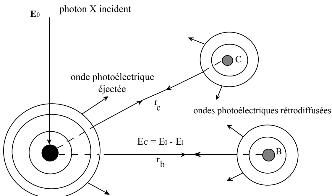
Figure V.4: Représentation de l'interférence entre l'onde photoélectrique émise par l'atome centrale (A) et les ondes rétrodiffusées par les atomes proches
