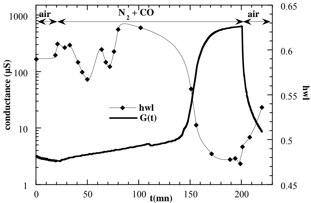
Figure V.31 : Cinétique de la réaction de réduction des agrégats de platine et évolution de la conductance électrique. Cas de \text{SnO}_2 + 6\% \text{ Pt}
