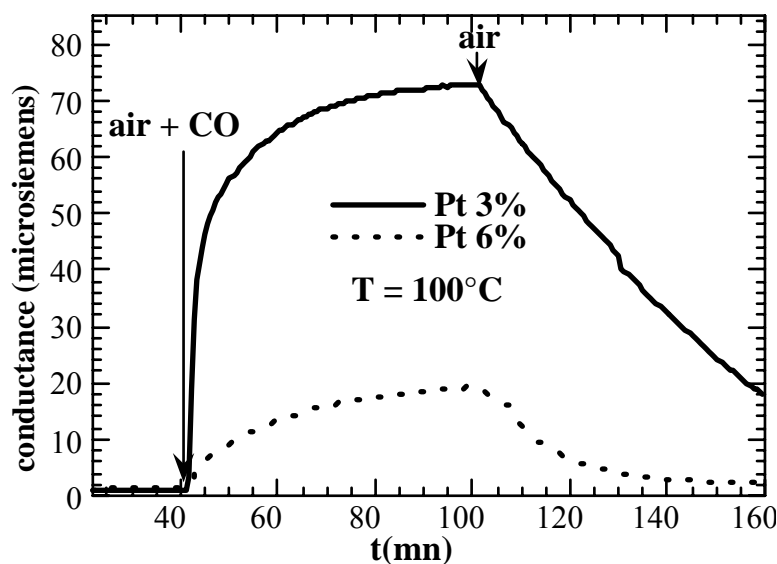
Figure IV.19 : Mesure électrique en cinétique, d'une couche de SnO 2 + 3 ou 6 % de Pt, sous air + CO (T = 100°C).
