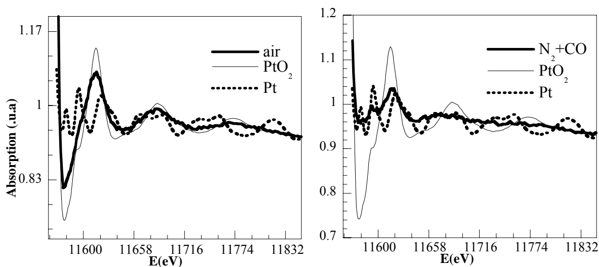
Figure V.14 : Oscillations EXAFS en fonction de la nature de l'atmosphère environnante (cas SnO 2 + 6 % Pt) et comparaison avec les spectres de références (de Pt et PtO 2 ). T = 350°C.
