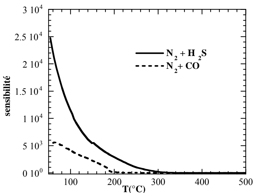
Figure VI.2 : Evolution de la sensibilité mesuré sous \text{H}_2\text{S} et sous \text{CO} en fonction de la température.
