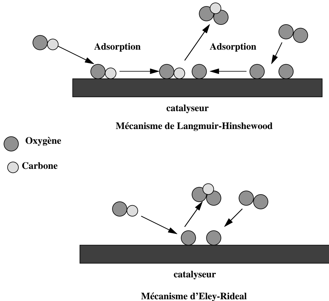
Figure I.15 : Mécanisme d'interaction à la surface d'un catalyseur, entre le monoxyde de carbone et l'oxygène.
